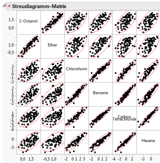
Streudiagramm-Matrix
