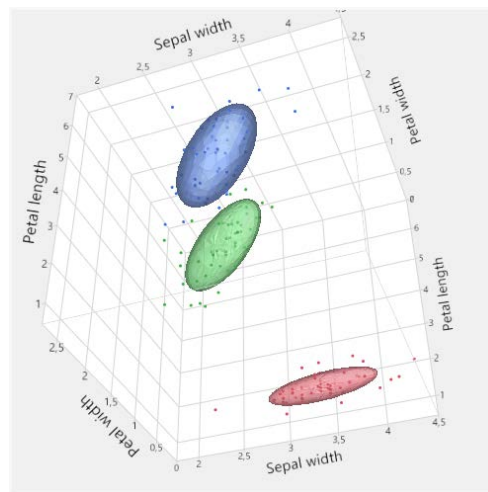
Dreidimensionales Streudiagramm
