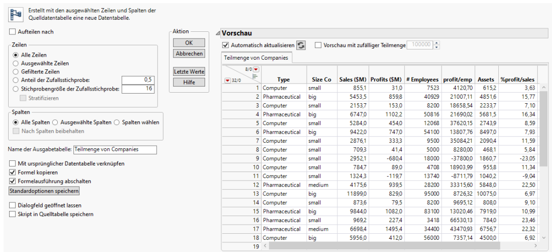
Abbildung 3.26 Teilmengenfenster
