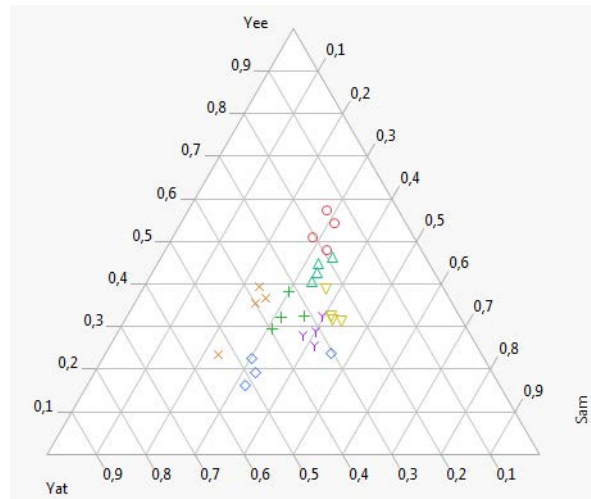
Ternäres Diagramm
