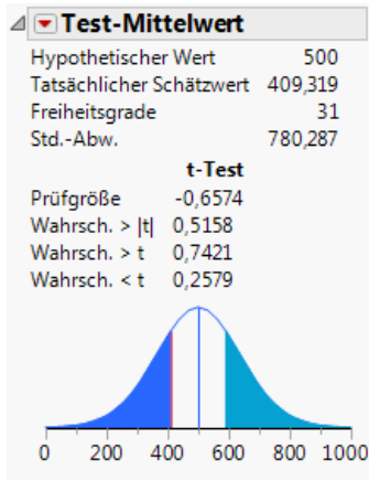
Abbildung 2.8 Mittelwerttest
