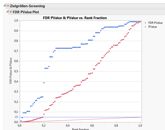
FDR PWert-Plot
