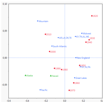
Multiple Korrespondenzanalyse
