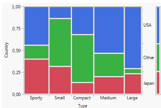
Mosaikdiagramm
