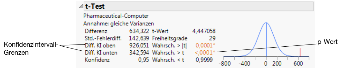
Abbildung 5.18 t -Test-Ergebnisse
