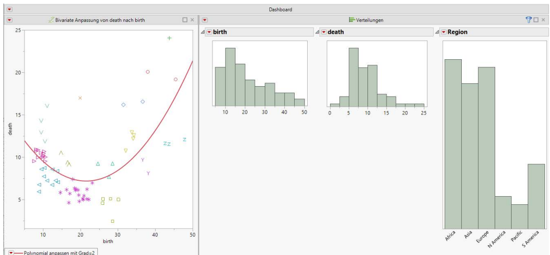
Abbildung 7.19 Verbundene Fenster
