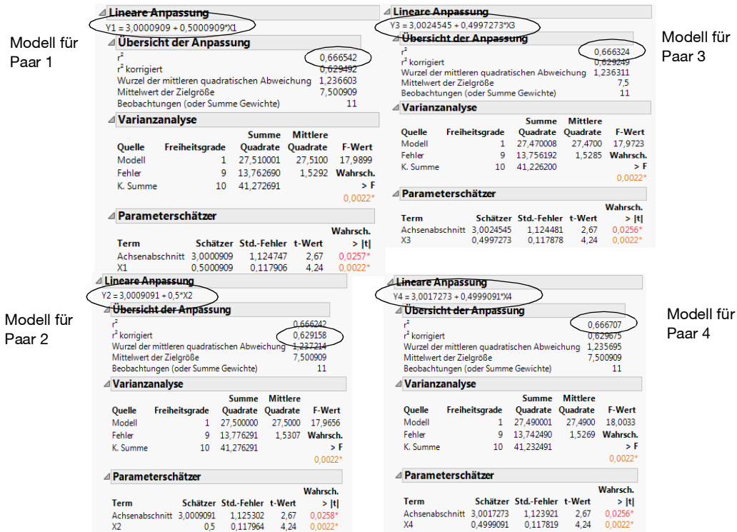
Abbildung 5.2 Vier Modelle
