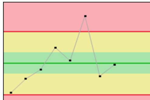
Xquer-Regelkarte
