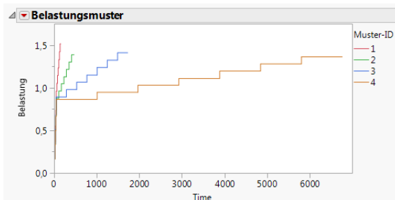
Belastungsmusterdiagramm
