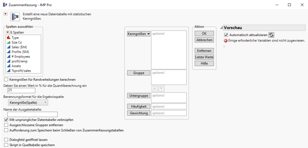
Abbildung 3.18 Ausgefülltes Zusammenfassungsfenster
