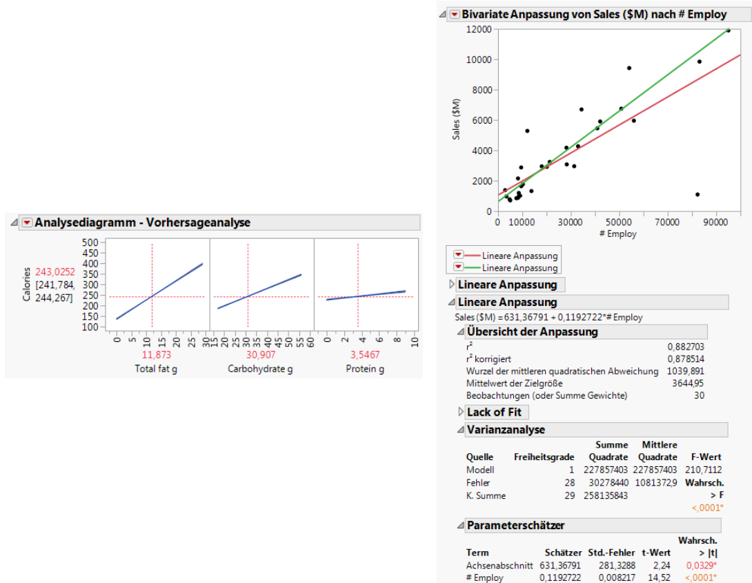
Abbildung 5.1 Analysebeispiele
