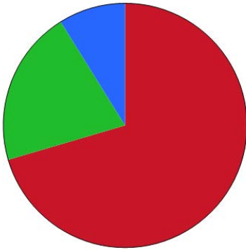
Tortendiagramm
