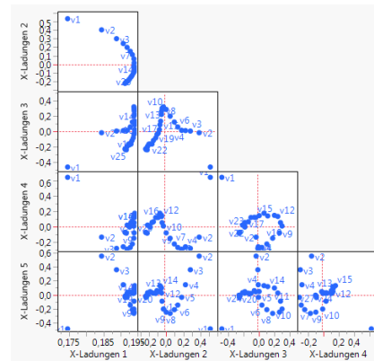
Ladungsdiagramme
