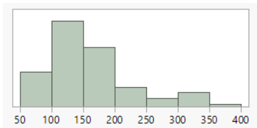
Histogramm
