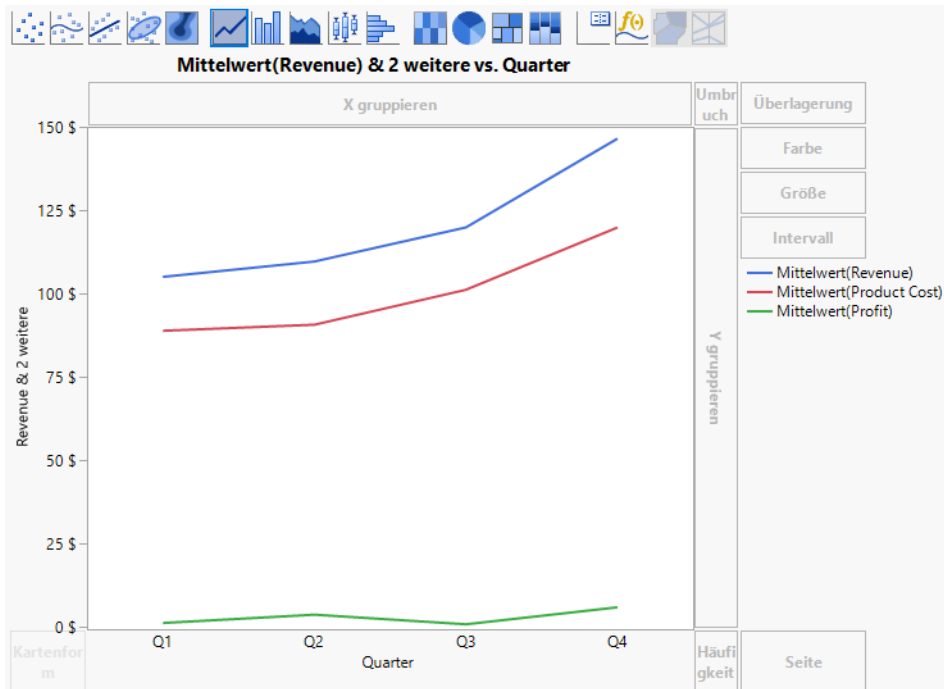
Abbildung 4.24 Linien-Plot
