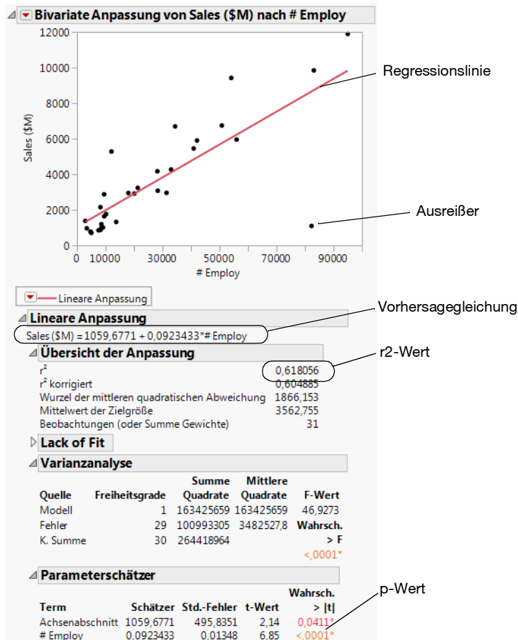
Abbildung 5.13 Regressionslinie
