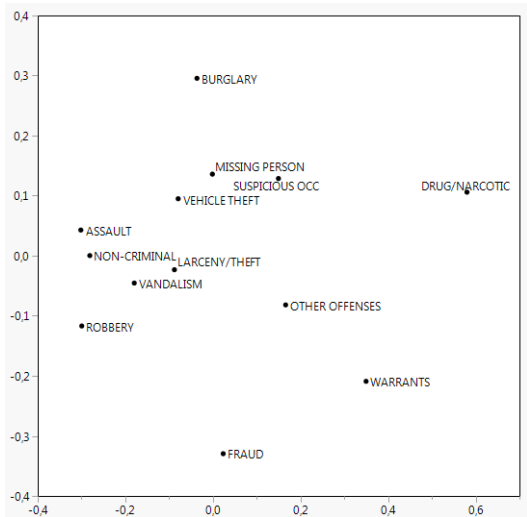
Multidimensionale Skalierung
