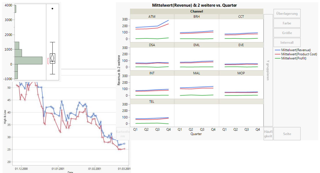
Abbildung 2.1 Beispiele von JMP-Berichten
