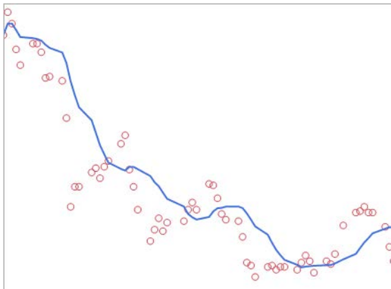
Glätten
