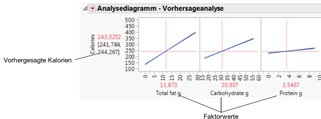
Abbildung 5.30 Analysediagramm - Vorhersageanalyse
