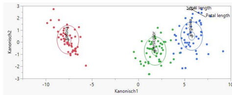
Kanonisches Diagramm
