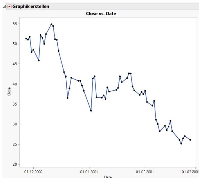
Abbildung 4.34 Verbundene Punkte
