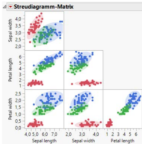
Streudiagramm-Matrix
