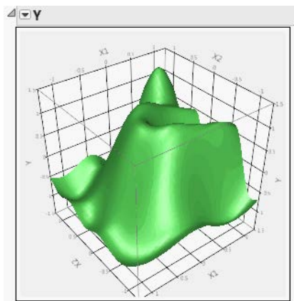
Wirkungsflächenanalyse
