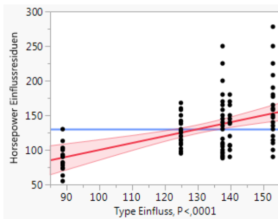
Einflussdiagramm
