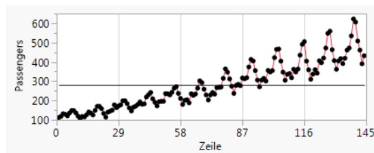
Zeitreihe
