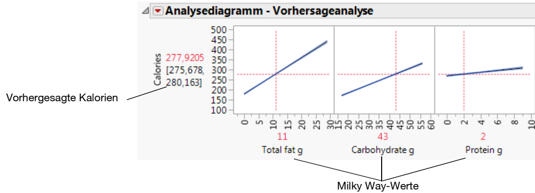
Abbildung 5.31 Faktorwerte für Milky Way
