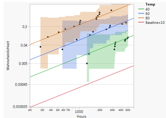
Nichtparametrische Überlagerung
