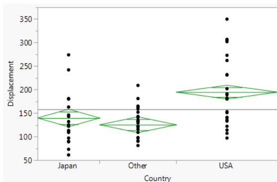
Einfaktoriell
