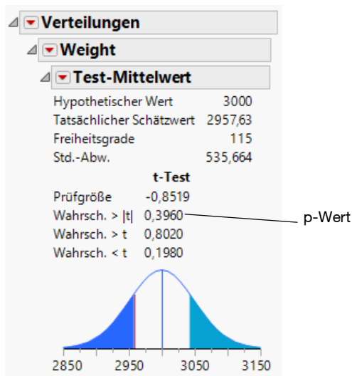
Abbildung 5.8 Testen der Mittelweltergebnisse
