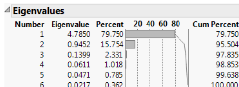
Figure 4.5 Eigenvalues
