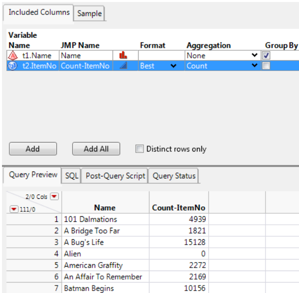
Figure 3.38 Grouped Columns
