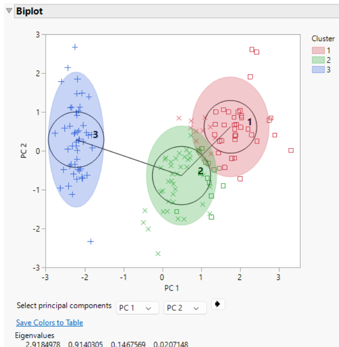
Figure 14.12 SOM Biplot
