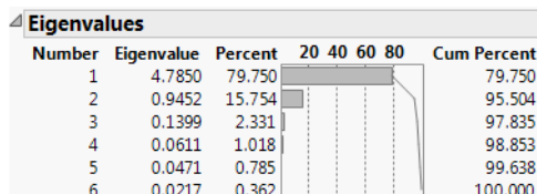
Figure 4.5 Eigenvalues
