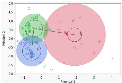
Mapa autorganizado
