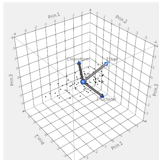
Componentes principales
