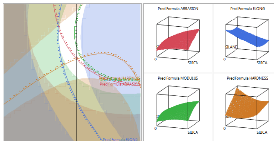
Perfilador de contorno
