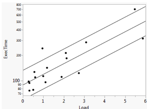
Cuantiles de supervivencia
