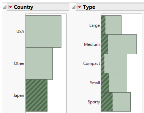
Figura 5.10 Automóviles japoneses
