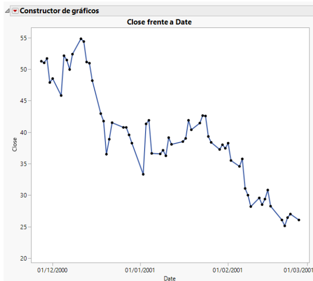
Figura 4.34 Puntos unidos
