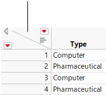
Figura 3.9 Deseleccionar columnas
