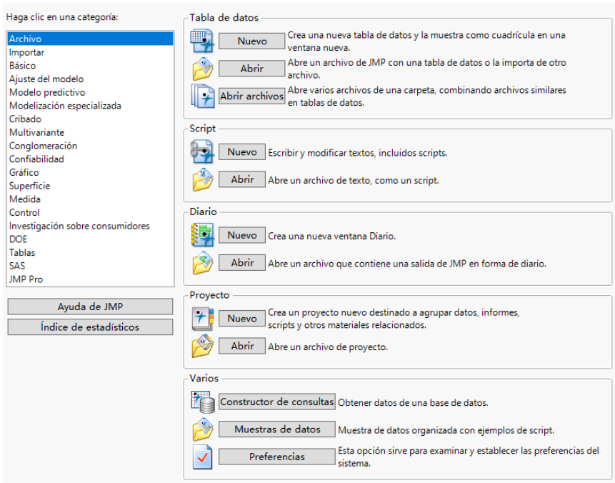
Figura 2.2 JMP Starter
