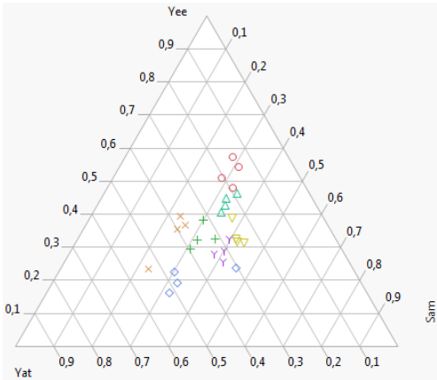
Gráfico ternario Gráficos > Gráfico ternario
