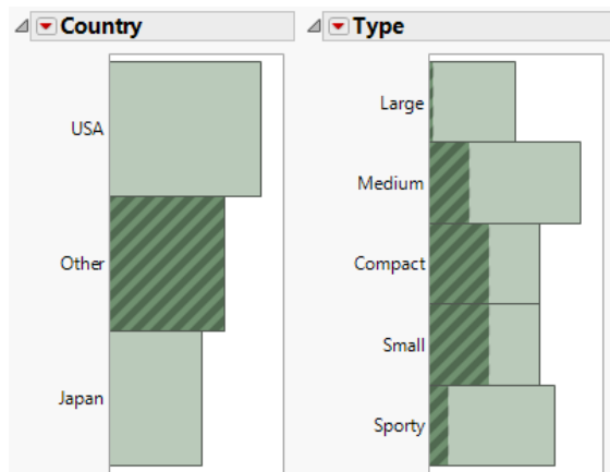
Figura 5.11 Otros automóviles
