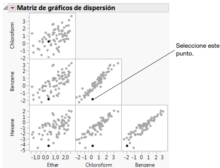
Figura 4.17 Puntos seleccionados
