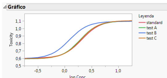
Ajuste no lineal
