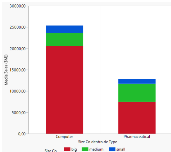
Gráfico de barras apilado
