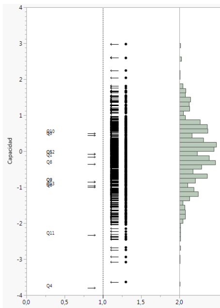
Gráfico dual
