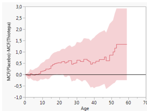
Gráfico de la MCF
