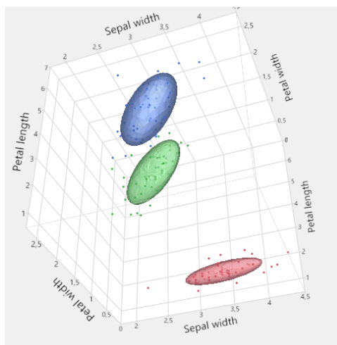
Gráfico de dispersión tridimensional
