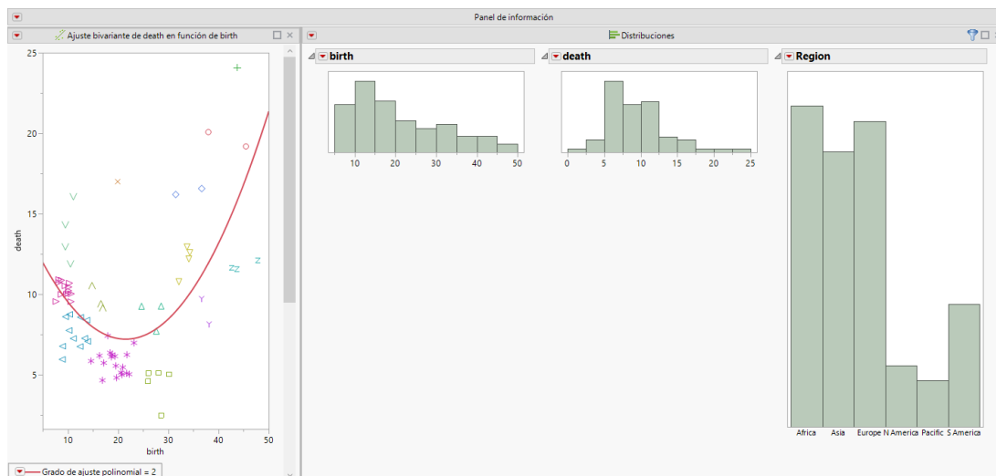
Figura 7.19 Ventanas combinadas
