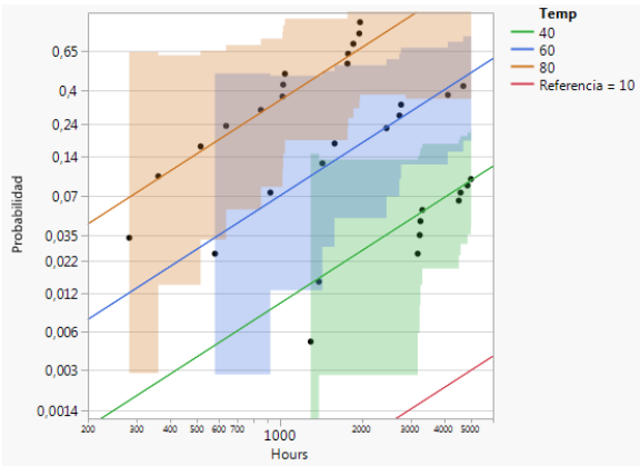
Superposición no paramétrica Análisis > Confiabilidad y supervivencia > Ajustar vida por X
