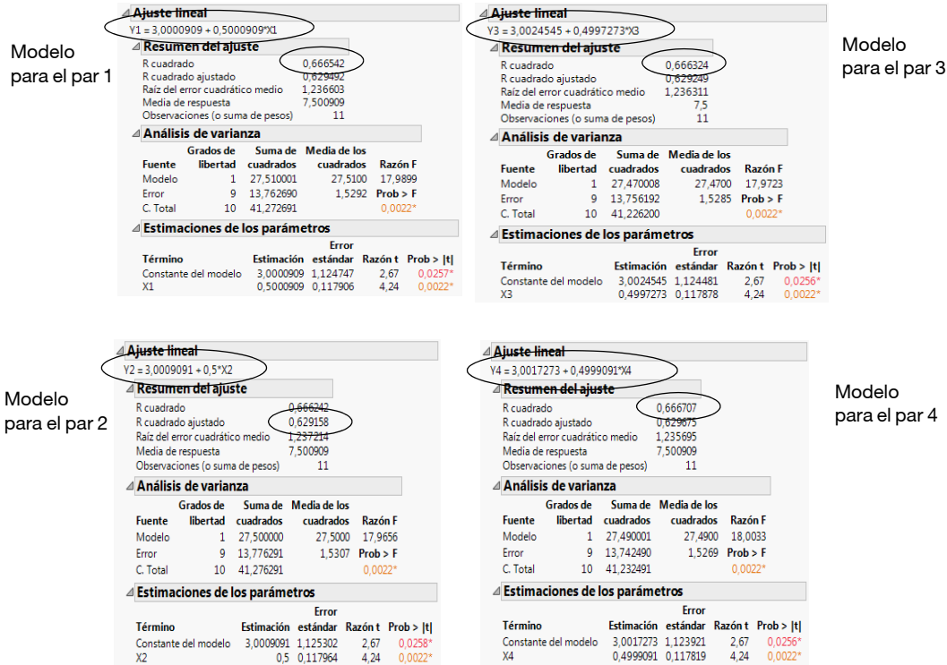
Figura 5.2 Cuatro modelos
