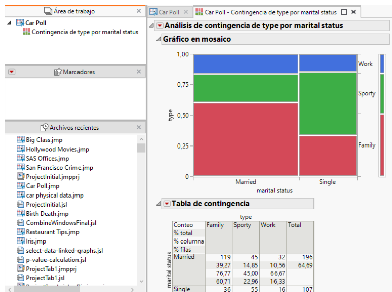
Figura 7.3 Proyecto inicial
