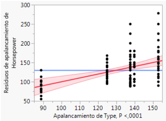
Gráfico de apalancamiento Análisis > Ajuste del modelo
