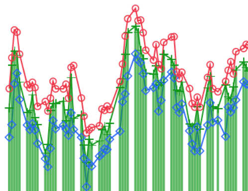
Gráfico de líneas y agujas
