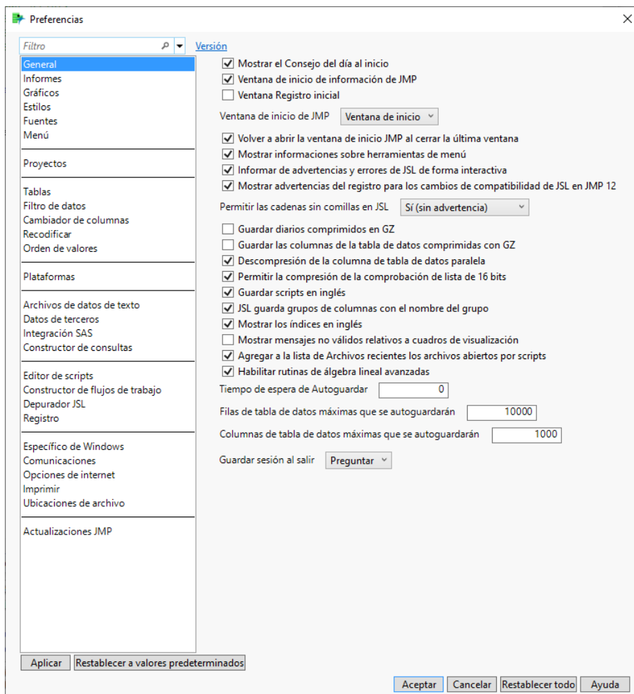
Figura 8.6 Ventana Preferencias
