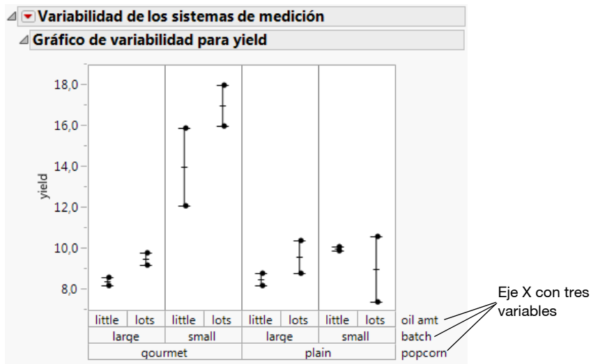
Figura 4.38 Ventana Resultados
