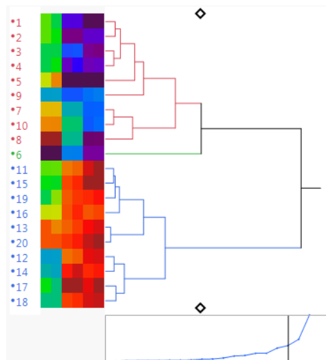
Dendrograma
