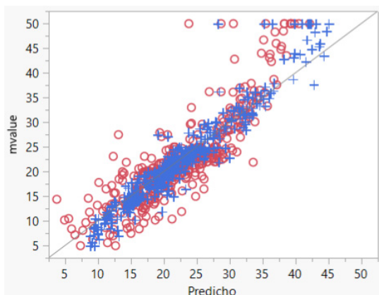
Observados frente a predichos
