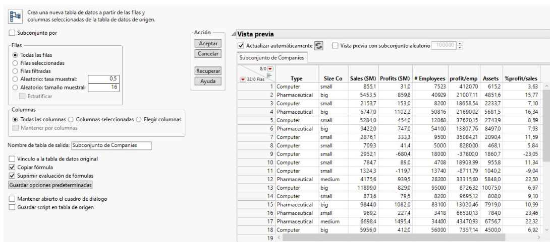
Figura 3.26 Ventana Subconjunto
