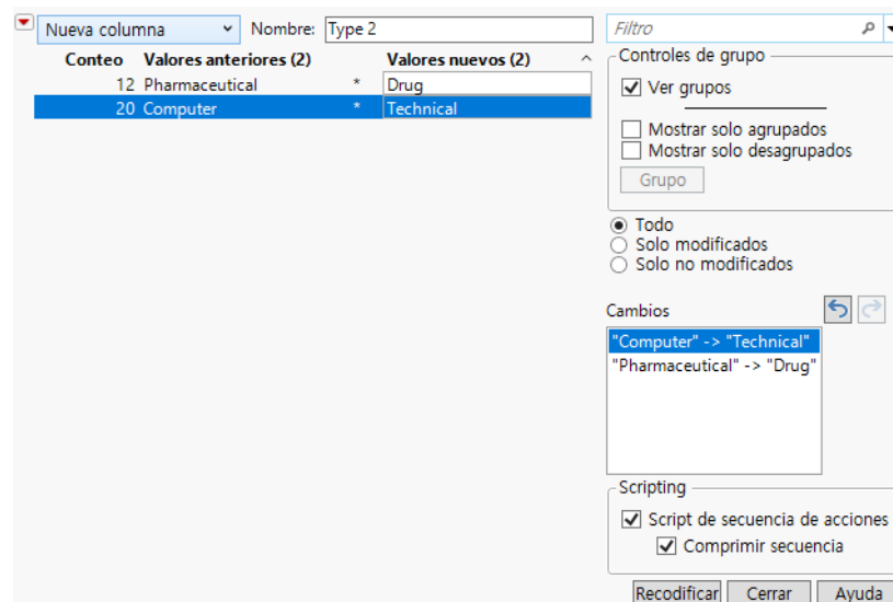
Figura 3.7 Ventana Recodificar
