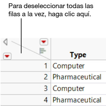
Figura 3.8 Deseleccionar filas
