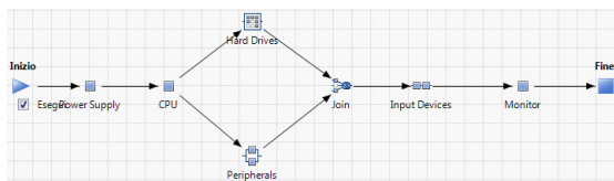
Diagramma a blocchi di affidabilità
