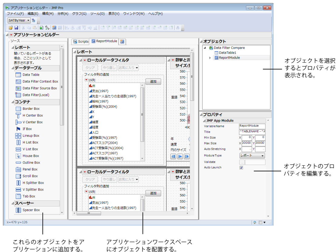
図16.4 「アプリケーションビルダー」 ウィンドウ
