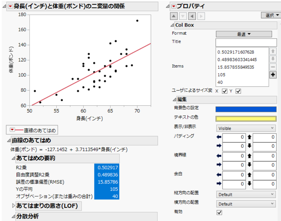
図11.5 プロットの「プロパティの表示」の例
