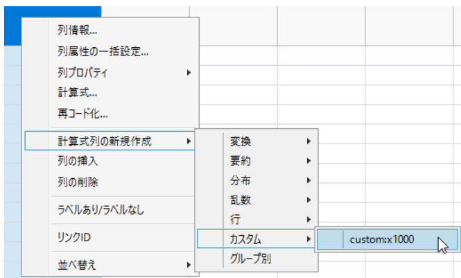
図9.10 データテーブル内のカスタム変換
