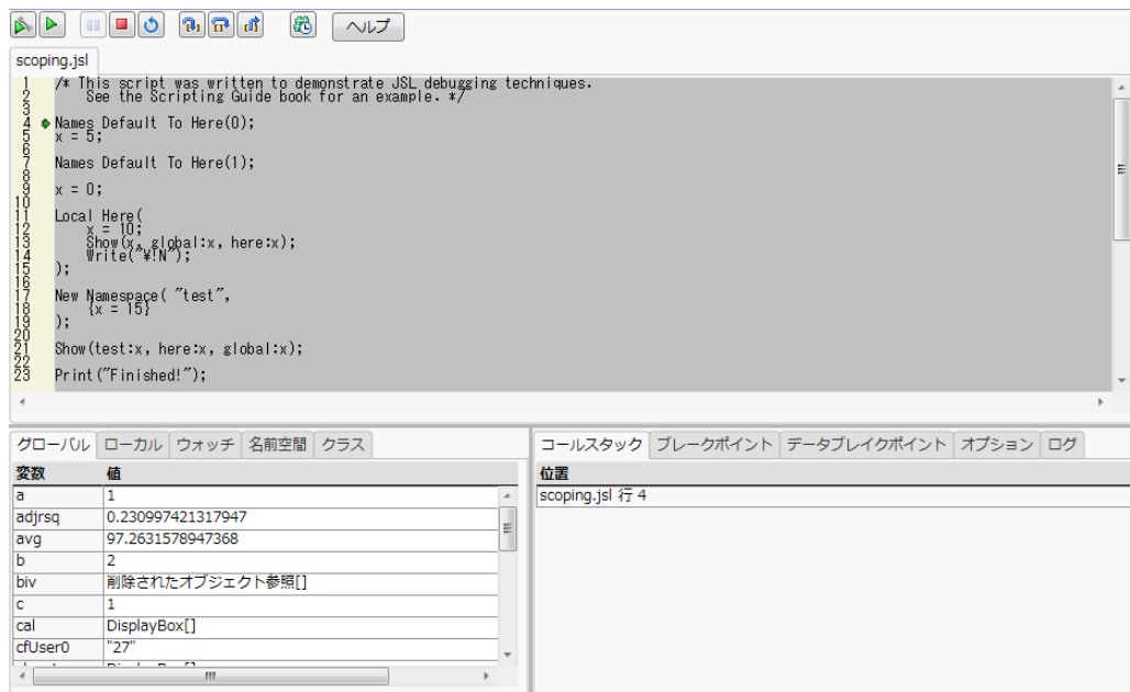
図4.10 デバッガウィンドウ
