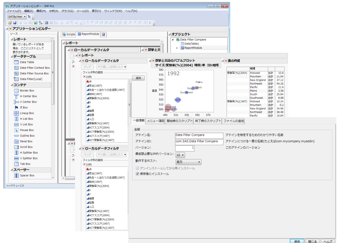
図16.1 アプリケーションビルダーでカスタマイズしたレポートを作成する
