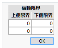
図11.9 信頼限界
