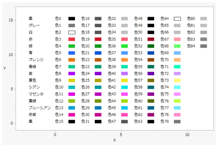
図9.14 JMPカラー
