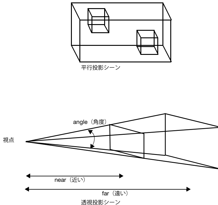
図13.5 投影の比較
