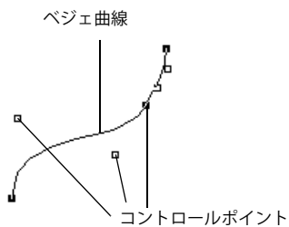
図13.19 ベジェ曲線
