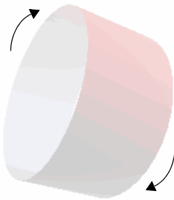
図13.18 霧
