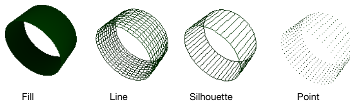
図13.13 描画の種類
