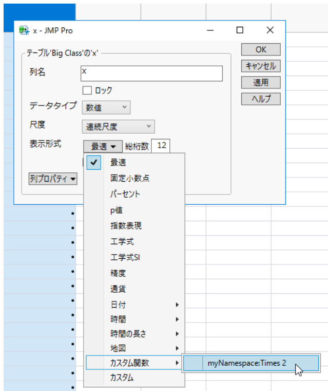
図9.11 [列情報] ウィンドウのカスタム表示形式
