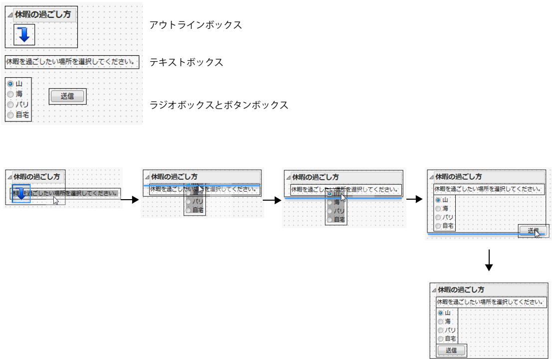
図16.5 コンテナ内にオブジェクトをドラッグする例
