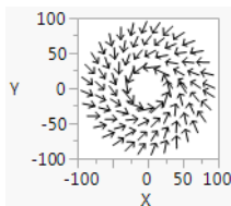
図12.11 矢印を描く
