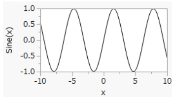
図12.32 正弦波
