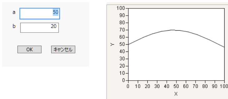
図8.2 起動と結果
