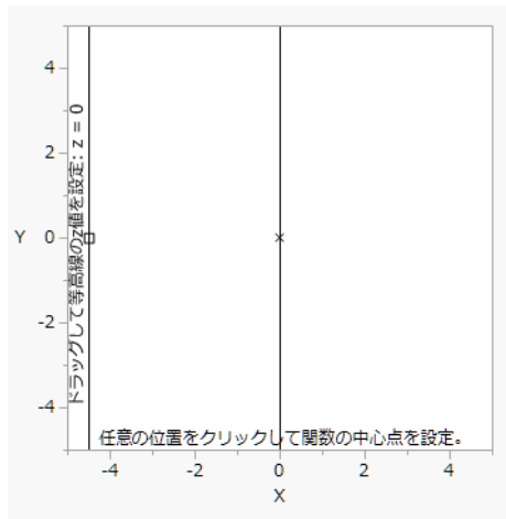
図12.27 Mousetrap() と Handle()
