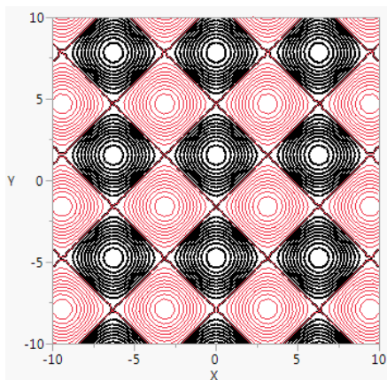
図12.36 卵ケース
