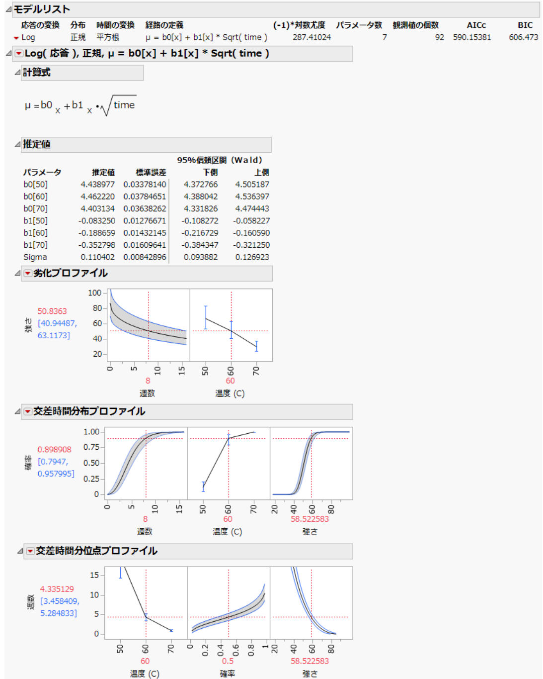
図9.4 基本的なモデルのレポート
