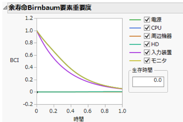
図12.22 余寿命 Birnbaum 要素重要度
