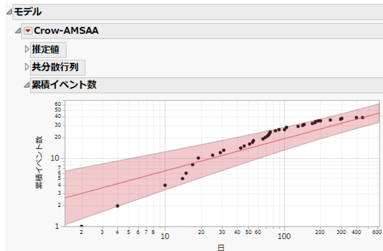
図11.11 「累積イベント数」グラフ
