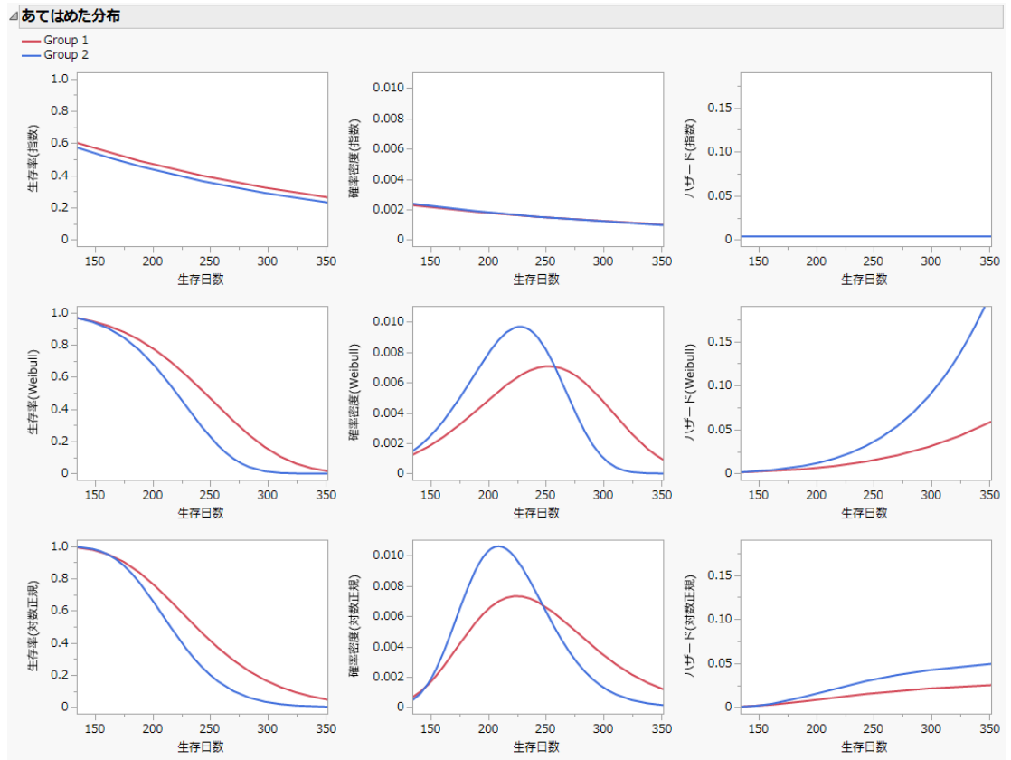
図14.7 3つの分布のグラフ
