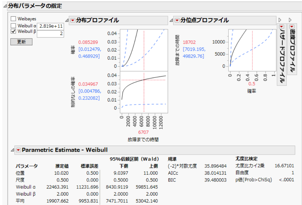
図3.26 Weibull \beta を指定したパラメータ指定モデル
