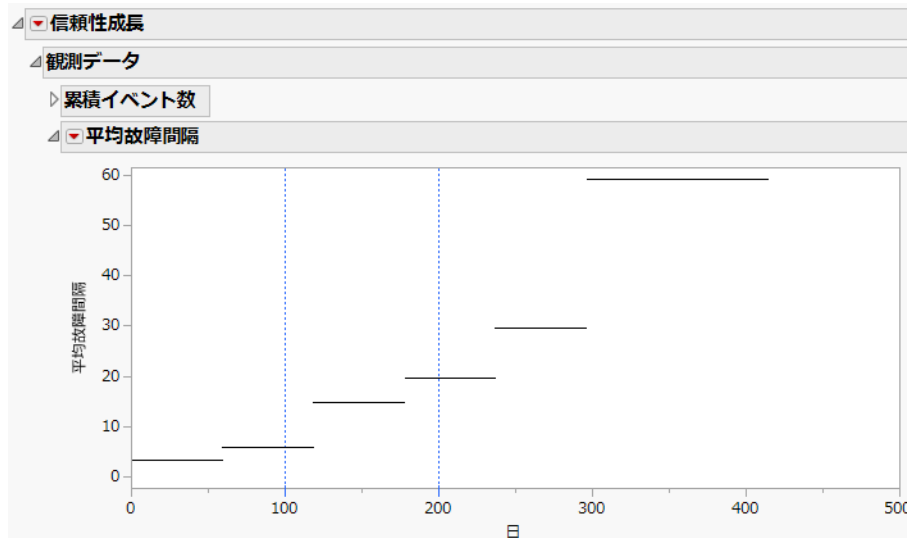
図11.3 「平均故障間隔」グラフ
