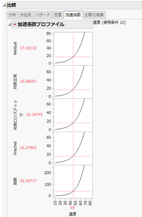
図4.10 加速係数プロファイル
