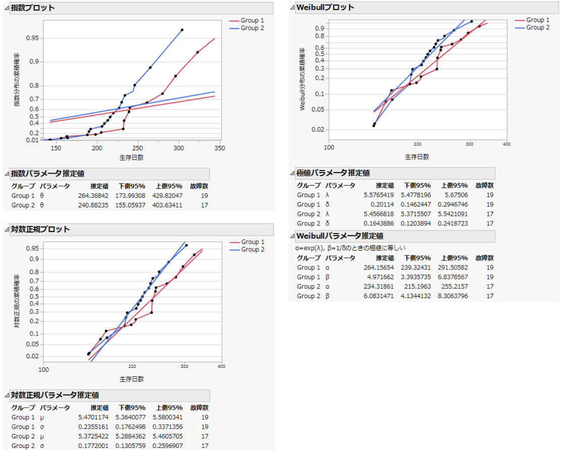
図14.5 指数プロット・Weibull・プロット・対数正規プロット
