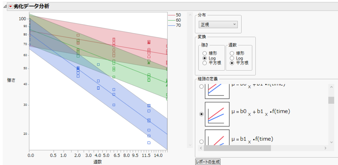
図9.11 破壊劣化のプロットとオプション
