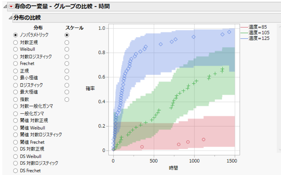
図3.16 分布の群間比較
