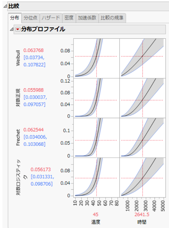
図4.8 分布プロファイル
