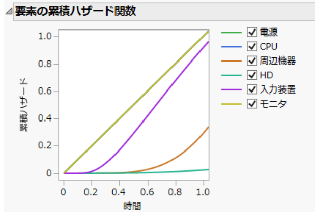
図12.28 要素の累積ハザード関数
