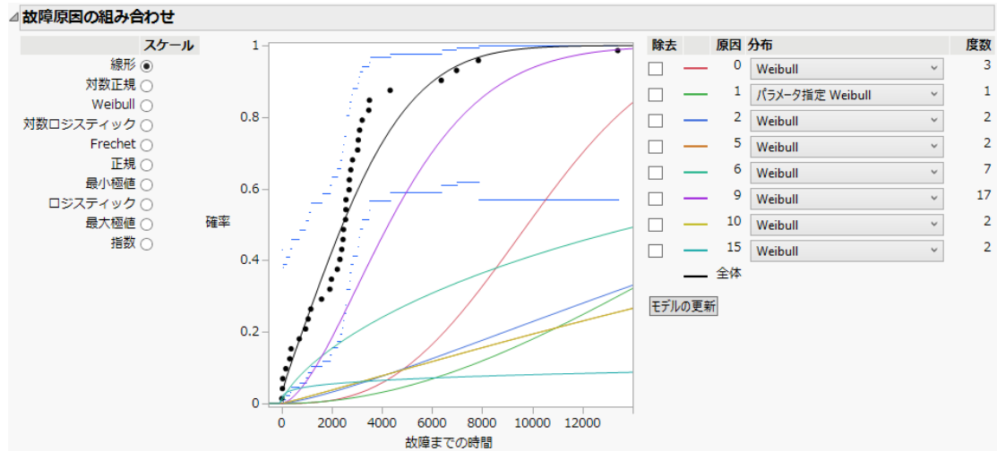
図 3.27 原因 1 が表示された更新モデル
