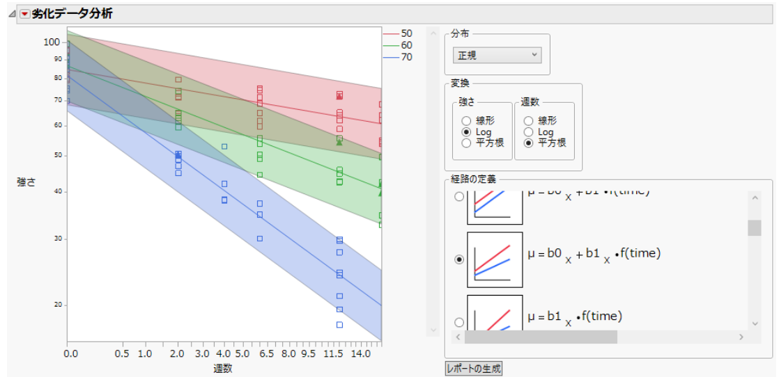
図9.3 モデルを表示したプロット
