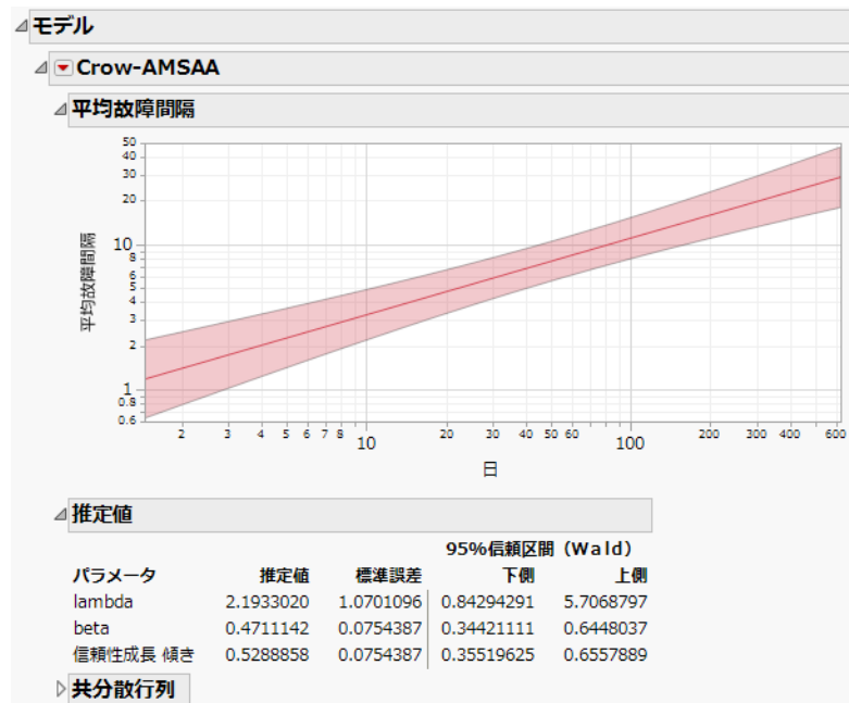
図11.9 「平均故障間隔」 グラフ
