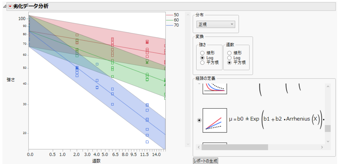
図9.5 Arrhenius変換を行ったモデルを表示したプロット
