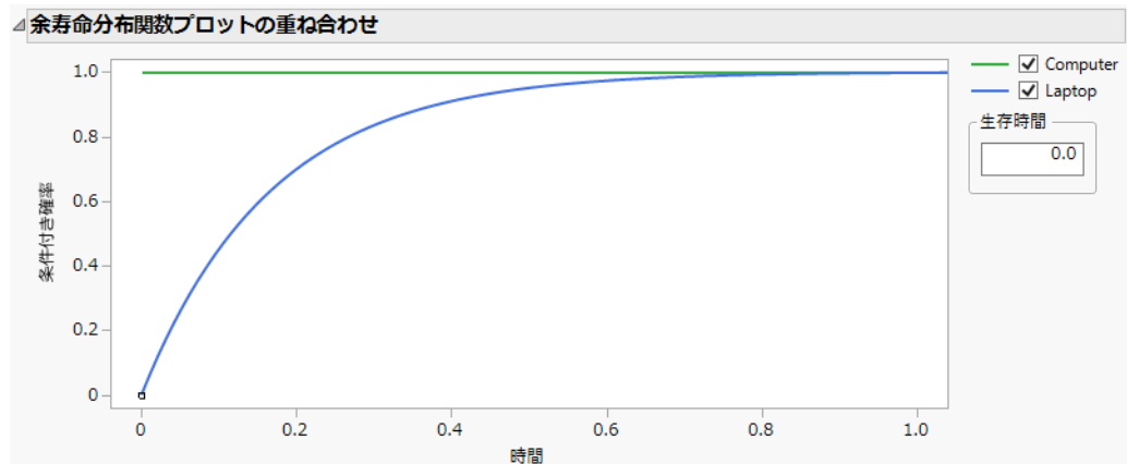
図 12.15 「余寿命分布関数プロットの重ね合わせ」の例
