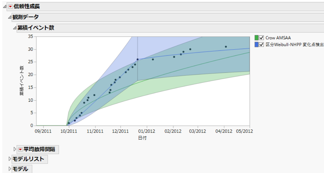
図 11.26 2つのモデルを割り当てた場合の「累積イベント数」グラフ
