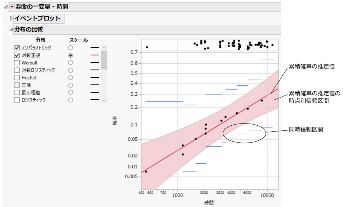
図3.2 確率プロット
