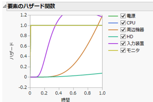
図12.27 要素のハザード関数
