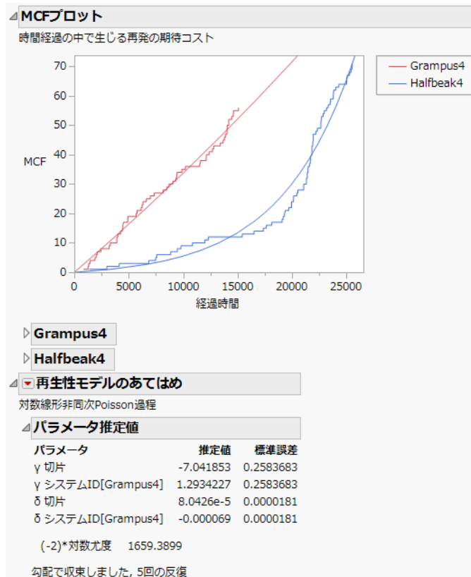
図6.11 「Diesel Ship Engines.jmp」にあてはめたモデル
