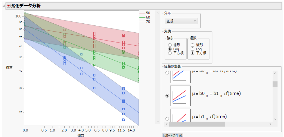
図9.1 「Adhesive Bond.jmp」の破壊劣化モデルの例
