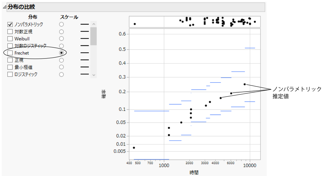
図3.14 Fréchetのスケールで表示したノンパラメトリック推定値
