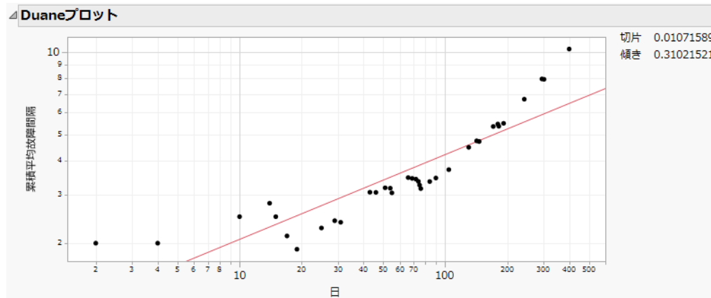
図11.4 Duane プロット
