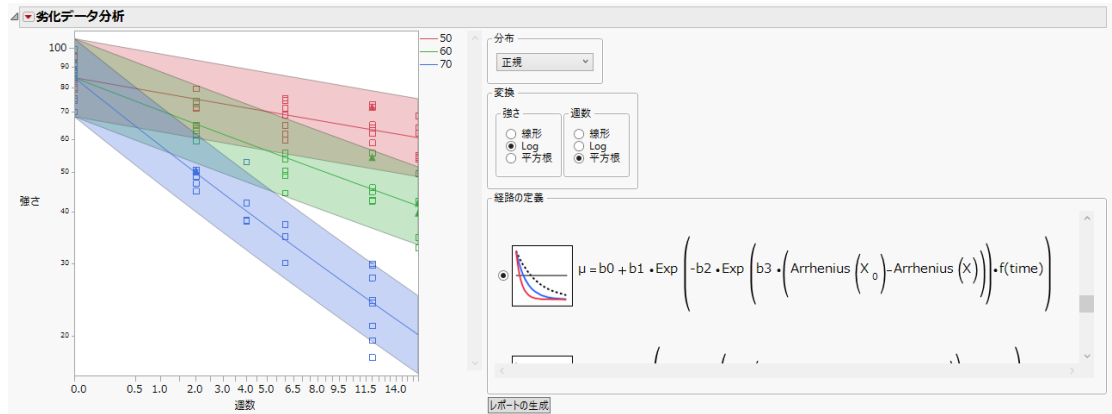
図9.13 1次反応速度 タイプ3の例
