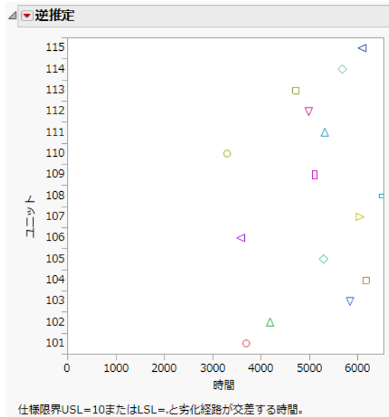
図7.14 「逆推定」プロット
