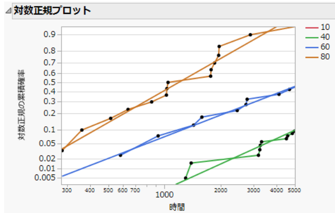
図15.8 対数正規プロット
