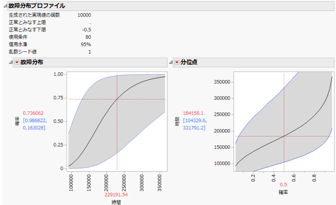
図8.16 故障分布プロファイル
