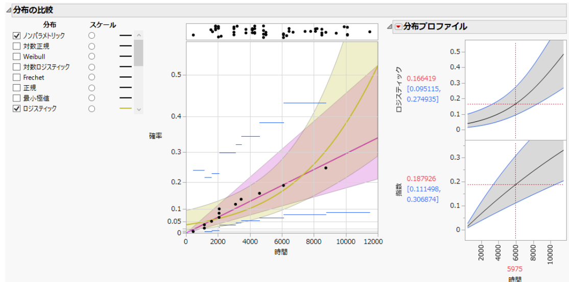
図3.1 分布のあてはめと比較
