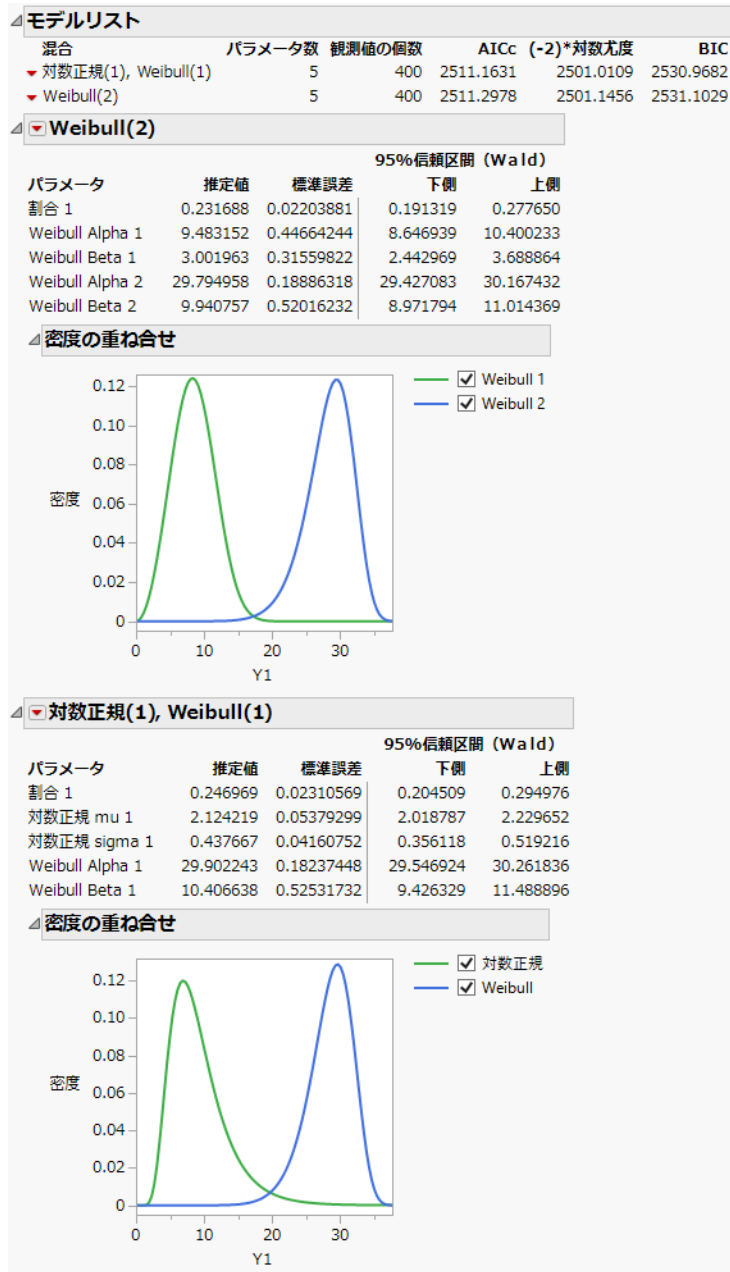
図3.21 「Lognormal(1), Weibull(1)」の混合分布のあてはめ
