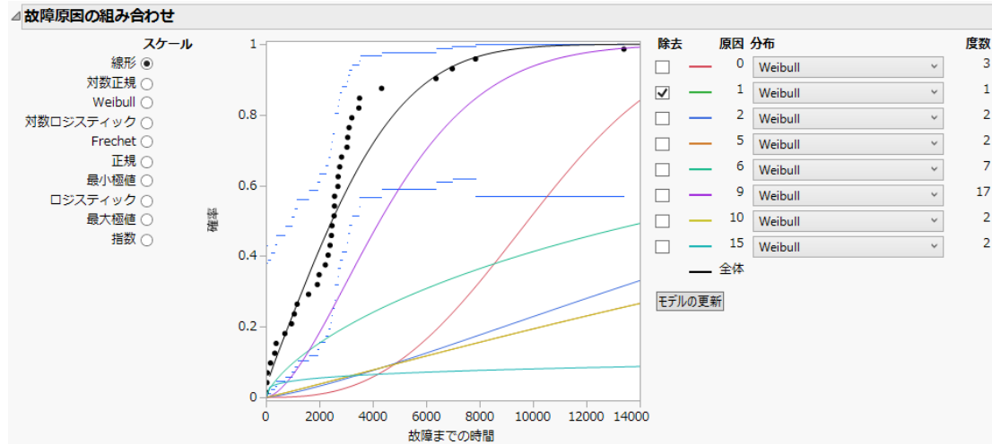
図 3.25 原因1を削除したパラメータ指定モデル
