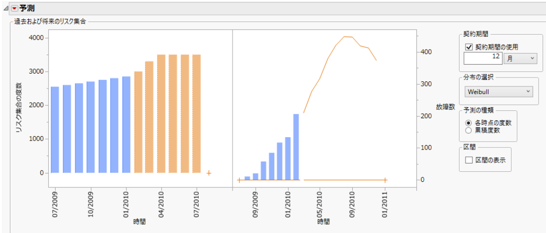
図10.6 将来の生産数と予測される故障数
