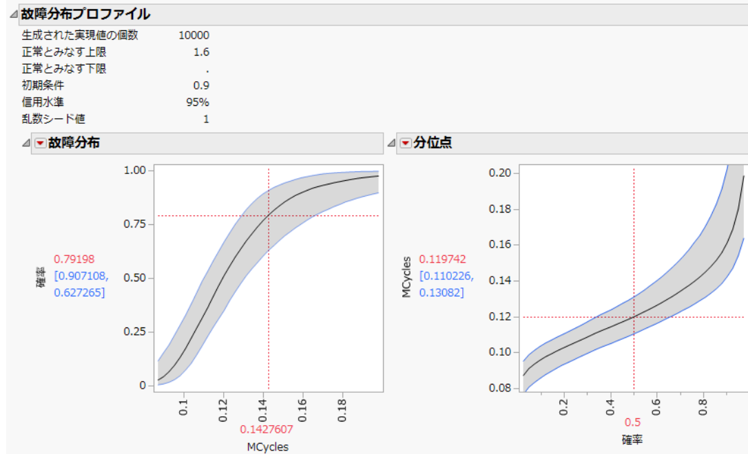
図8.6 故障分布プロファイル
