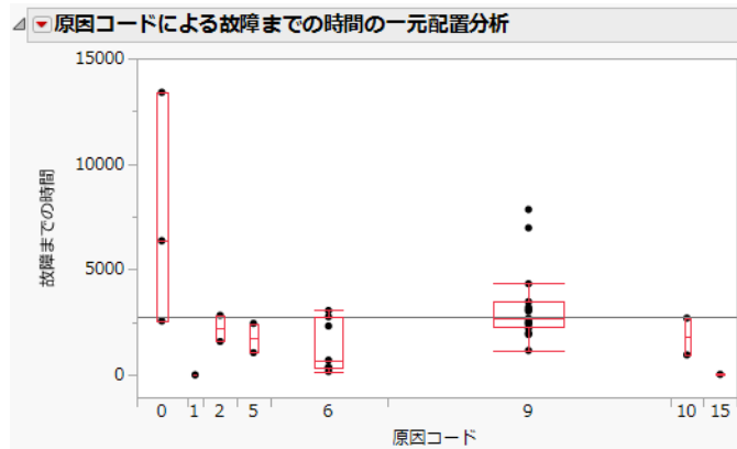
図14.12 「二変量の関係」で作成した「故障までの時間」と「原因コード」
