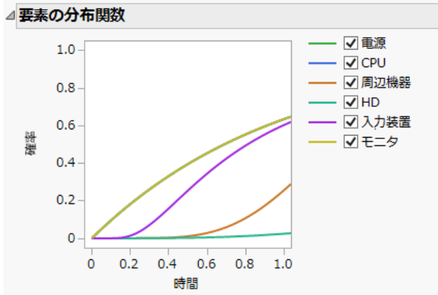
図12.24 要素の分布関数
