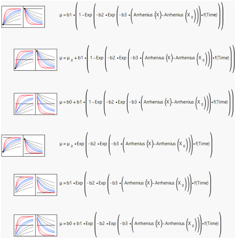
図8.10 1次反応速度モデル
