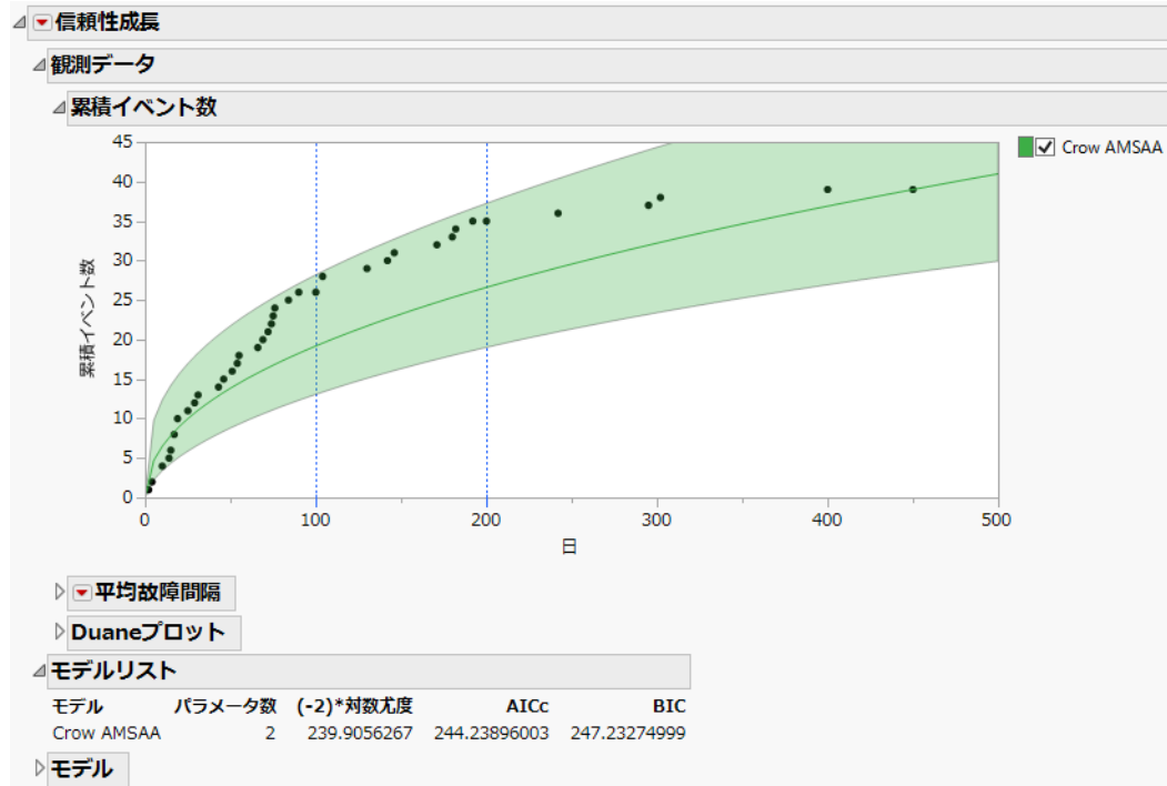
図 11.8 Crow AMSAA の「累積イベント数」グラフと「モデルリスト」レポート
