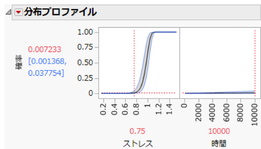
図5.4 指定された設定における指数分布の分布プロファイル
