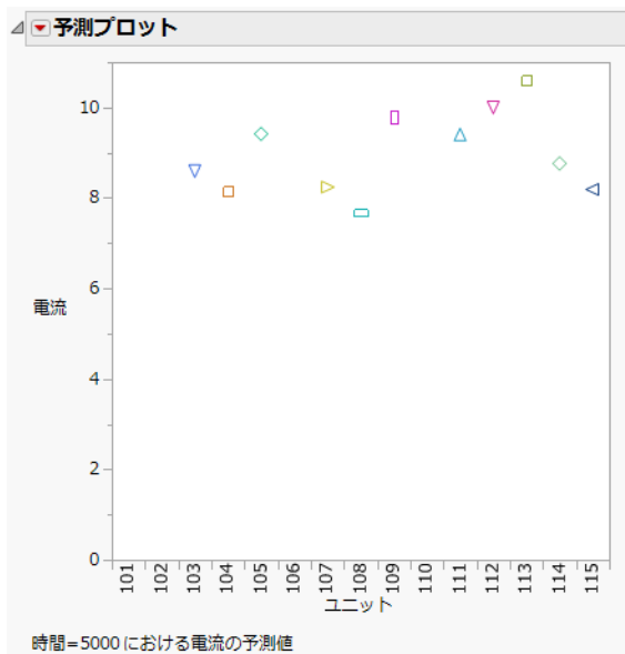
図7.16 予測グラフ
