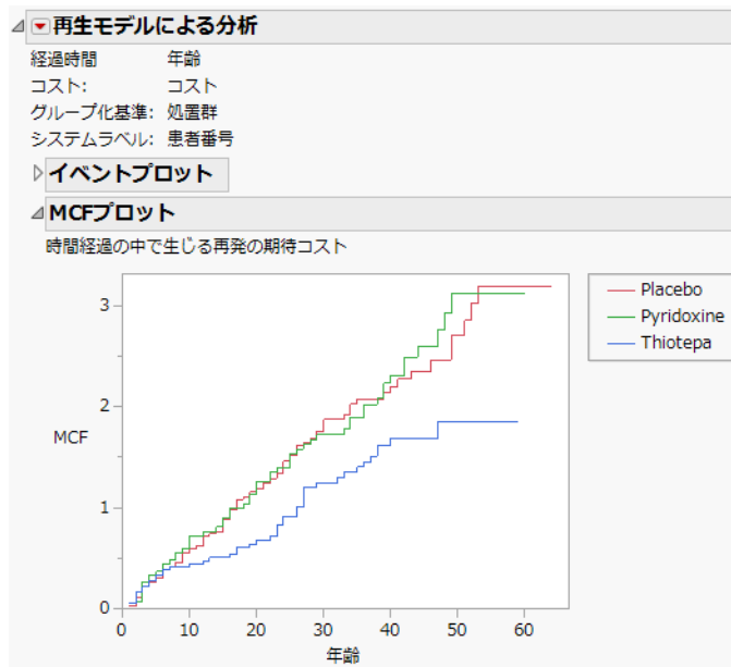
図6.7 「ぼうこう癌」のMCFプロット
