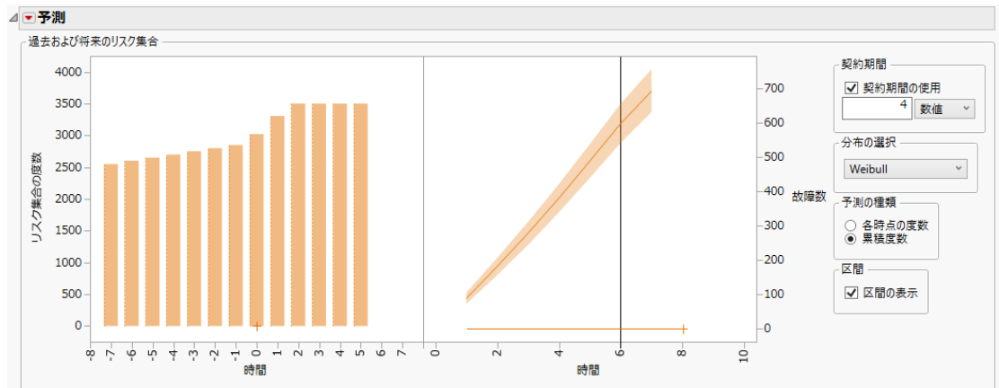
図10.16 予測結果
