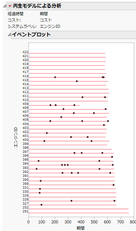
図6.2 バルブシートの交換を示したイベントプロット
