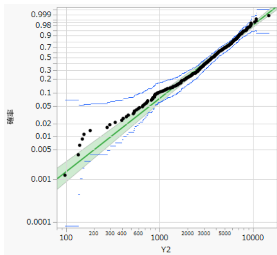
図3.23 Weibull 分布のあてはめ
