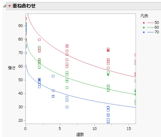
図7.22 あてはめたモデルのプロット
