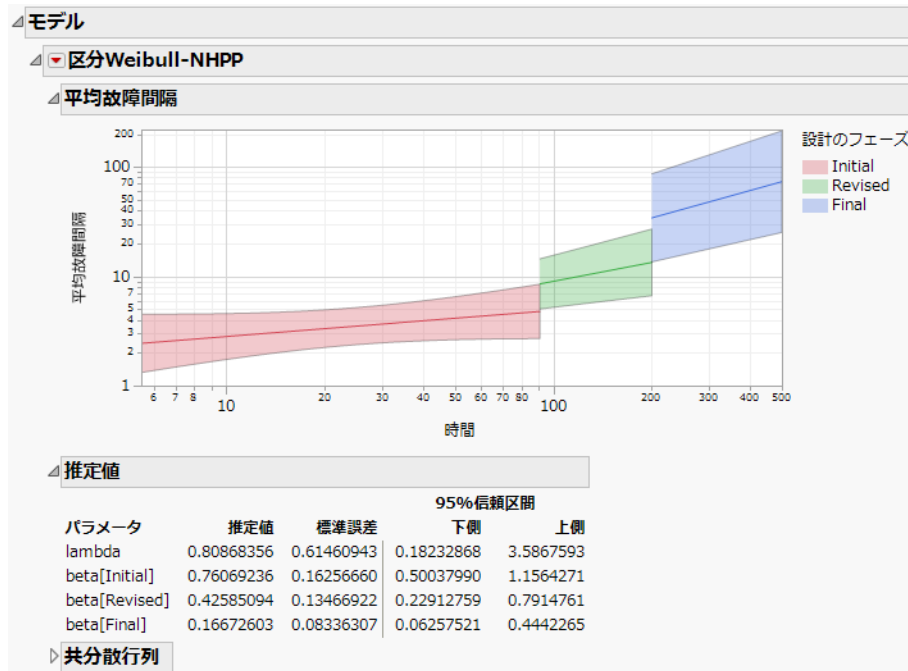
図11.24 「平均故障間隔」グラフ
