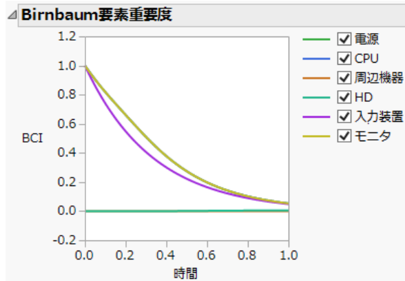
図12.21 Birnbaum要素重要度のグラフ
