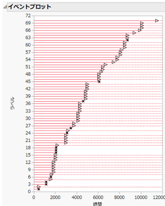
図3.7 右側打ち切りデータのイベントプロット
