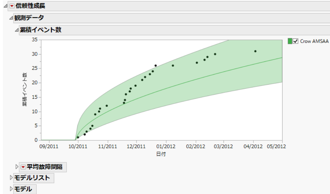
図11.25 AMSAAモデルをあてはめた場合の「累積イベント数」グラフ
