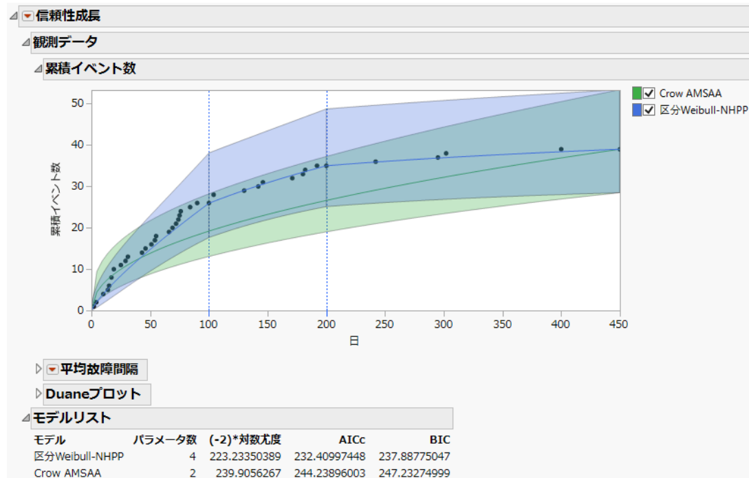
図11.17 「累積イベント数」グラフと「モデルリスト」レポート
