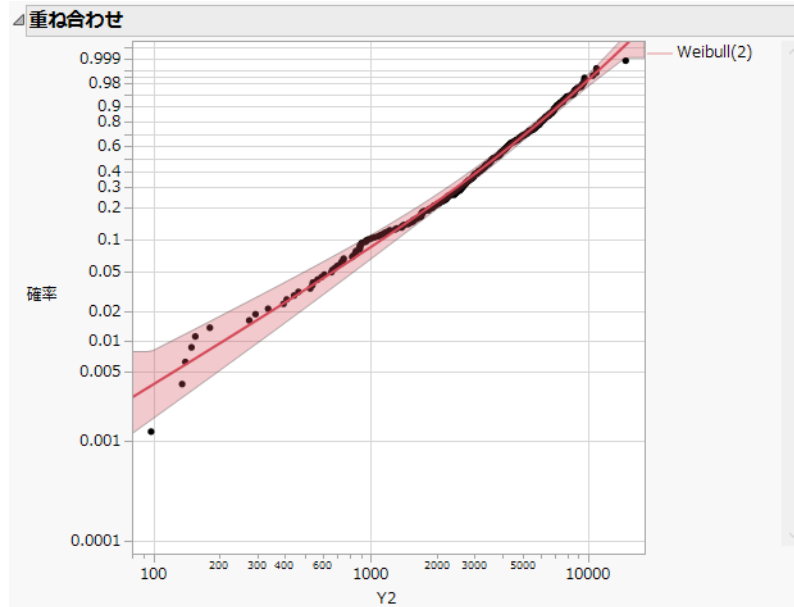
図3.24 Weibull(2)競合リスク混合分布のあてはめ
