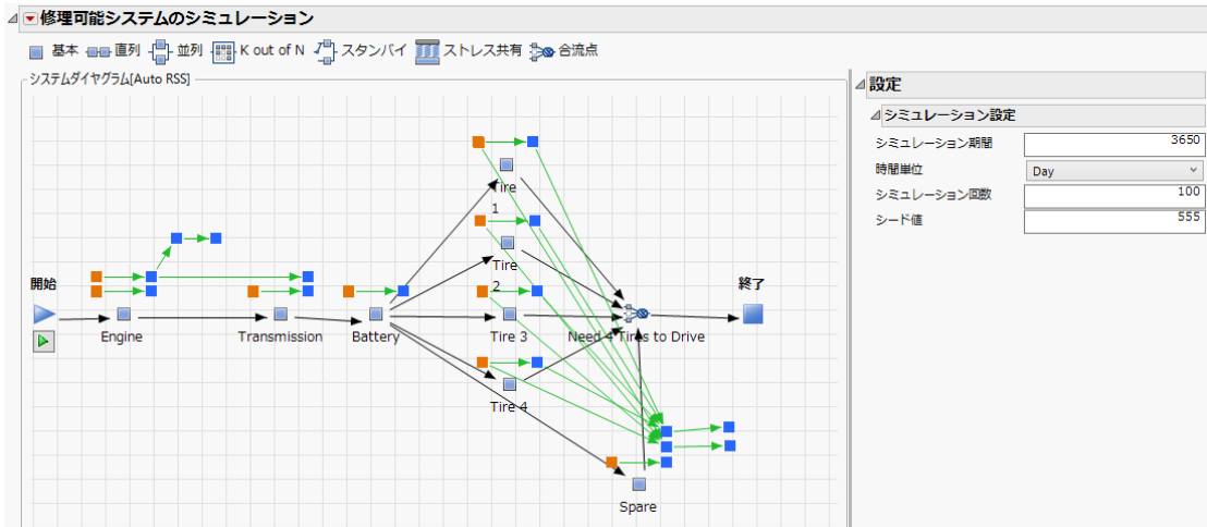
図 13.2 車の修理システムのダイアグラム
