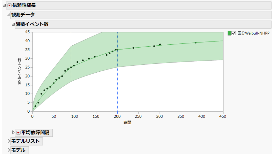
図 11.23 「累積イベント数」グラフ
