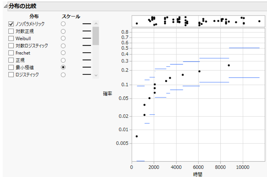
図3.15 最小極値のスケールで表示したノンパラメトリック推定値
