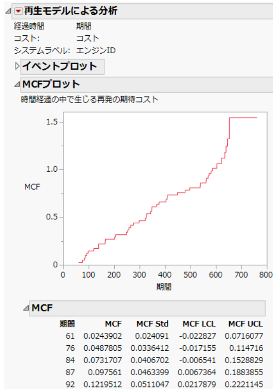
図6.3 再生モデルによる分析のMCFプロットと表の一部
