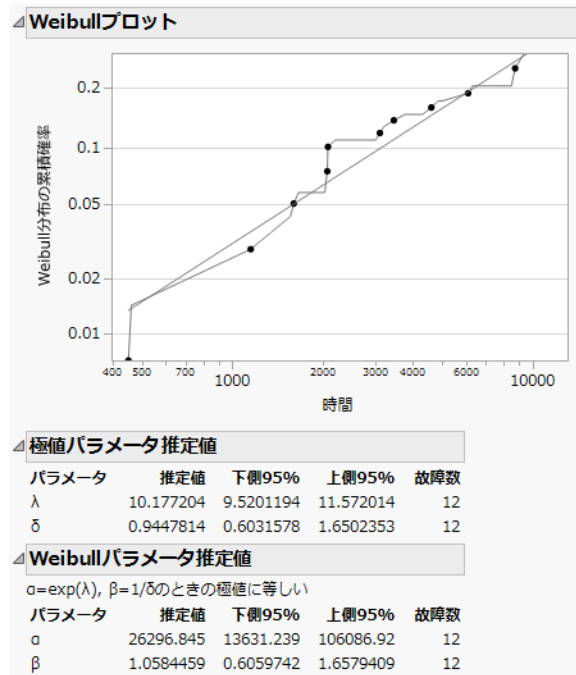
図14.9 「Fan」データのWeibullプロット
