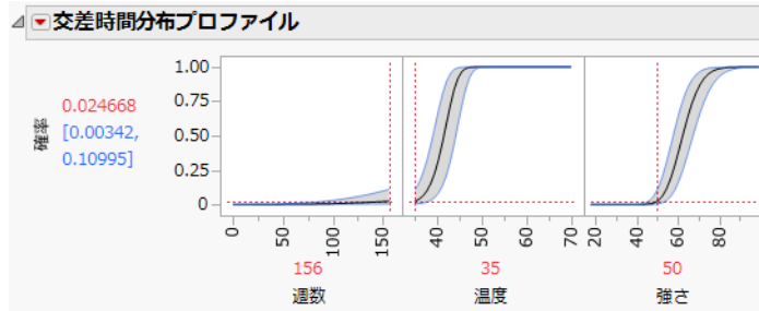
図9.8 交差時間分布プロファイル
