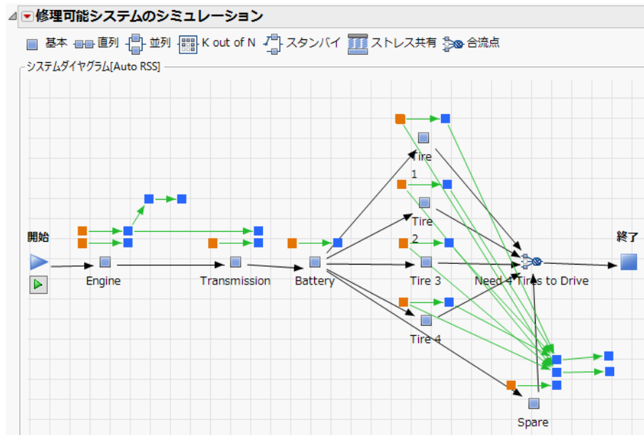
図13.1 修理可能なシステムのシミュレーションダイアグラム
