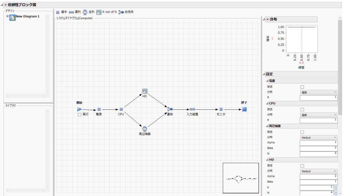
図 12.1 信頼性ブロック図の例
