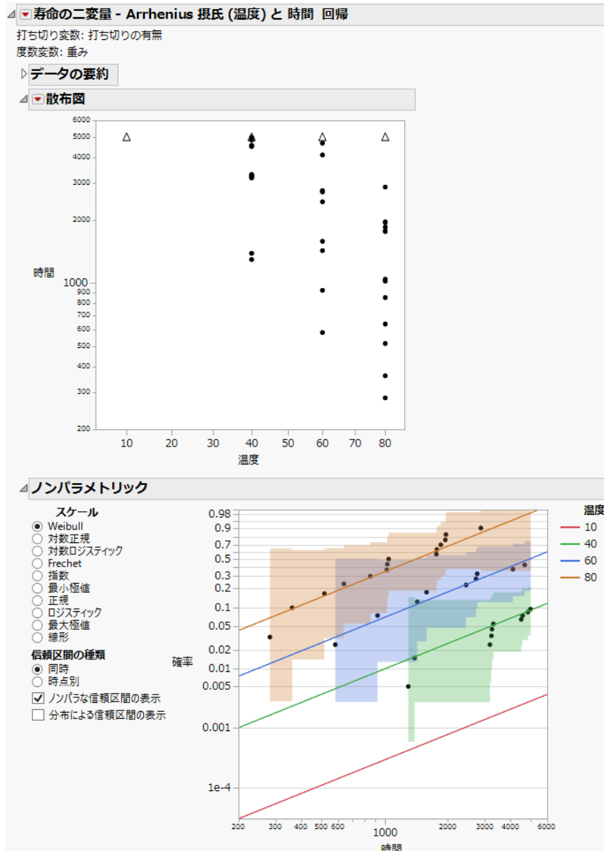
図4.3 「寿命の二変量」レポートウィンドウ
