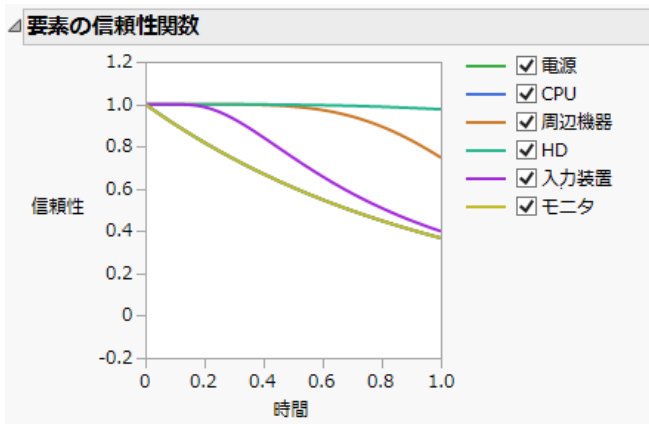
図12.25 要素の信頼性関数
