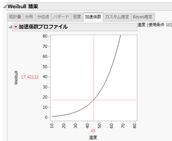
図4.17 Weibull加速係数プロファイル
