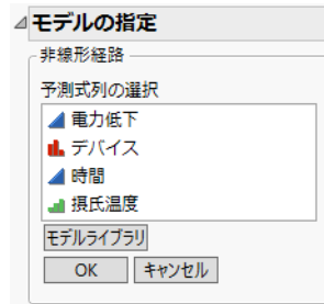
図7.10 列の選択
