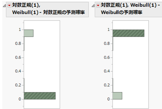
図3.22 混合確率のヒストグラム
