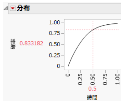
図12.18 分布
