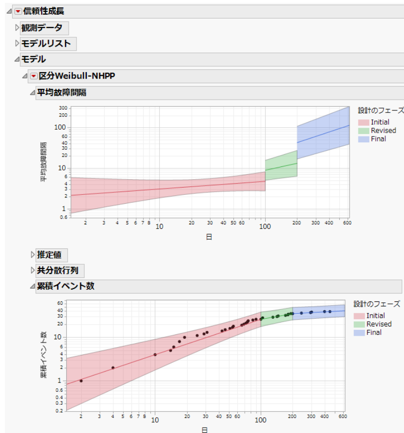
図11.1 フェーズが3つある信頼性成長モデルの例
