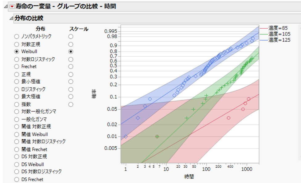
図3.17 Weibull分布のグループ間比較
