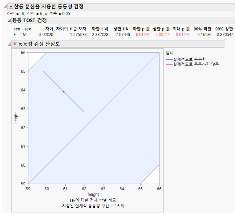
그림 6.30 동등성 검정의 예
