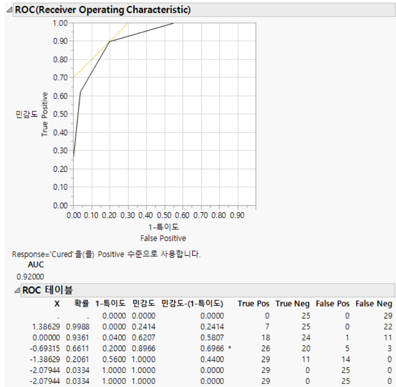
그림 8.9 ROC 곡선 및 테이블의 예
