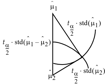
그림 6.45 t -검정 통계량의 기하학적 관계
