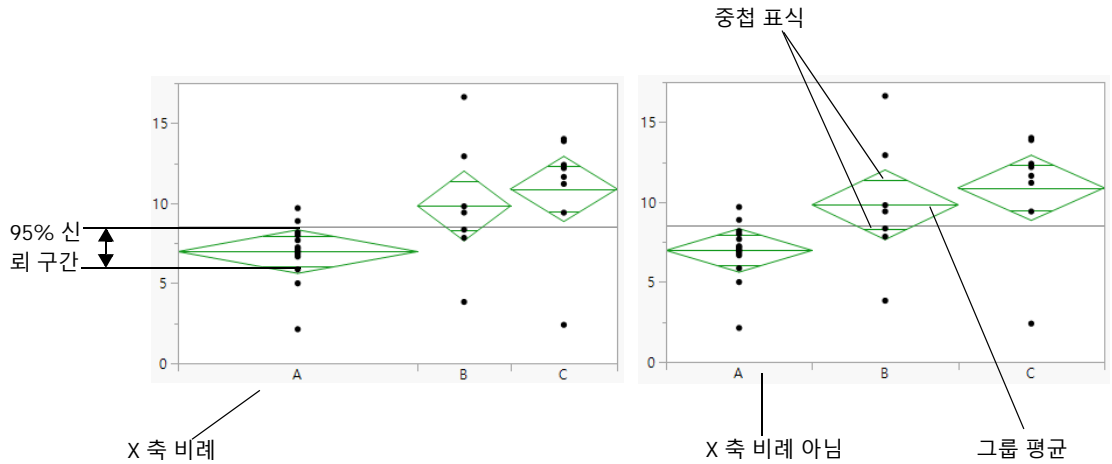
그림 6.8 평균 다이아몬드 및 X 축 비례 옵션의 예
