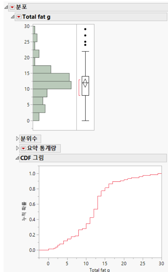
그림 3.10 CDF 그림
