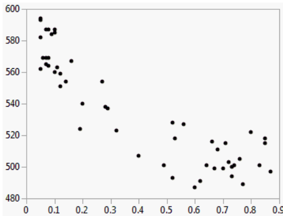
그림 5.4 이변량 그림
