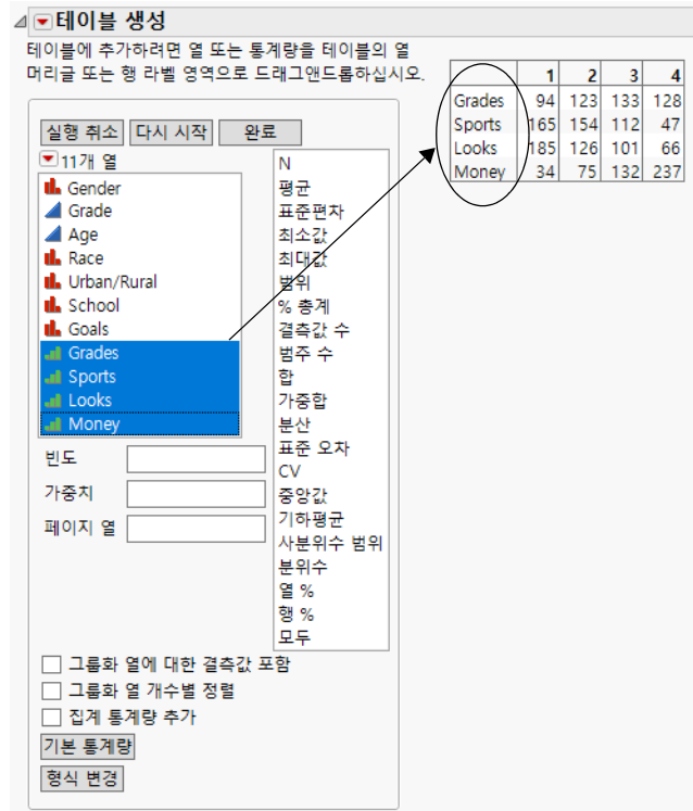
그림 9.20 범주별 열
