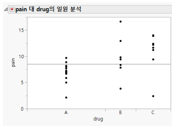
그림 6.1 일원 분석
