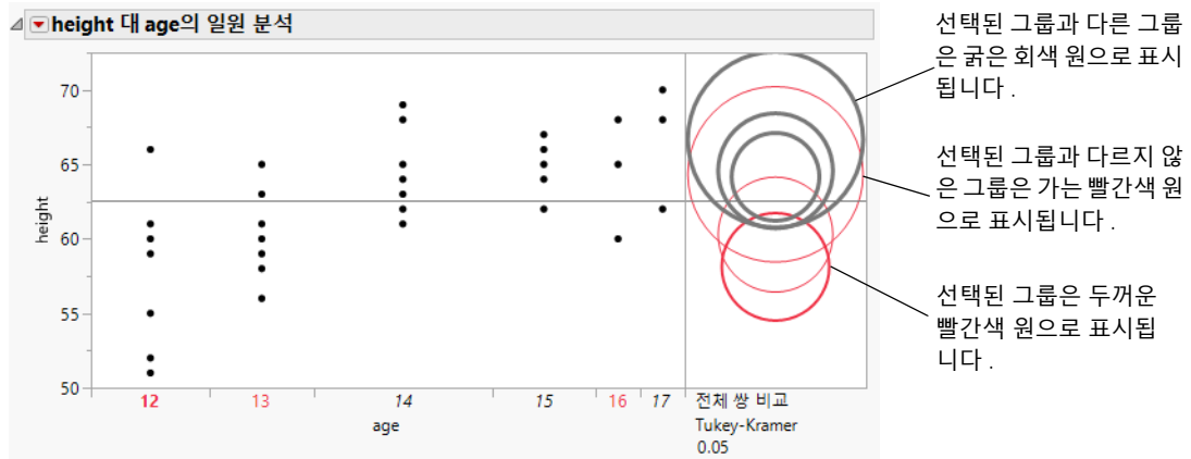
그림 6.12 비교 원 강조 표시
