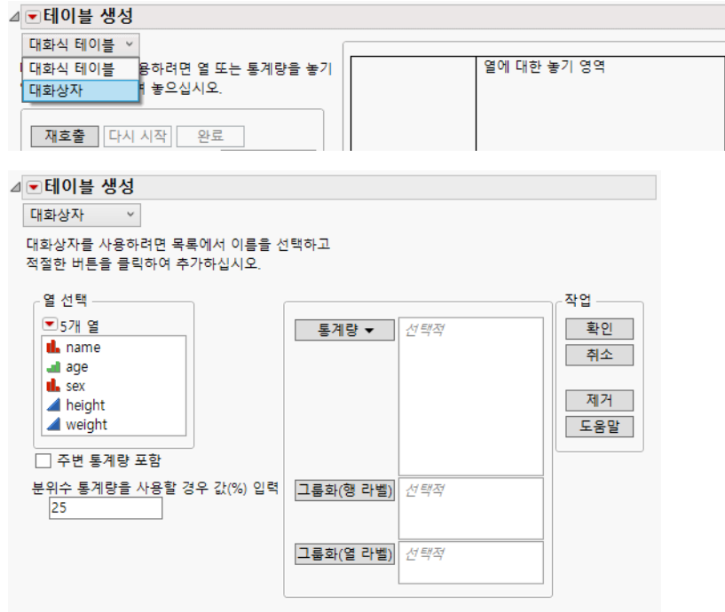
그림 9.8 대화상자 사용
