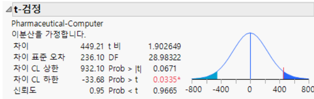
그림 6.26 t-검정 결과
