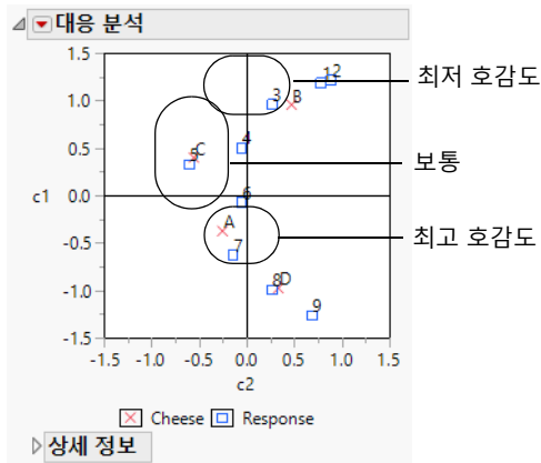
그림 7.11 대응 분석 그림의 예
