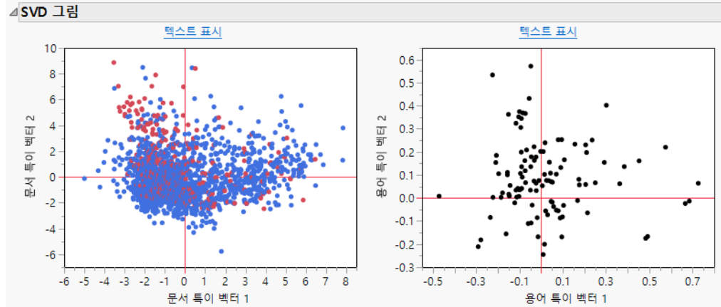
그림 12.15 Narrative Cause 에 대한 SVD 그림
