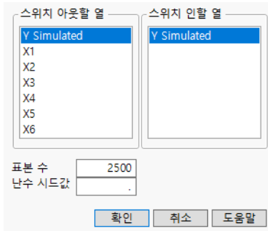
그림 10.21 시뮬레이션 창
