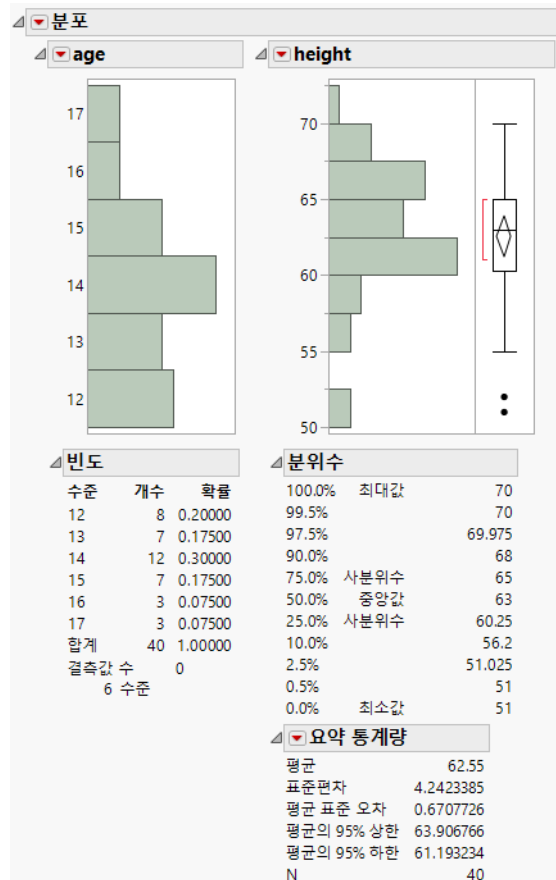
그림 3.5 초기 분포 보고서 창
