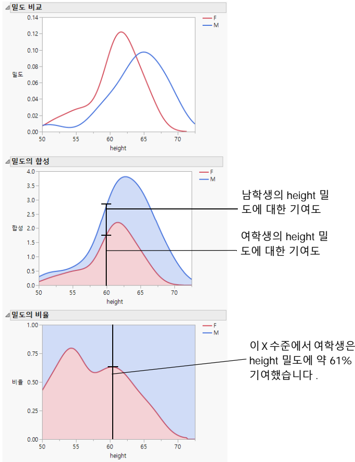
그림 6.36 밀도 옵션의 예
