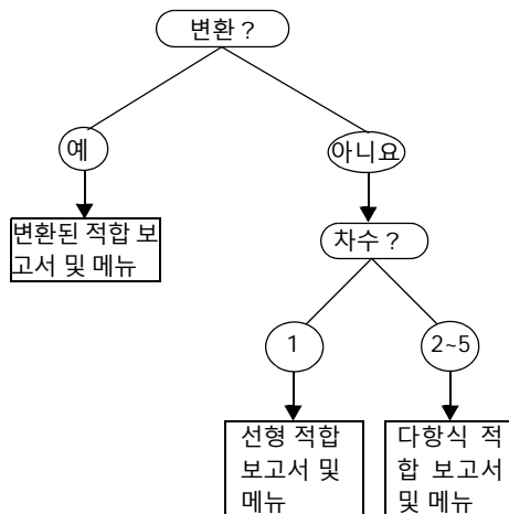
그림 5.14 특수 적합 순서도의 예
