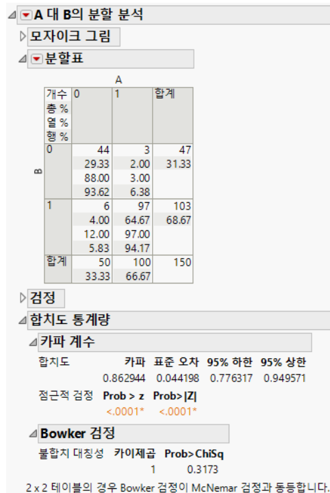
그림 7.14 합치도 통계량 보고서의 예
