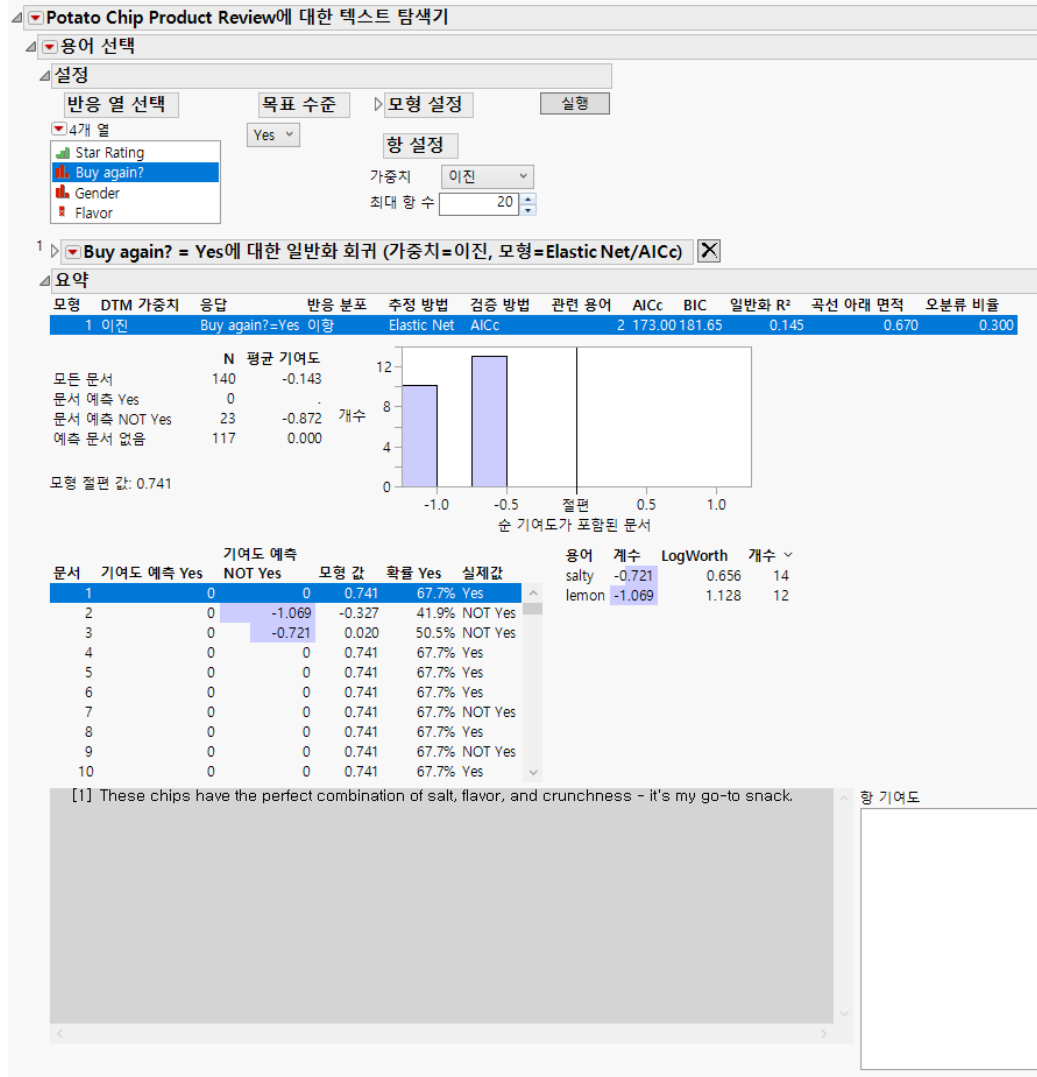
그림 12.12 용어 선택 보고서
