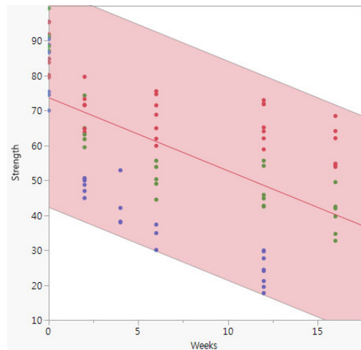
예측 구간
