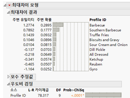
최대차이
