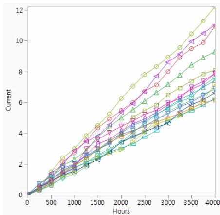
중첩
