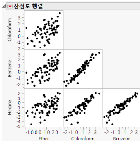
그림 4.16 산점도 행렬
