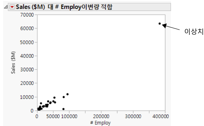
그림 8.2 초기 산점도
