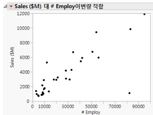
그림 4.9 산점도의 예
