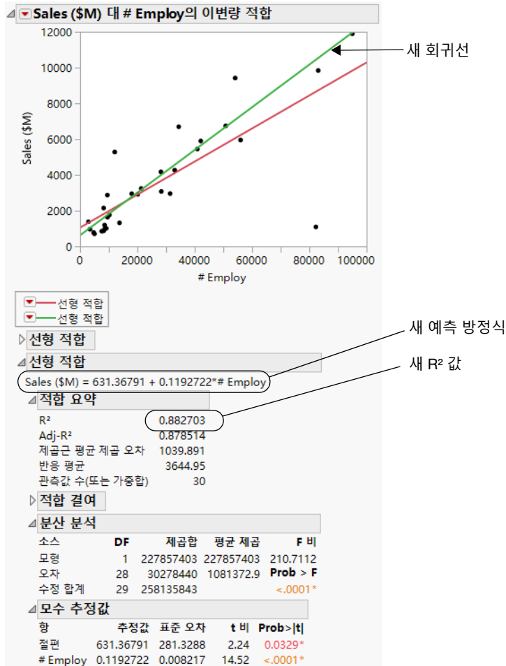
그림 5.14 모형 비교
