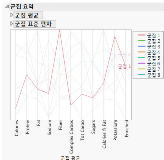
그림 6.15 군집 요약
