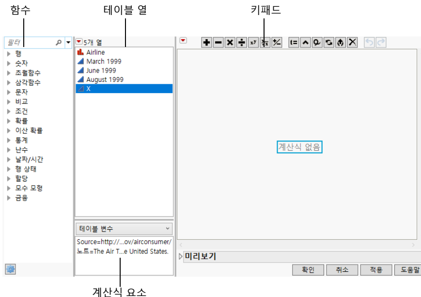
그림 3.12 계산식 편집기
