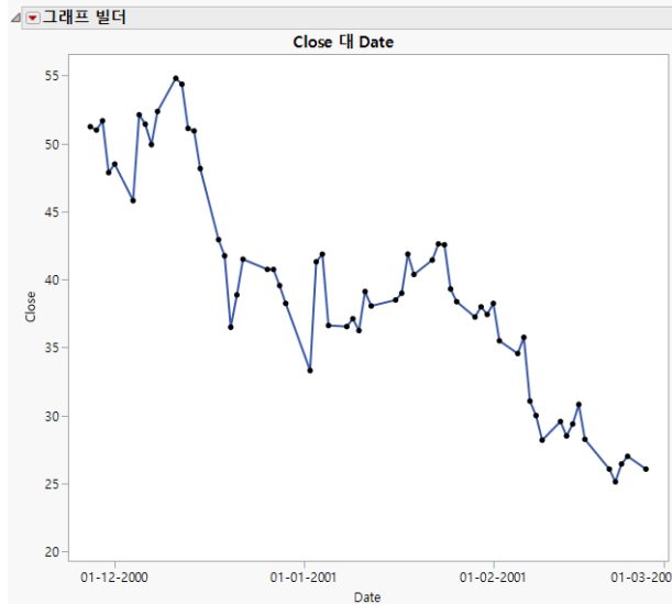
그림 4.34 연결된 점
