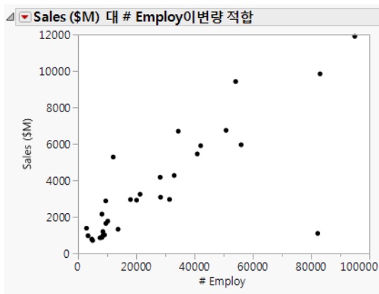
그림 8.3 업데이트된 산점도
