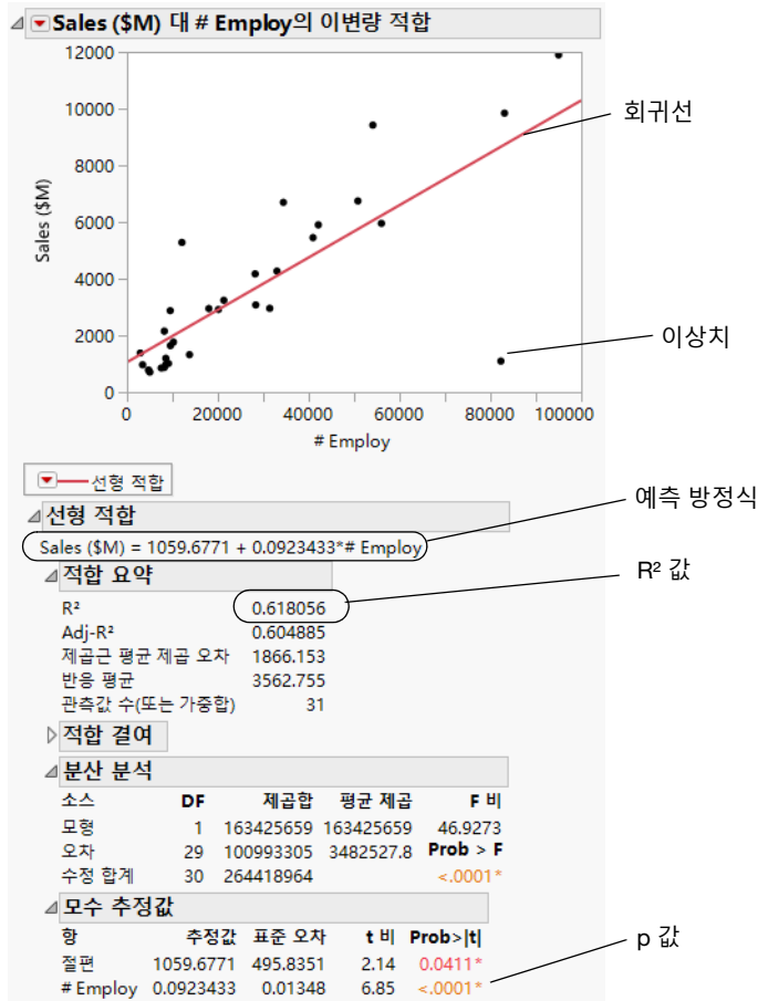
그림 5.13 회귀선
