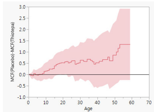
MCF 그림
