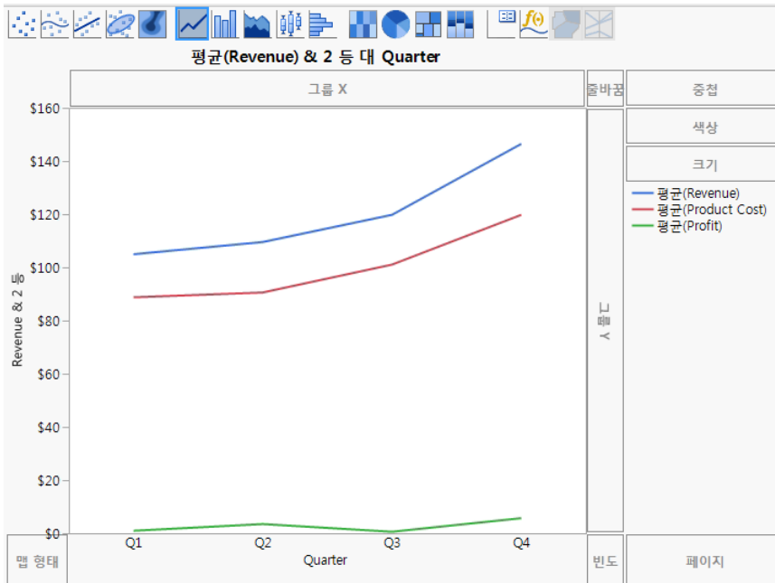
그림 4.24 선 그림
