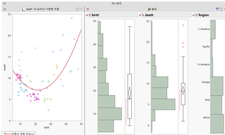
그림 7.19 결합된 창
