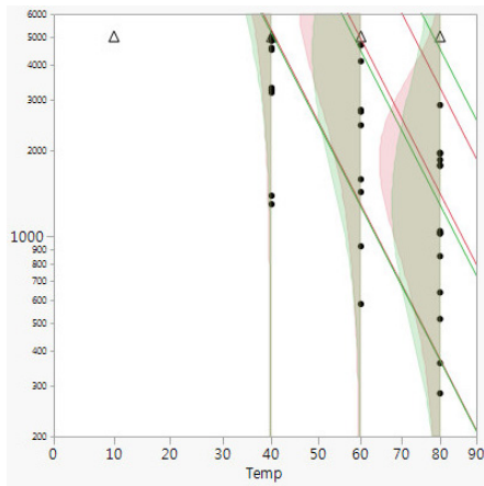
산점도
