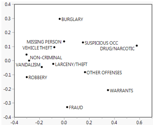
다차원 척도법
