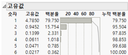
그림 4.5 고유값
