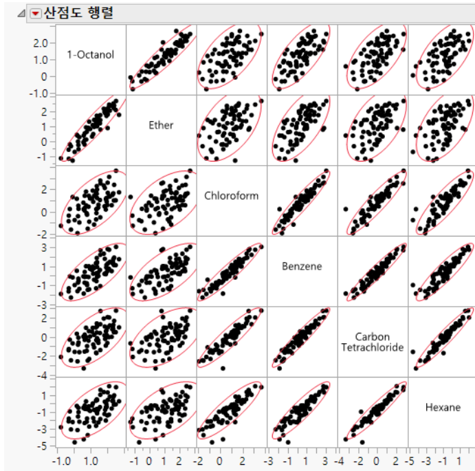
그림 3.4 산점도 행렬
