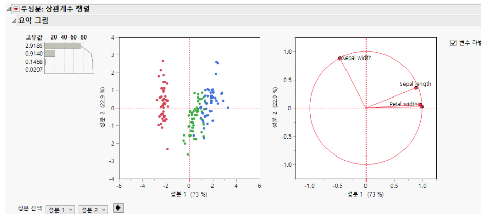
그림 4.1 주성분의 예
