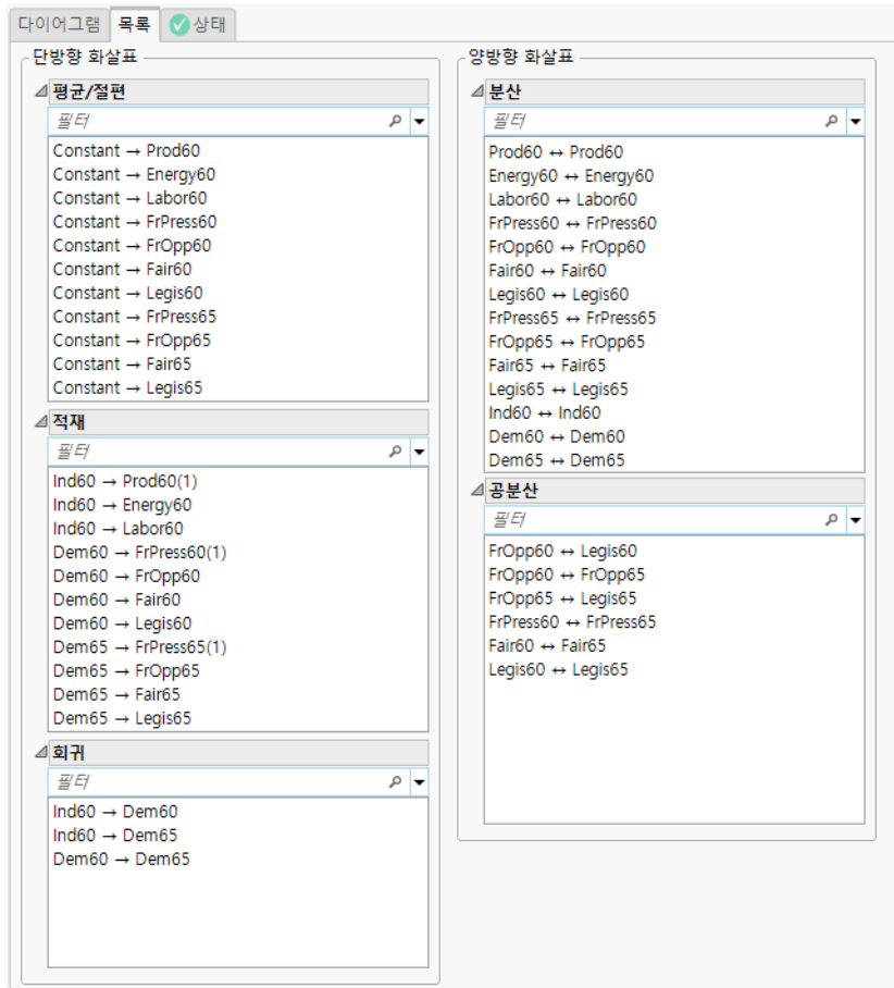
그림 8.7 공분산
