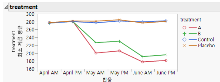
그림 10.5 treatment 그래프
