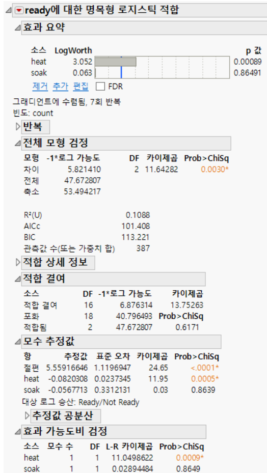
그림 12.2 명목형 로지스틱 적합 보고서
