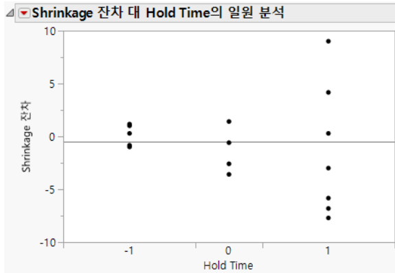
그림 11.6 잔차 대 산포 효과
