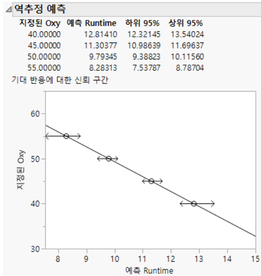
그림 3.31 역추정 예측 보고서
