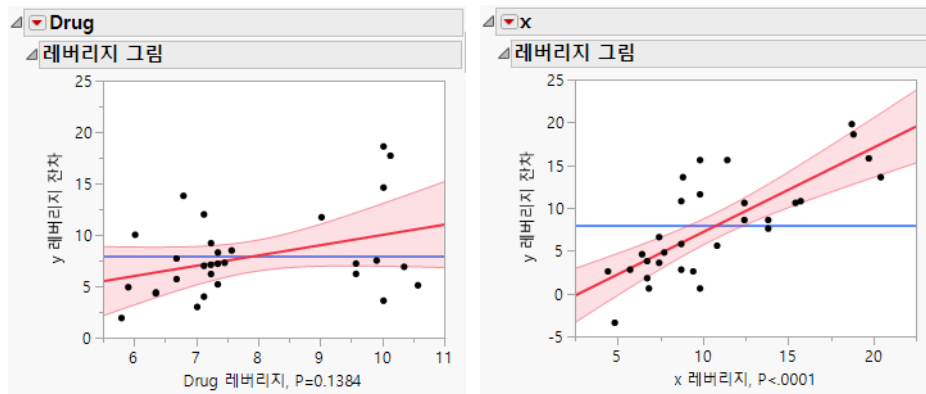
그림 4.5 약물 검정 데이터에 대한 레버리지 그림 비교
