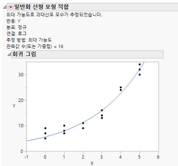
그림 13.1 일반화 선형 모형 적합의 예
