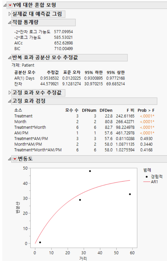
그림 8.20 AR(1) 공분산 구조에 대한 혼합 모형 보고서
