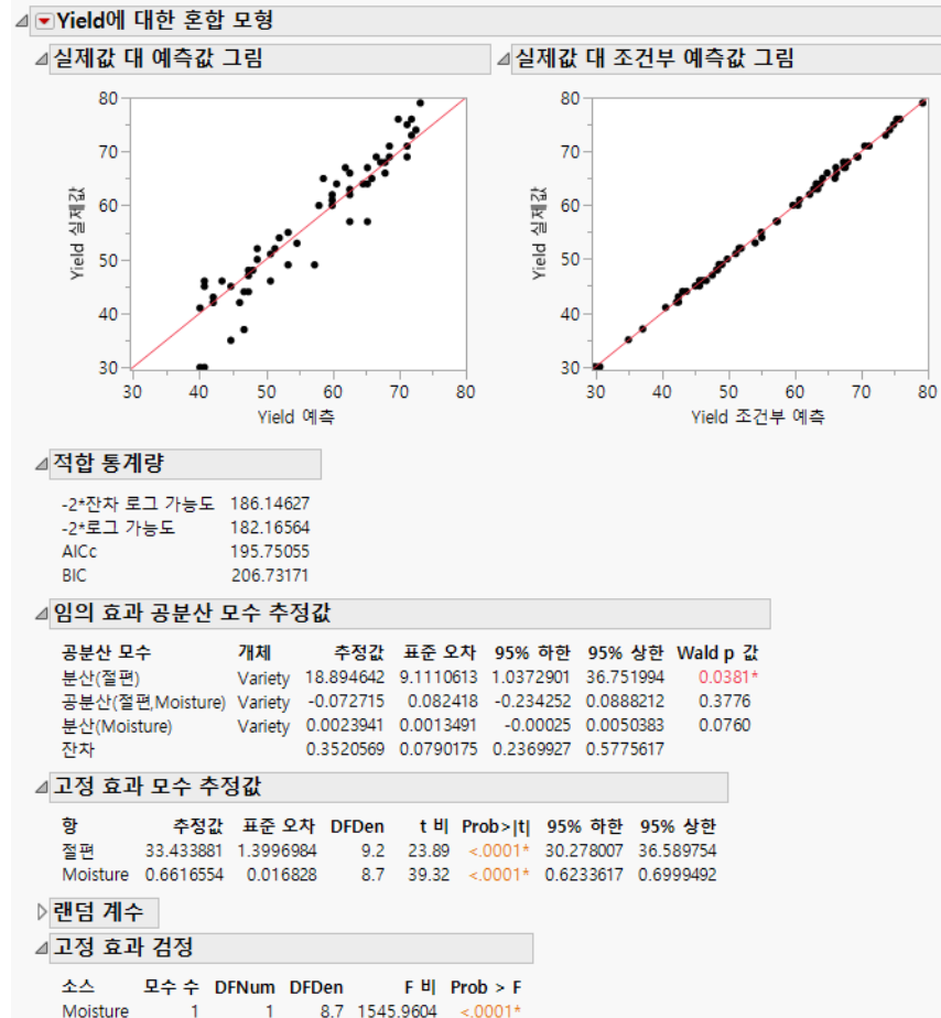
그림 8.5 혼합 모형 보고서
