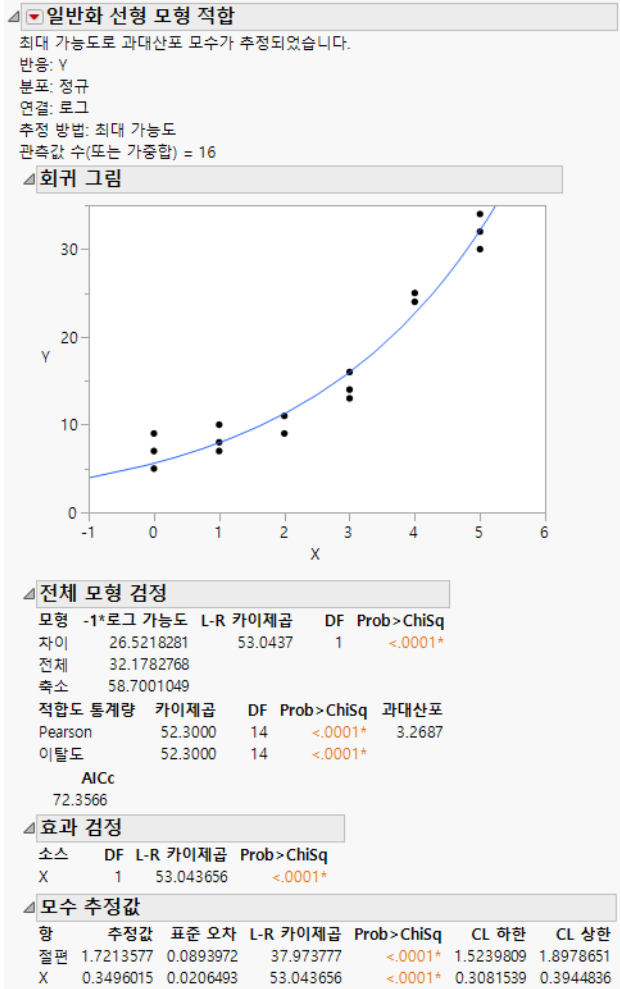
그림 13.9 모형 결과
