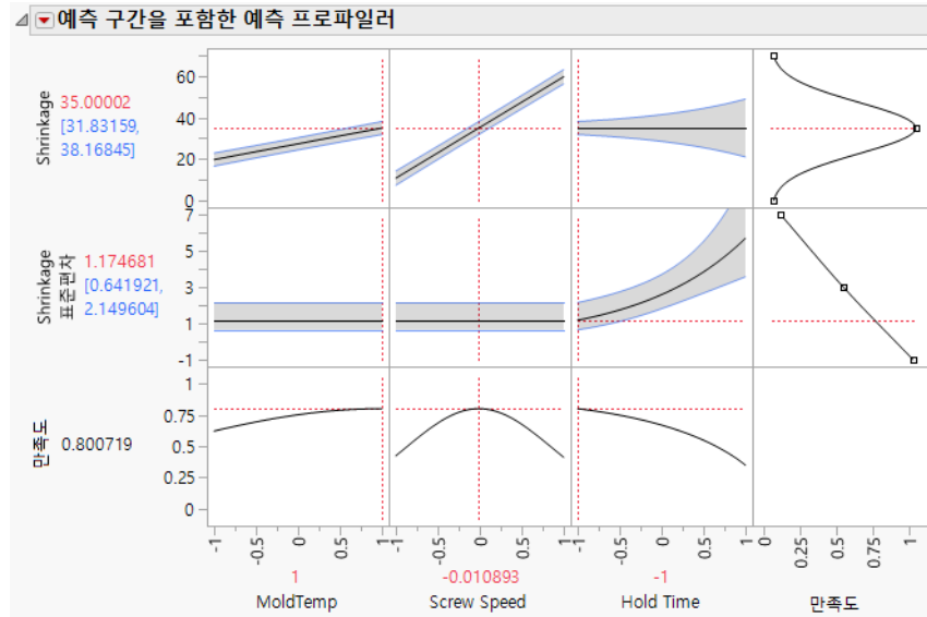
그림 11.7 예측 구간을 포함한 목표값 일치 및 분산 최소화 프로파일러
