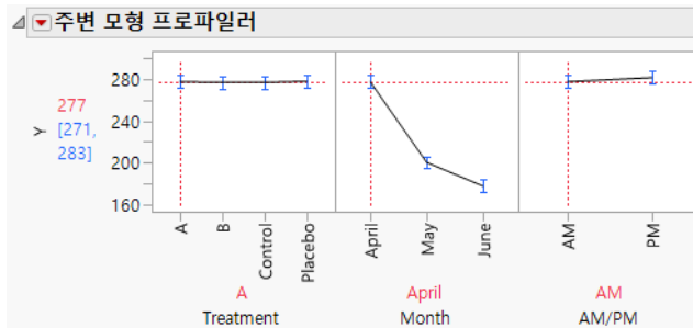
그림 8.21 Treatment A 에 대한 주변 프로파일러 그림
