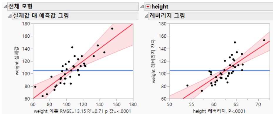
그림 3.52 전체 모형 및 효과 레버리지 그림
