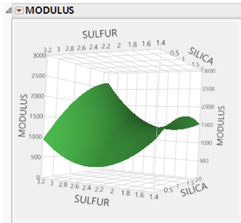
그림 3.9 안장 모양 표면을 사용한 표면 프로파일러 그림
