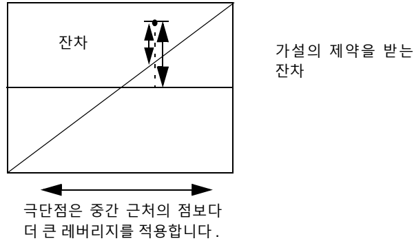
그림 3.50 일반 레버리지 그림의 예
