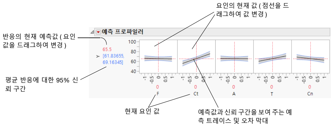
그림 3.43 예측 트레이스 그림
