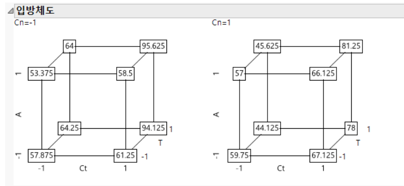
그림 3.47 입방체도
