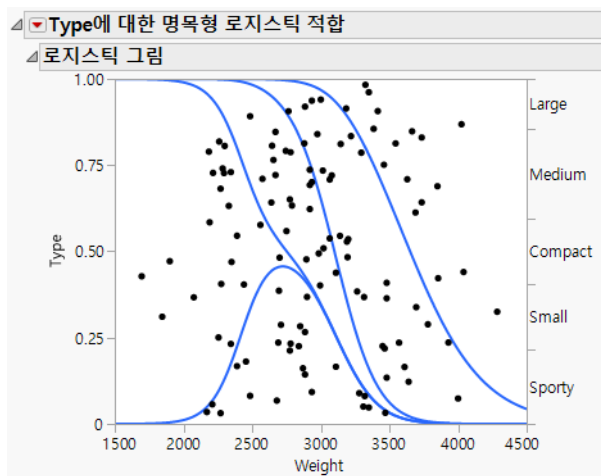
그림 12.1 명목형 로지스틱 회귀 모형에 대한 로지스틱 그림
