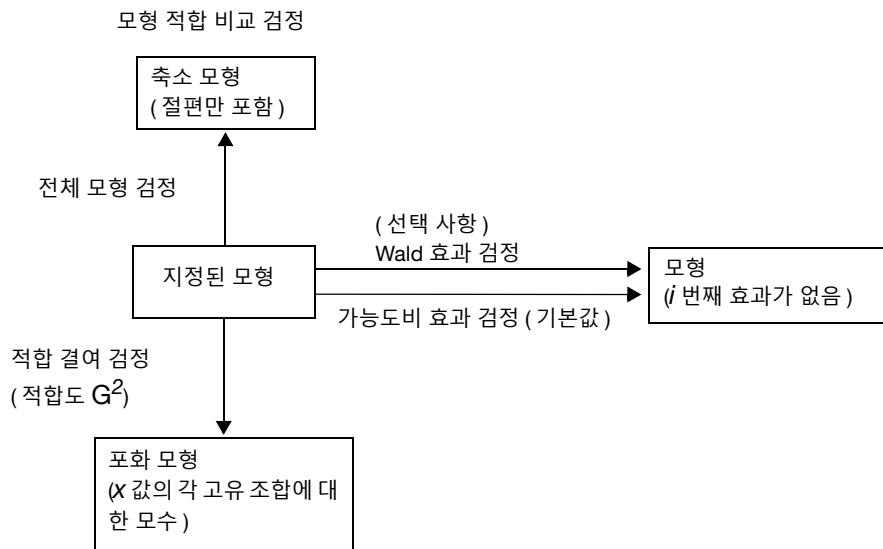
그림 12.14 통계적 검정의 관계
