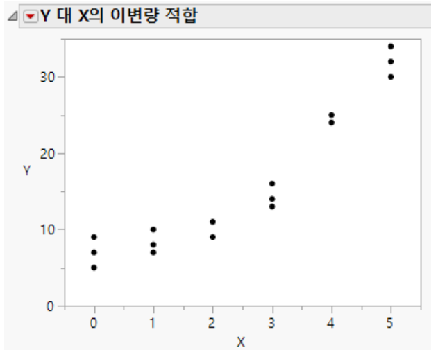
그림 13.8 X 로 Y 적합 결과
