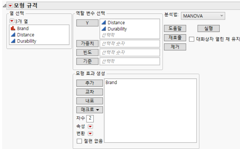
그림 10.1 MANOVA 설정
