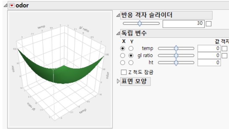
그림 3.49 표면 그림
