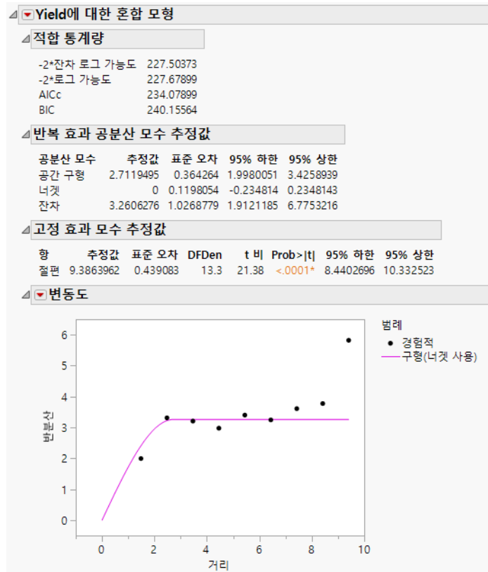
그림 8.34 공간 구형 (너겟 사용) 에 대한 혼합 모형 보고서
