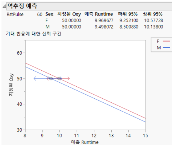
그림 3.33 다중 회귀 모형에 대한 역추정 예측 보고서
