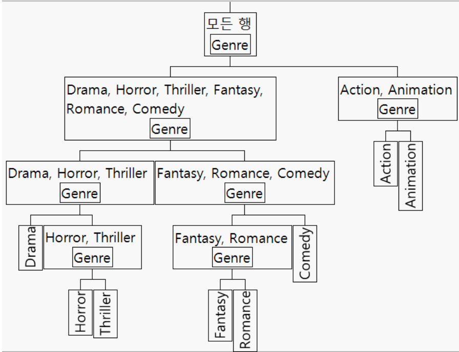
그림 5.17 계층적 코딩에 사용되는 분할을 보여 주는 트리
