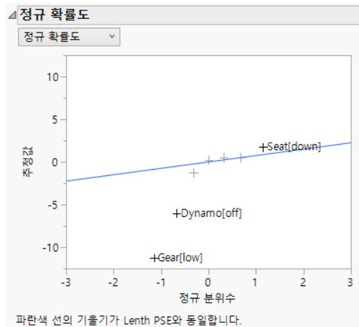
그림 3.39 정규 확률도
