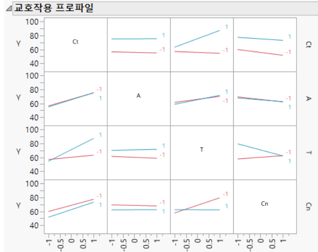
그림 3.44 교호작용 그림
