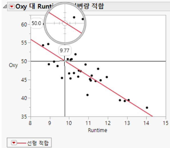
그림 3.29 Fitness.jmp 에 대한 이변량 적합
