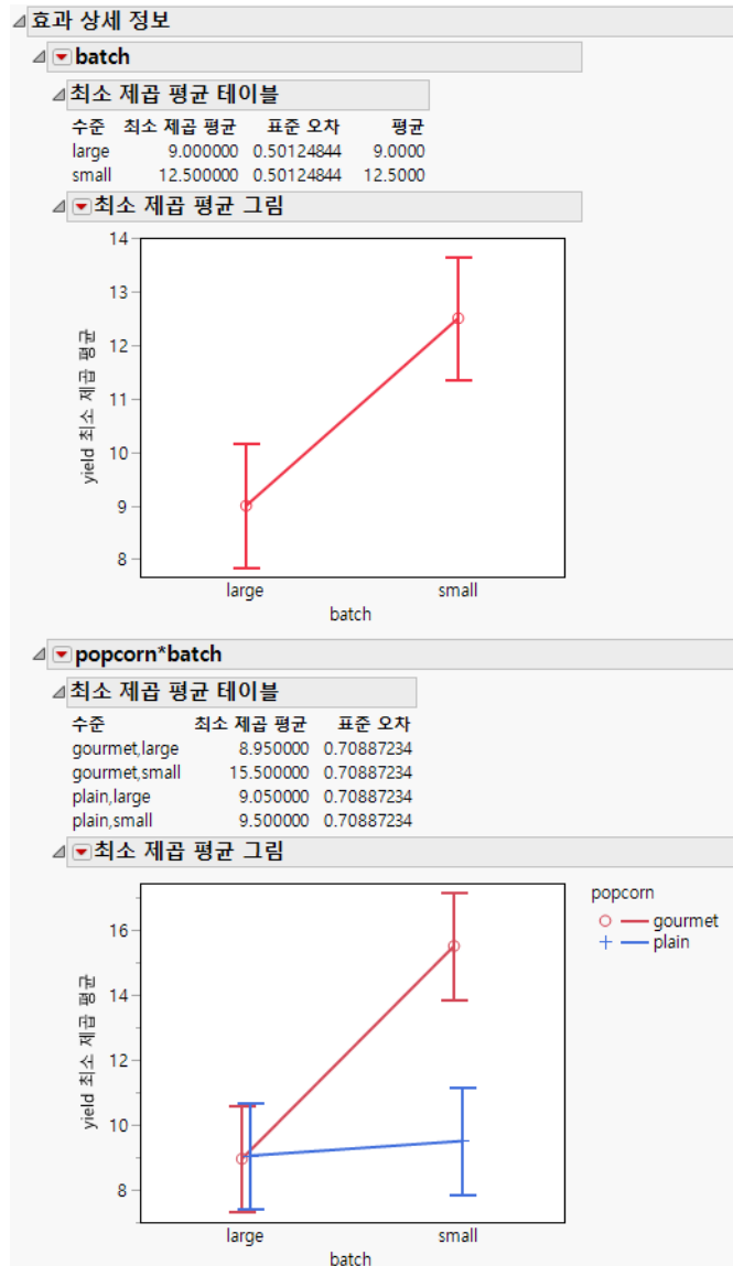
그림 3.12 두 효과에 대한 최소 제곱 평균 테이블 및 최소 제곱 평균 그림
