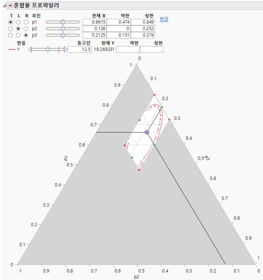
그림 3.46 혼합물 프로파일러
