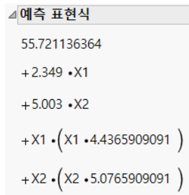
그림 4.13 예측 표현식
