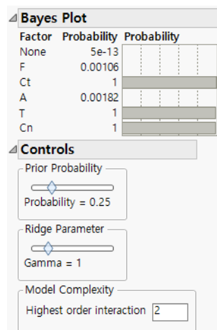
그림 4.24 요인 활동에 대한 Bayes 그림
