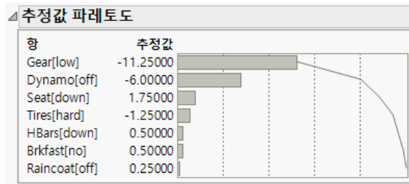
그림 3.42 파레토도
