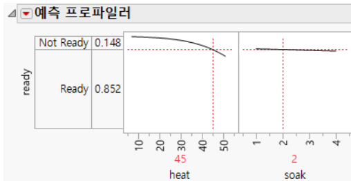
그림 12.3 예측 프로파일러
