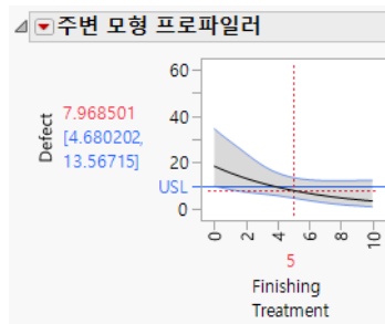
그림 9.14 결함 수에 대한 주변 모형 프로파일러
