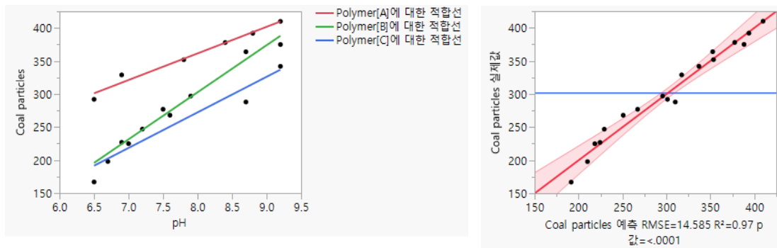
그림 3.1 표준 최소 제곱 그림의 예
