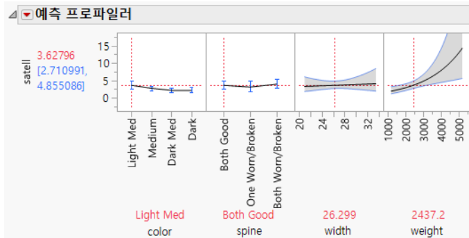
그림 13.3 satell 에 대한 예측 프로파일러
