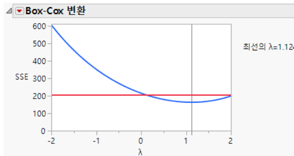
그림 3.48 Y의 Box-Cox 변환
