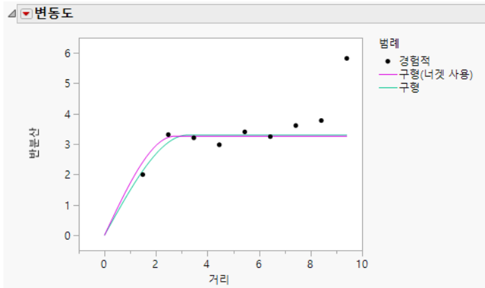
그림 8.35 혼합 모형 보고서의 변동도
