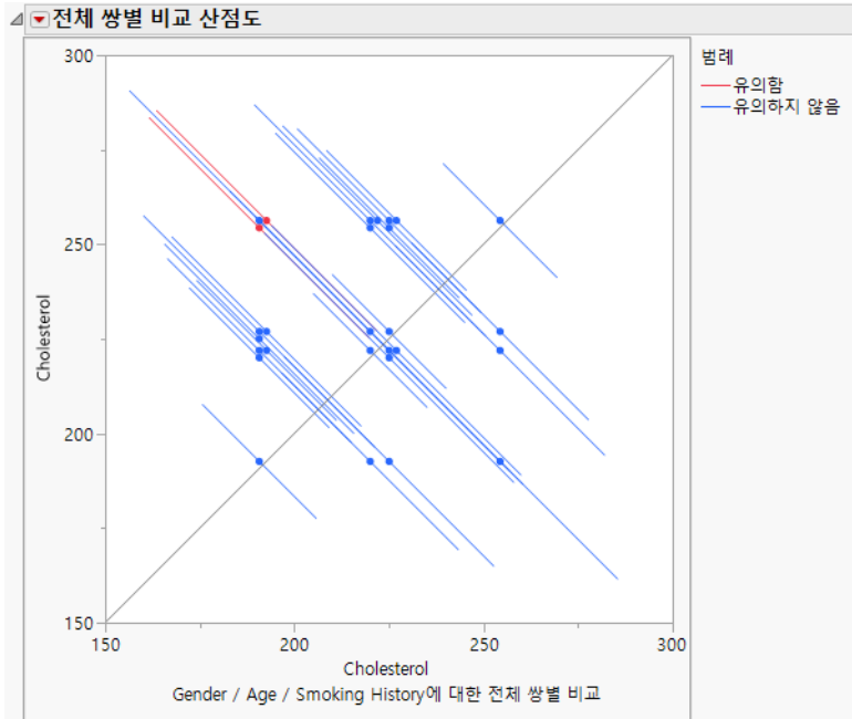
그림 3.57 사용자 정의 비교를 위한 전체 쌍별 비교 산점도
