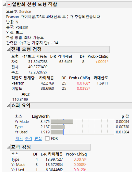
그림 13.7 오프셋을 사용하는 Poisson 모형에 대한 보고서 (일부분)
