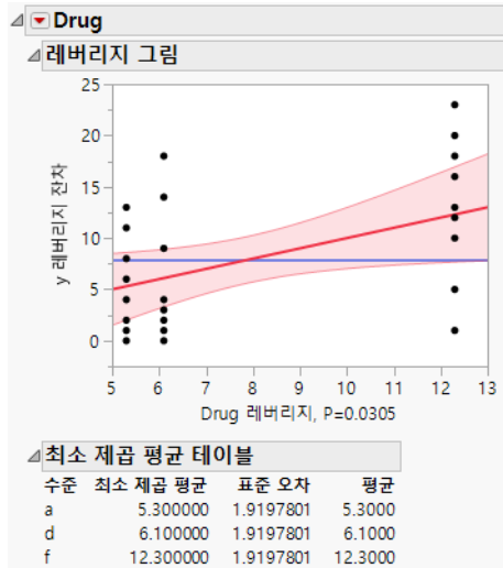
그림 4.1 Drug 에 대한 레버리지 그림 및 최소 제곱 평균 테이블
