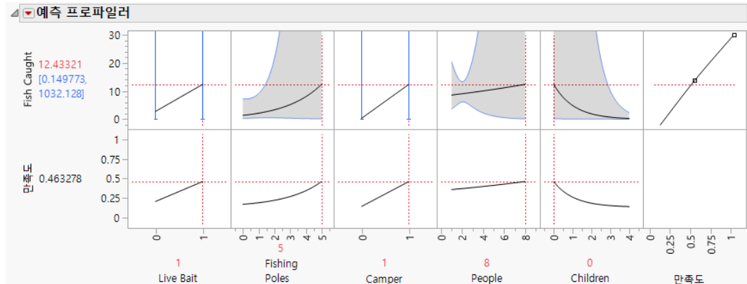
그림 7.7 Fish Caught 가 최대화된 예측 프로파일러
