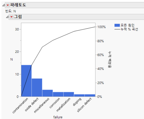
그림 15.8 원인이 분리된 파레토도
