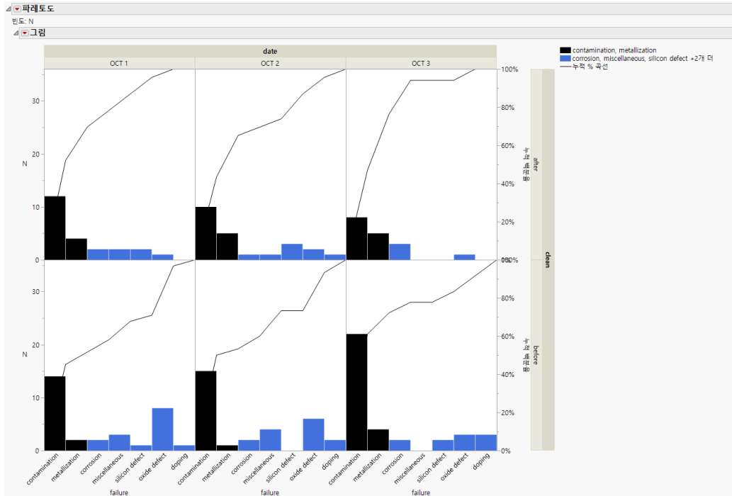
그림 15.15 이원 비교 파레토도
