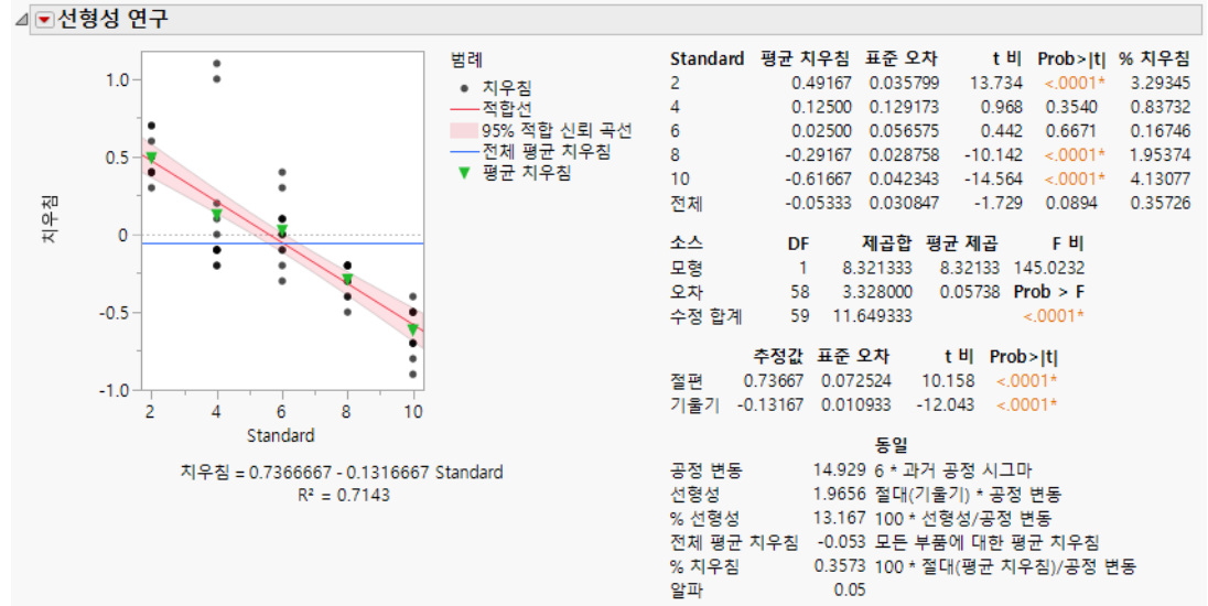
그림 6.12 선형성 연구
