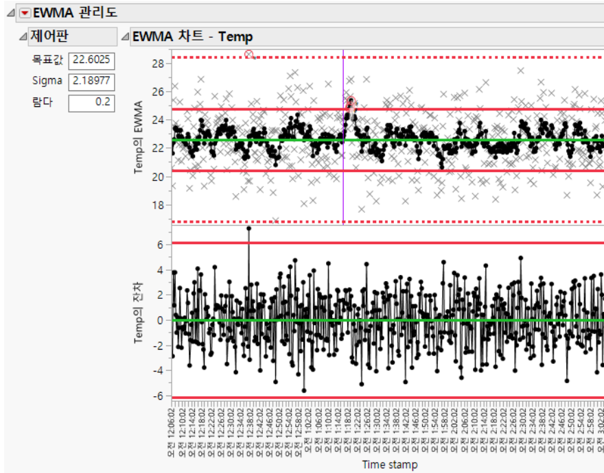
그림 11.8 상수 한계를 사용한 EWMA 차트
