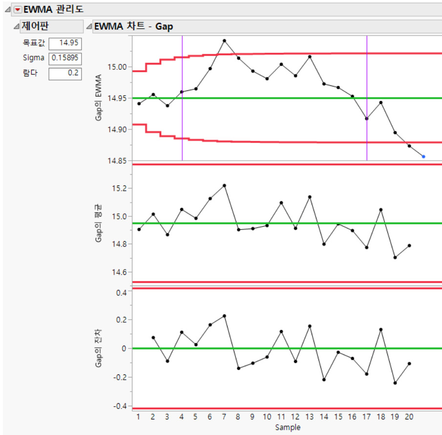
그림 11.4 EWMA 관리도 보고서
