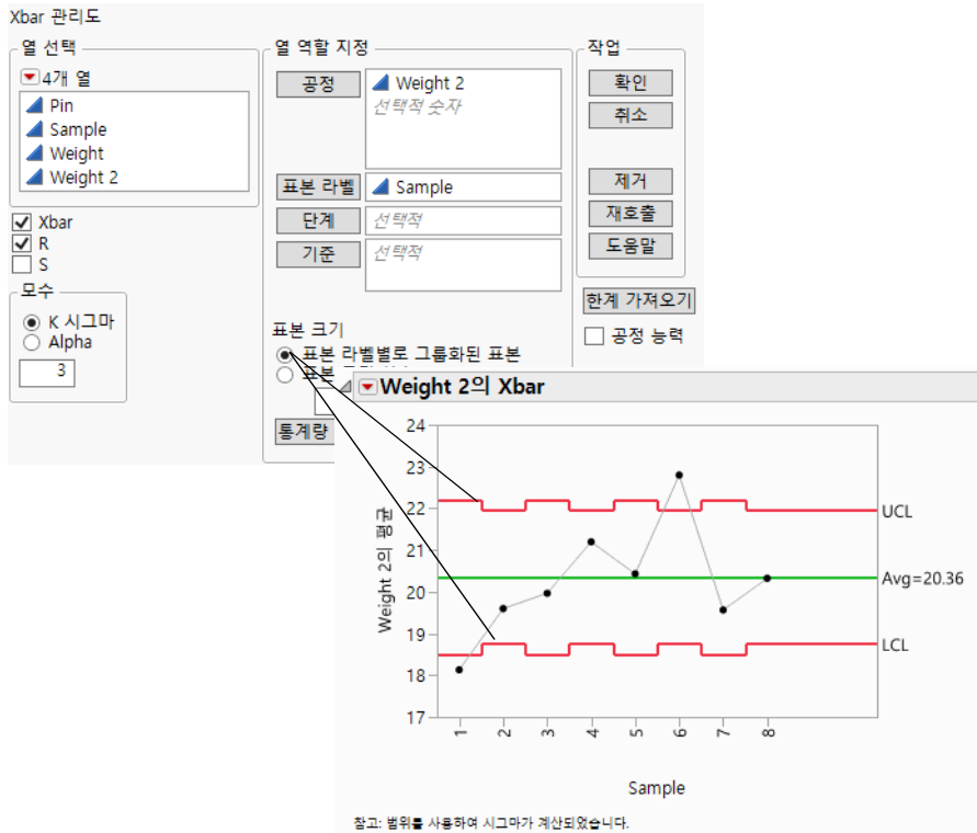
그림 14.4 부분군 표본 크기가 같지 않은 계량형 차트
