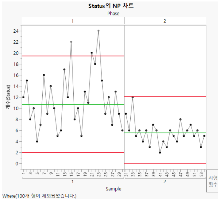
그림 3.27 단계 (Phase) 별 NP 차트
