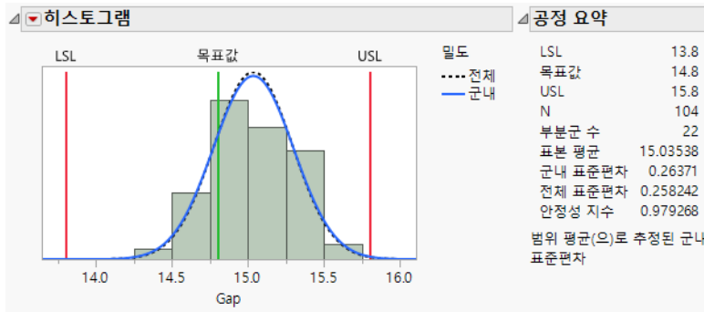
그림 9.22 Gap 에 대한 공정 능력 분석의 히스토그램
