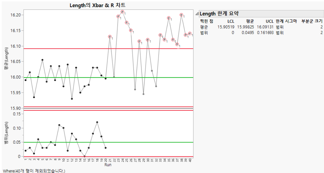
그림 3.12 제외된 데이터가 있는 Length(선 길이)의 Xbar-R 차트
