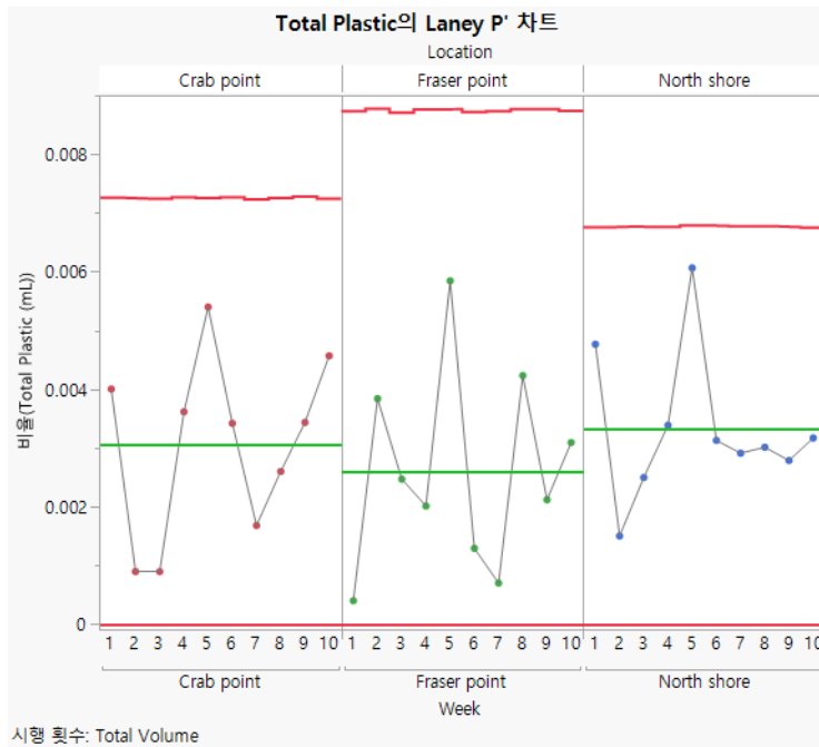
그림 3.25 Water Plastics 에 대한 Laney P' 차트
