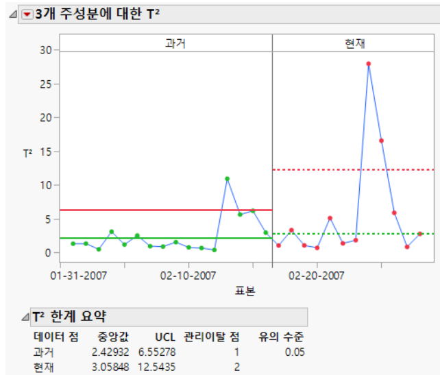
그림 13.9 과거 및 현재 데이터에 대한 T^2 차트
