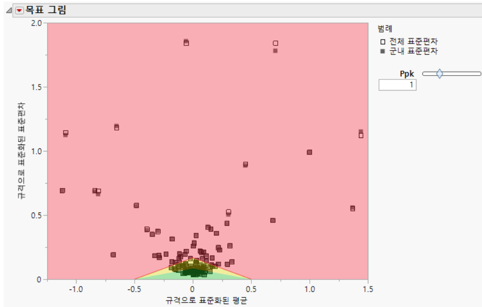
그림 9.11 목표 그림
