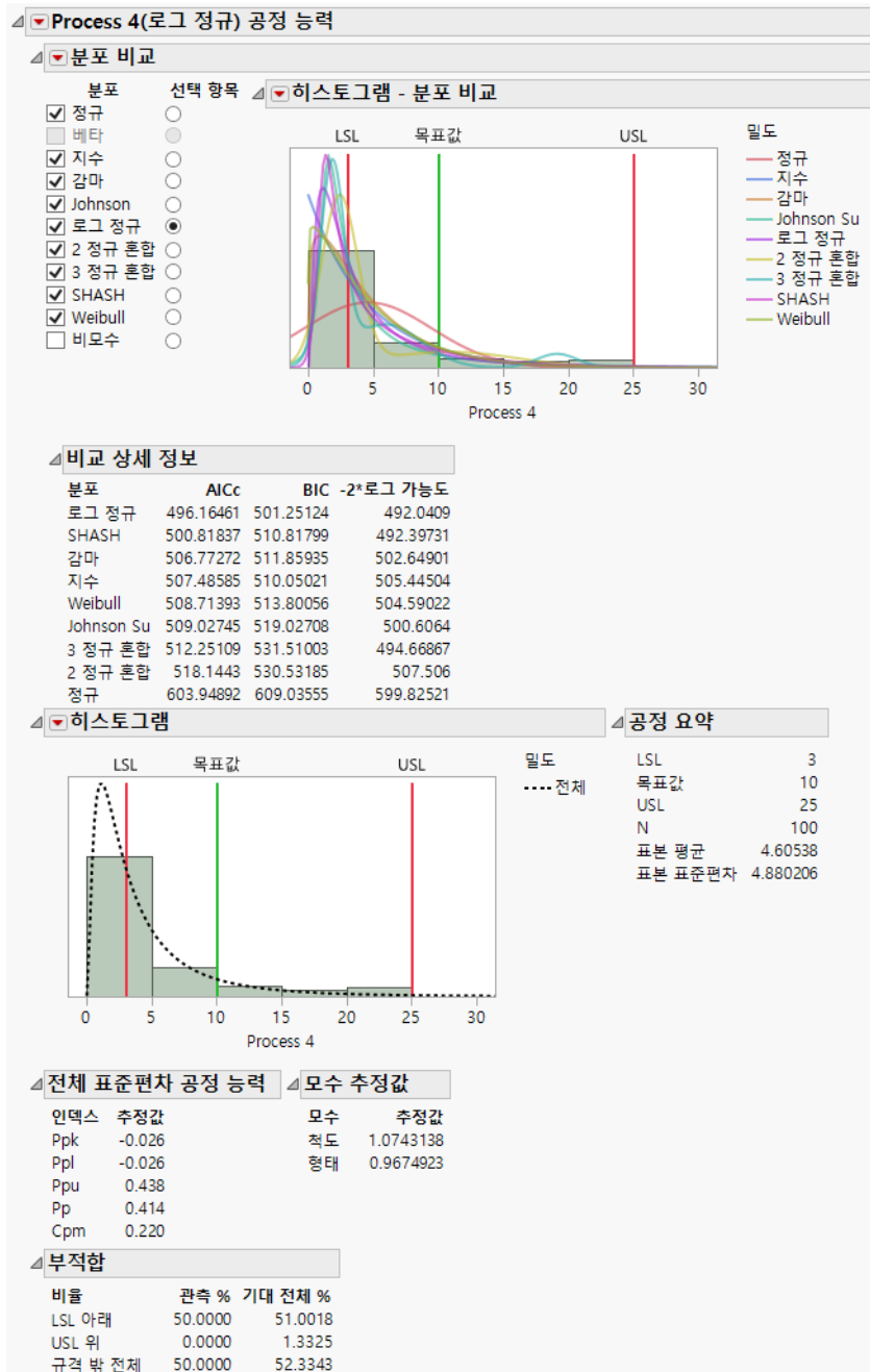
그림 9.5 Process 4의 개별 상세 정보 보고서
