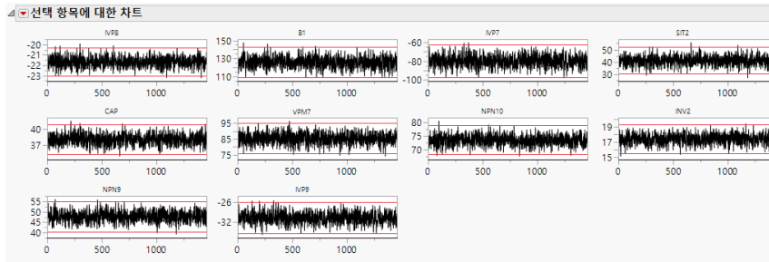
그림 8.3 경보 비율이 가장 높은 공정에 대한 차트
