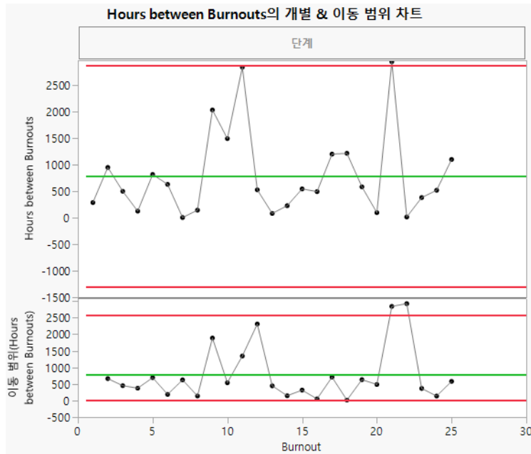
그림 3.32 Hours Between Burnouts( 연소 사이 시간 ) 의 개별값 및 이동 범위 차트
