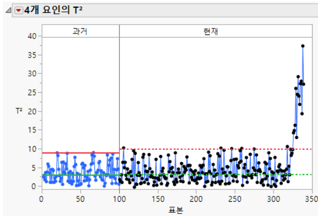
그림 13.10 T^2 차트
