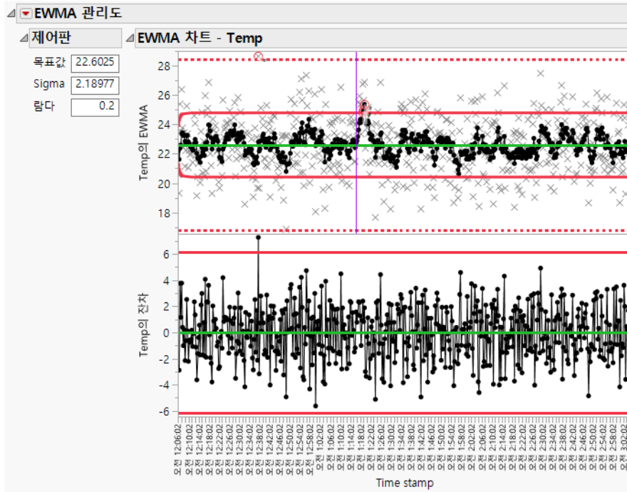
그림 11.7 X 차트가 중첩된 EWMA 차트
