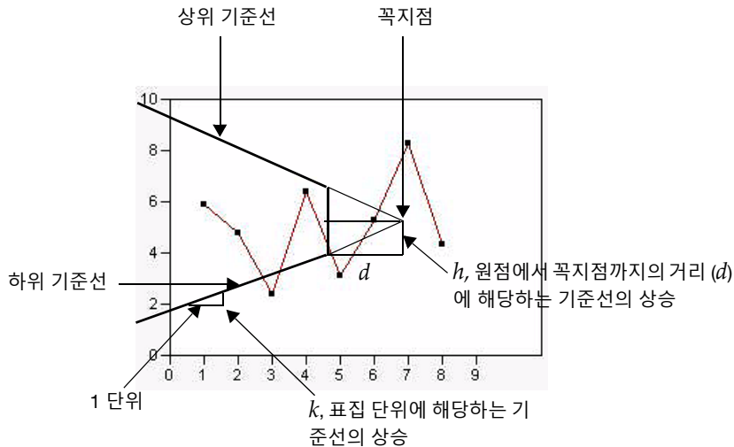
그림 14.9 양측 CUSUM 차트의 V- 마스크
