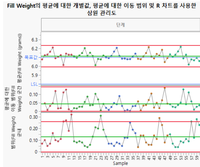
그림 3.34 Fill Weight( 충전 양 ) 에 대한 삼원 관리도
