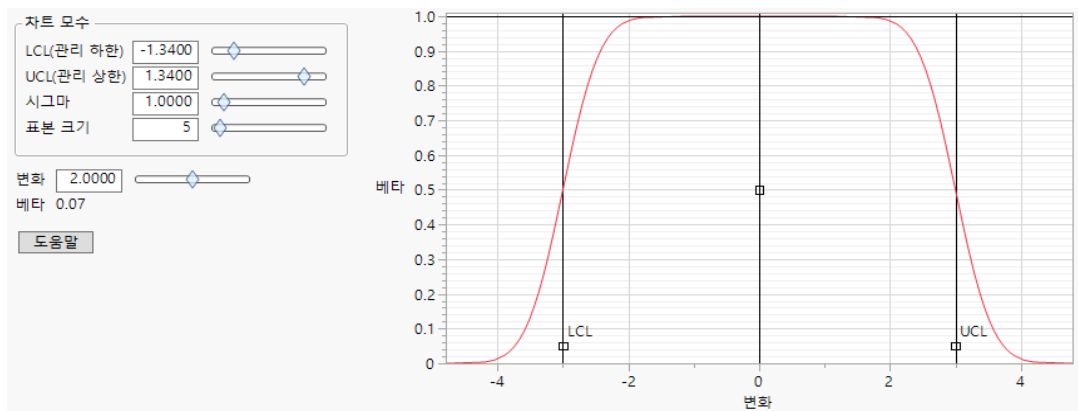
그림 18.1 OC 곡선 예
