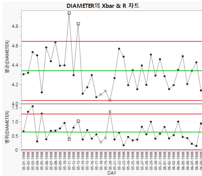
그림 3.17 Diameter( 지름 ) 에 대한 관리도
