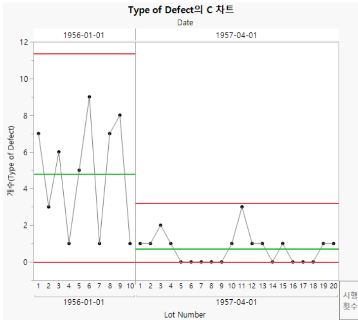
그림 3.28 단계가 있는 Type of Defect( 결함 유형 ) 의 C 차트
