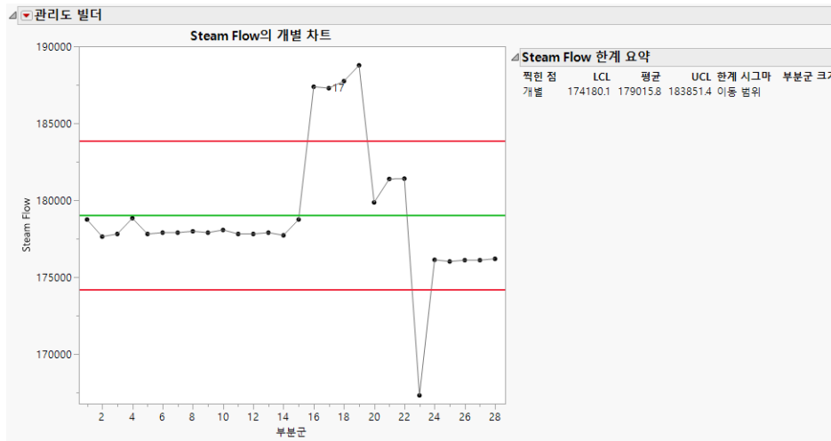
그림 13.4 Steam Flow에 대한 개별 차트
