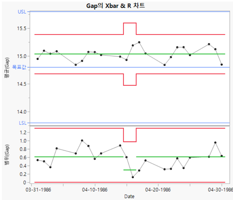
그림 9.21 Gap 에 대한 Xbar-R 관리도
