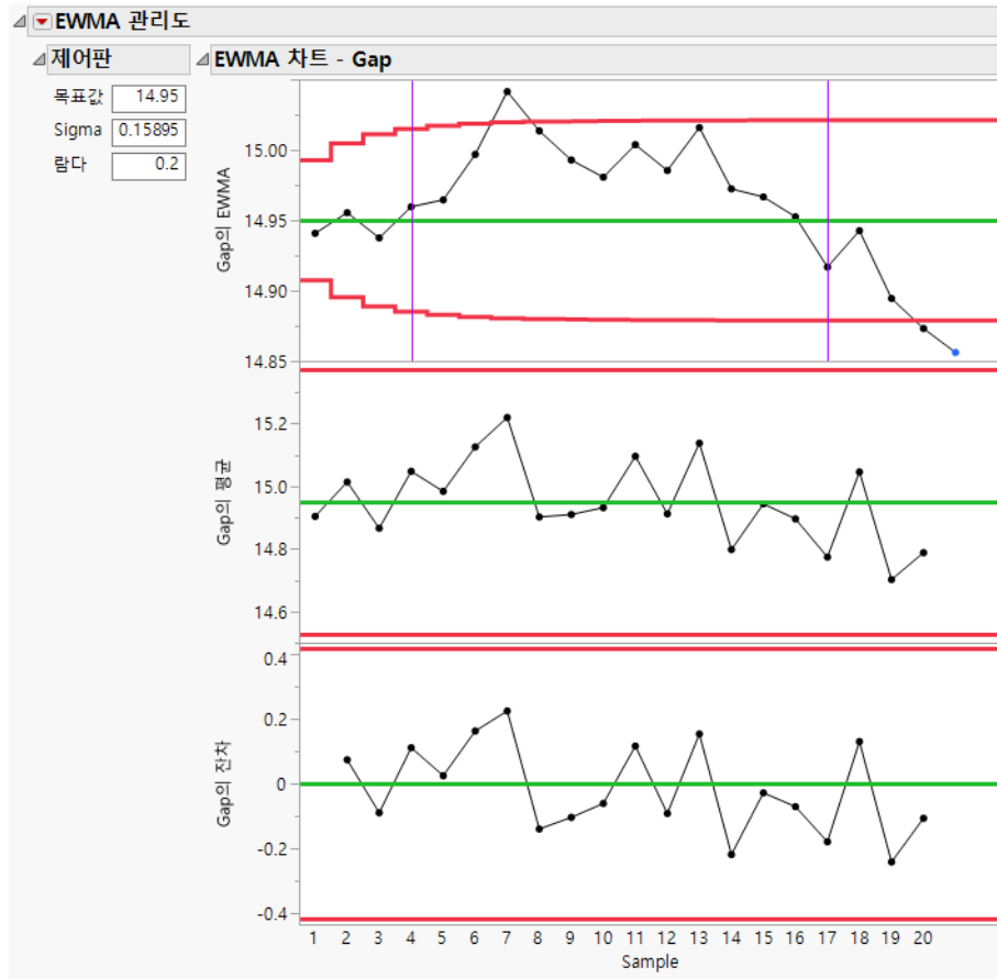
그림 11.2 EWMA 관리도
