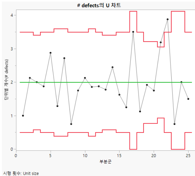
그림 3.30 # defects( 결함 수 ) 의 U 차트
