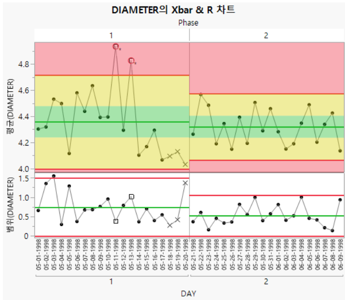
그림 3.18 각 Phase( 단계 ) 에 대한 관리도
