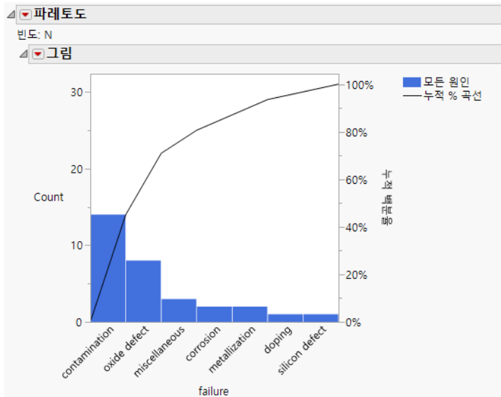
그림 15.6 파레토도 예제
