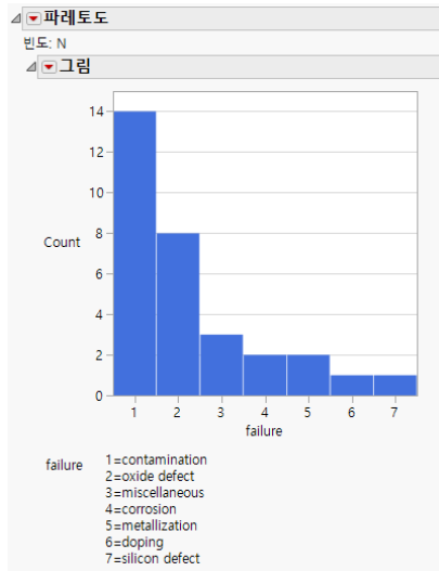
그림 15.3 표시 옵션이 있는 파레토도
