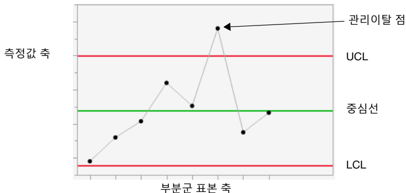
그림 14.7 관리도의 예
