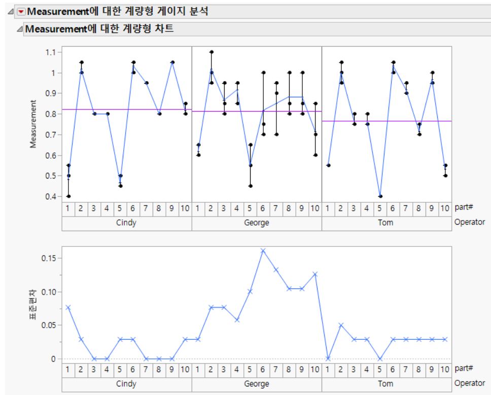
그림 6.1 계량형 차트의 예
