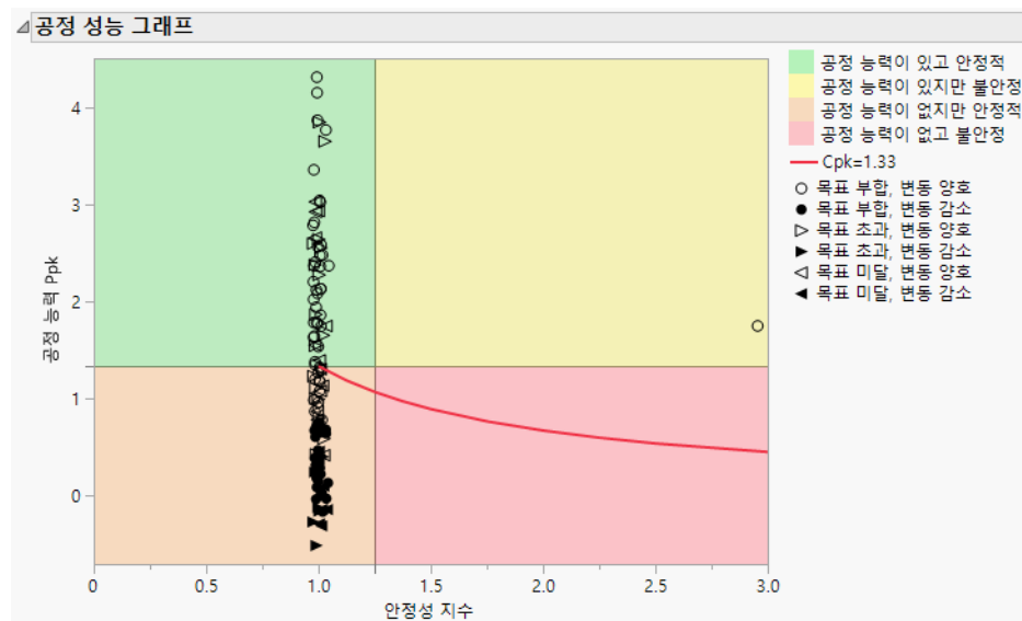
그림 8.1 공정 성능 그래프의 예
