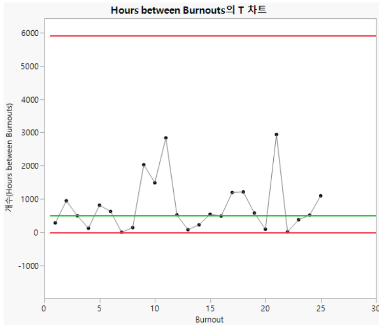
그림 3.33 Hours Between Burnouts( 연소 사이 시간 ) 의 T 차트
