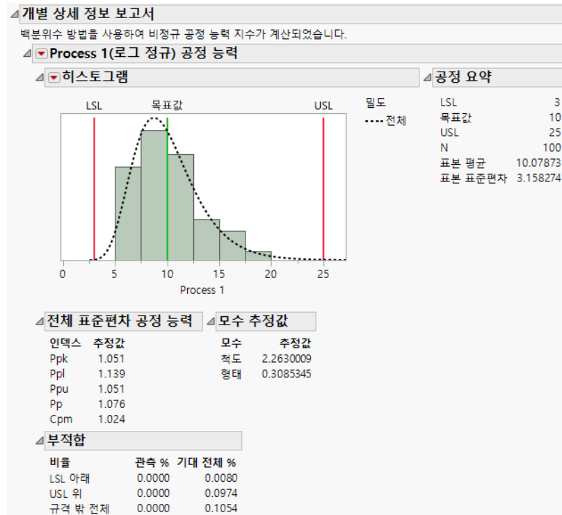
그림 9.15 Process 1의 개별 상세 정보 보고서
