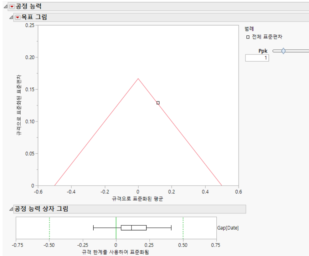
그림 9.24 Gap 에 대한 목표 그림 및 상자 그림
