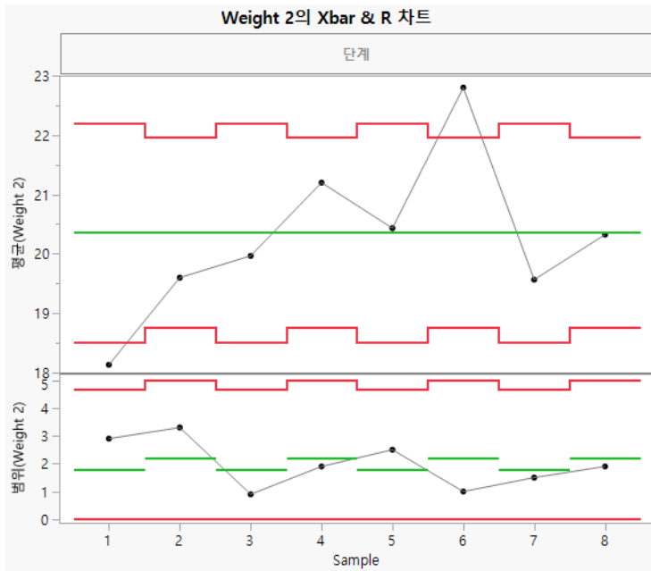
그림 3.20 다양한 부분군 크기에 대한 Xbar-R 차트
