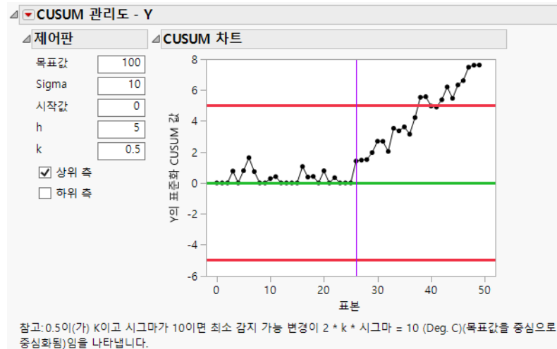
그림 10.3 단측 CUSUM 관리도 보고서
