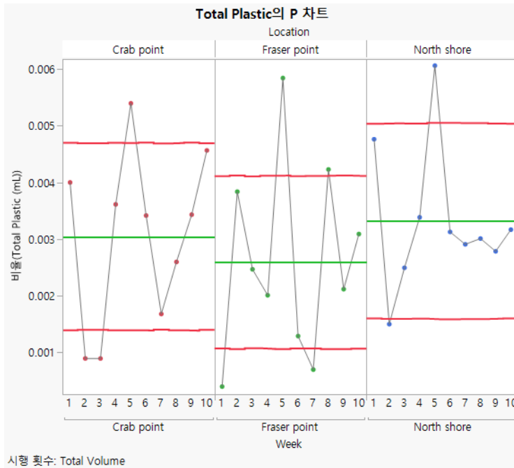
그림 3.24 Water Plastics 에 대한 표준 P 차트
