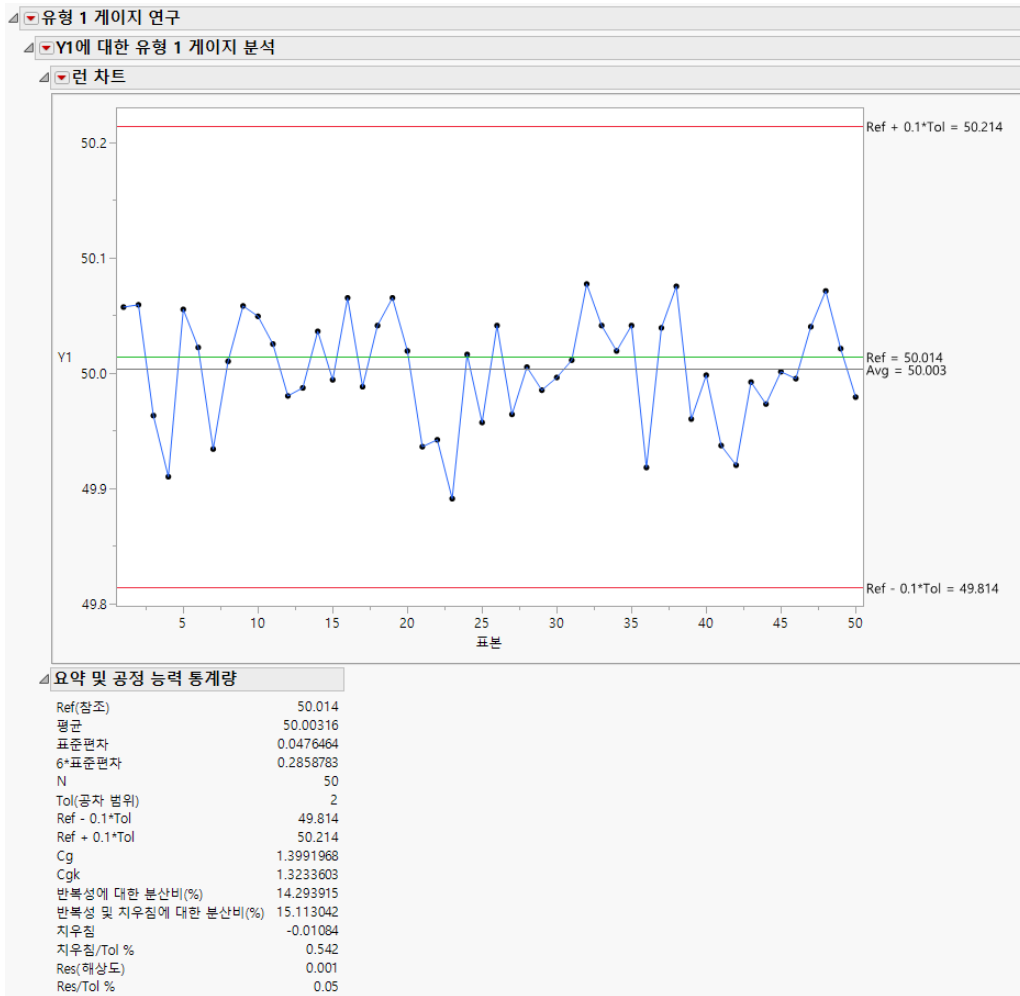
그림 5.3 Y1 에 대한 유형 1 게이지 분석 보고서
