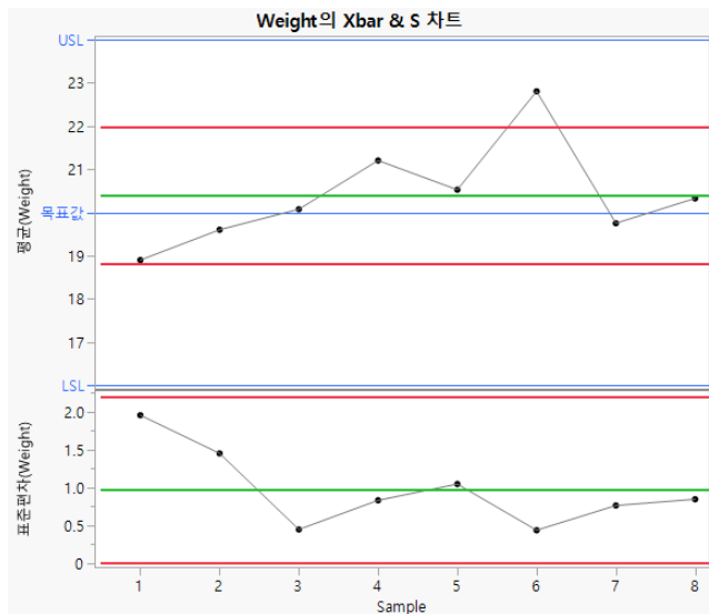
그림 9.26 Weight의 Xbar-S 차트
