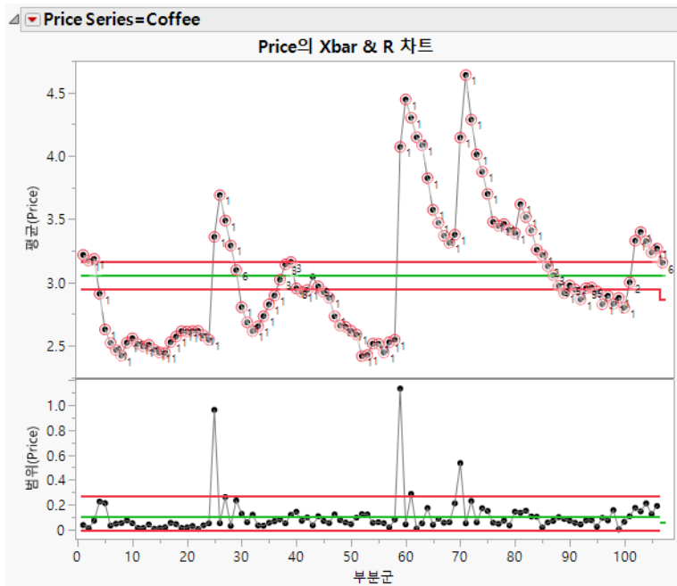
그림 8.8 Coffee에 대한 관리도
