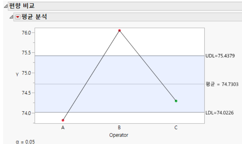
그림 4.11 치우침 비교
