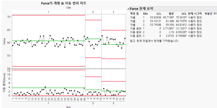
그림 3.14 과거 한계를 기반으로 한 새 데이터의 관리도
