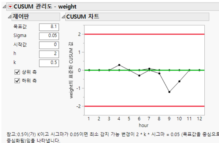
그림 10.7 부분군이 있는 CUSUM 관리도
