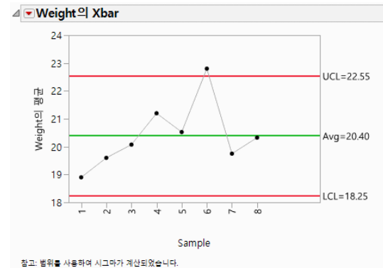
그림 14.5 K 시그마 = 3( 왼쪽 ) 및 K 시그마 = 4( 오른쪽 ) 관리 한계
