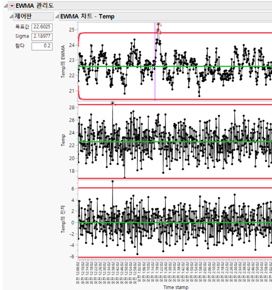
그림 11.6 한계를 벗어난 점이 강조 표시된 EWMA 차트
