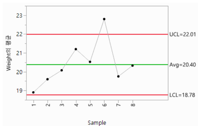
그림 14.1 관리도 예제
