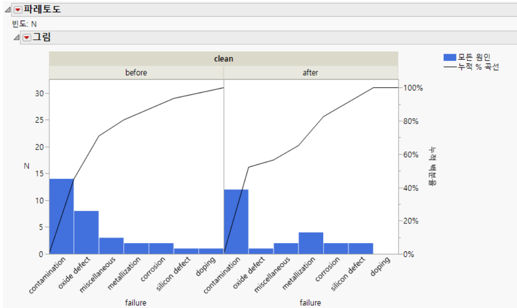
그림 15.14 셀이 재정렬된 일원 비교 파레토도
