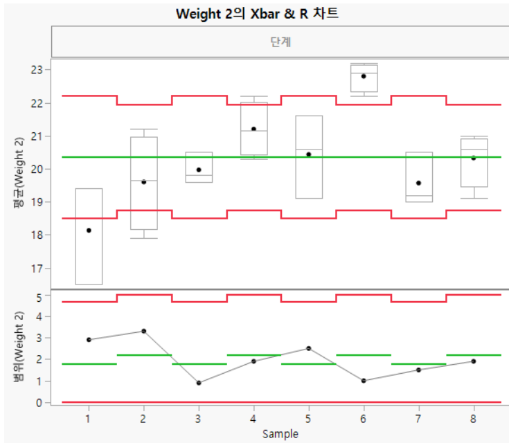
그림 3.21 상자 그림을 사용한 Xbar-R 차트
