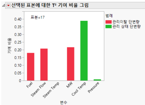
그림 13.3 표본 17에 대한 기여 비율 그림
