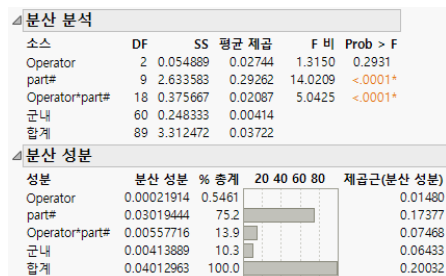
그림 6.5 분산 성분 보고서의 예
