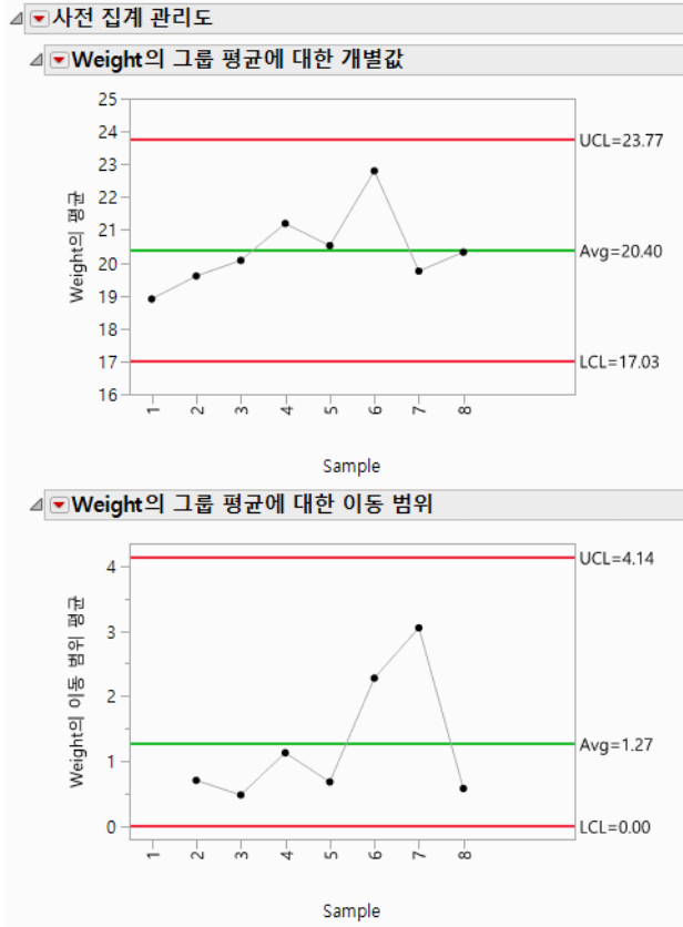
그림 14.17 사전 집계 데이터로 차트 생성의 예
