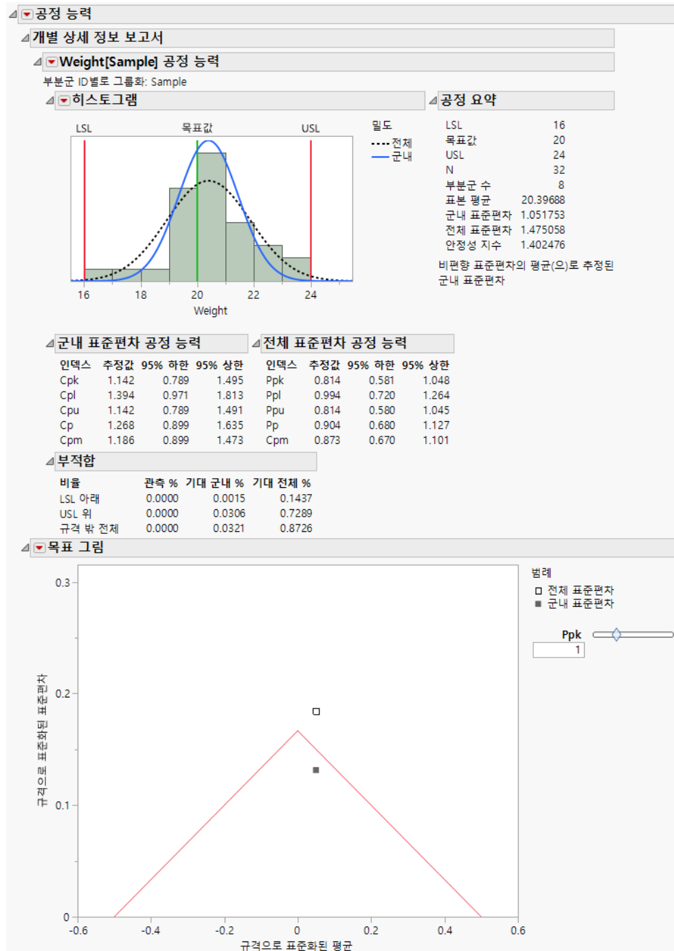
그림 9.25 Coating.jmp 데이터에 대한 공정 능력 보고서
