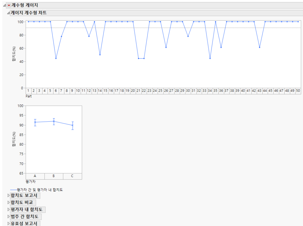
그림 7.6 게이지 계수형 차트
