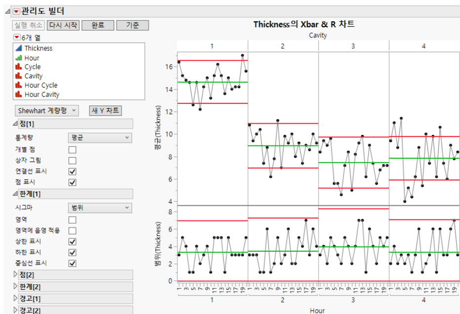
그림 3.1 관리도 빌더의 예
