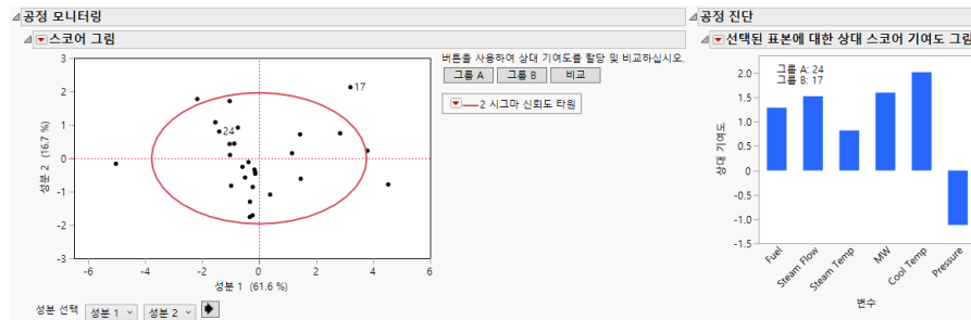
그림 13.8 24 행을 기준으로 17 행에 대한 상대 기여도 그림이 있는 스코어 그림
