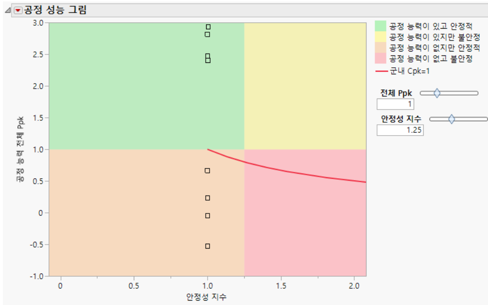
그림 9.18 공정 성능 그림
