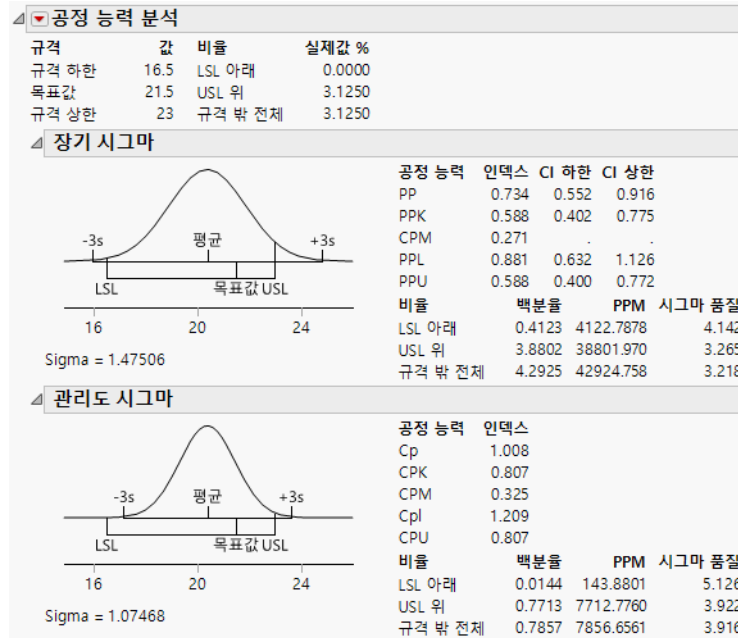
그림 14.13 Coating.jmp 에 대한 공정 능력 분석 보고서
