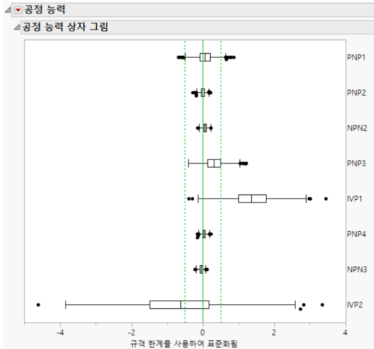
그림 9.12 공정 능력 상자 그림
