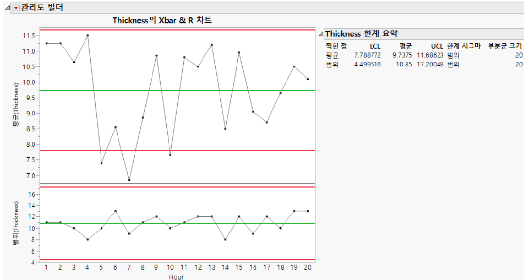
그림 3.2 Thickness( 소켓 두께 ) 에 대한 관리도
