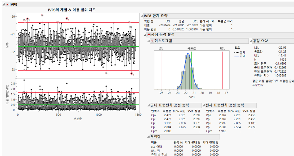
그림 8.4 IVP8에 대한 관리도 빌더 보고서
