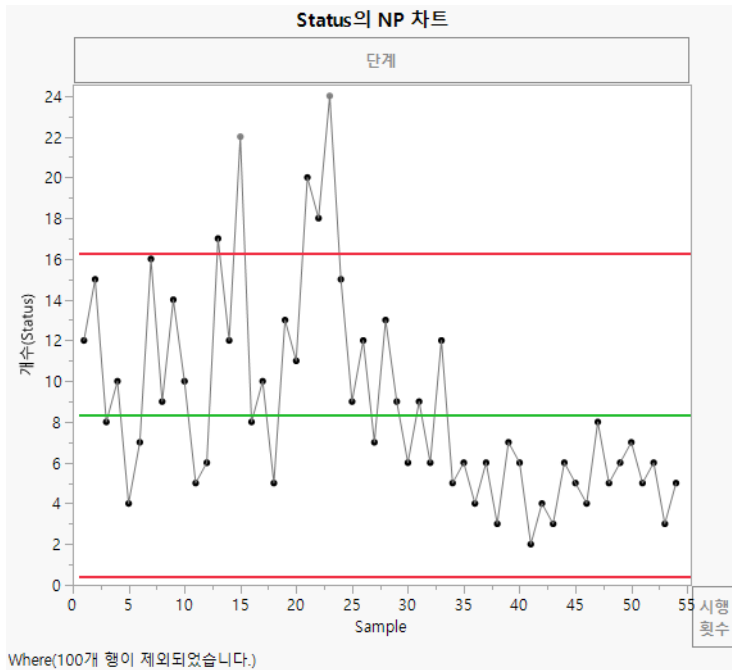
그림 3.26 Status( 부적합 상태 ) 의 NP 차트
