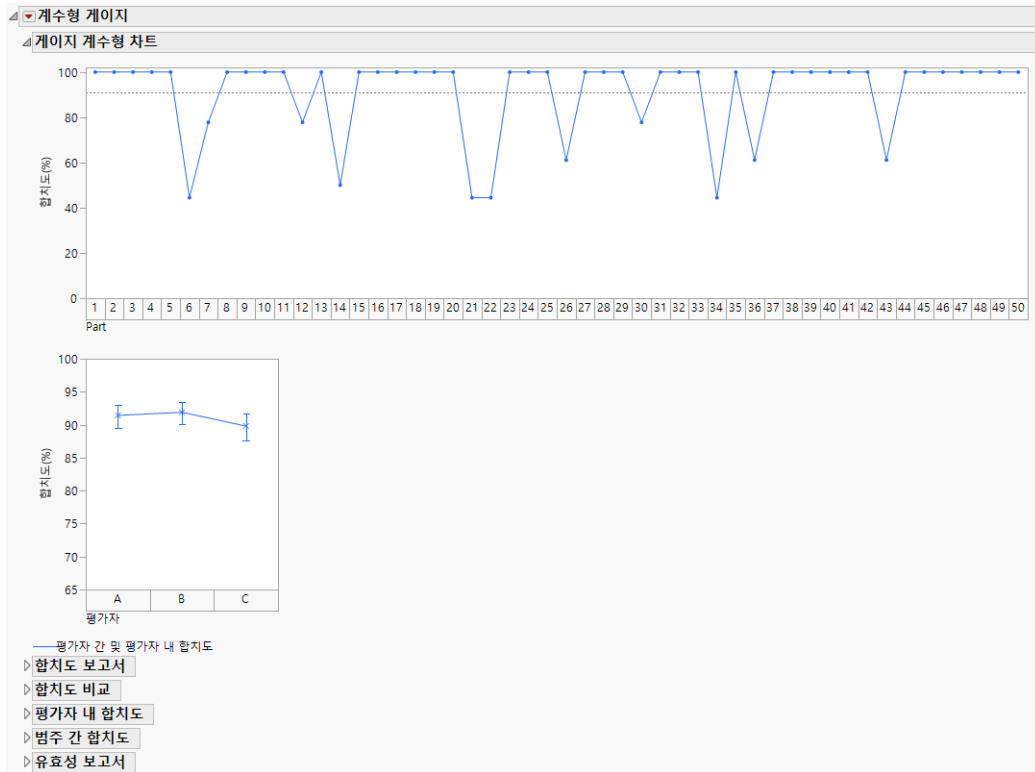
그림 7.3 계수형 차트의 예
