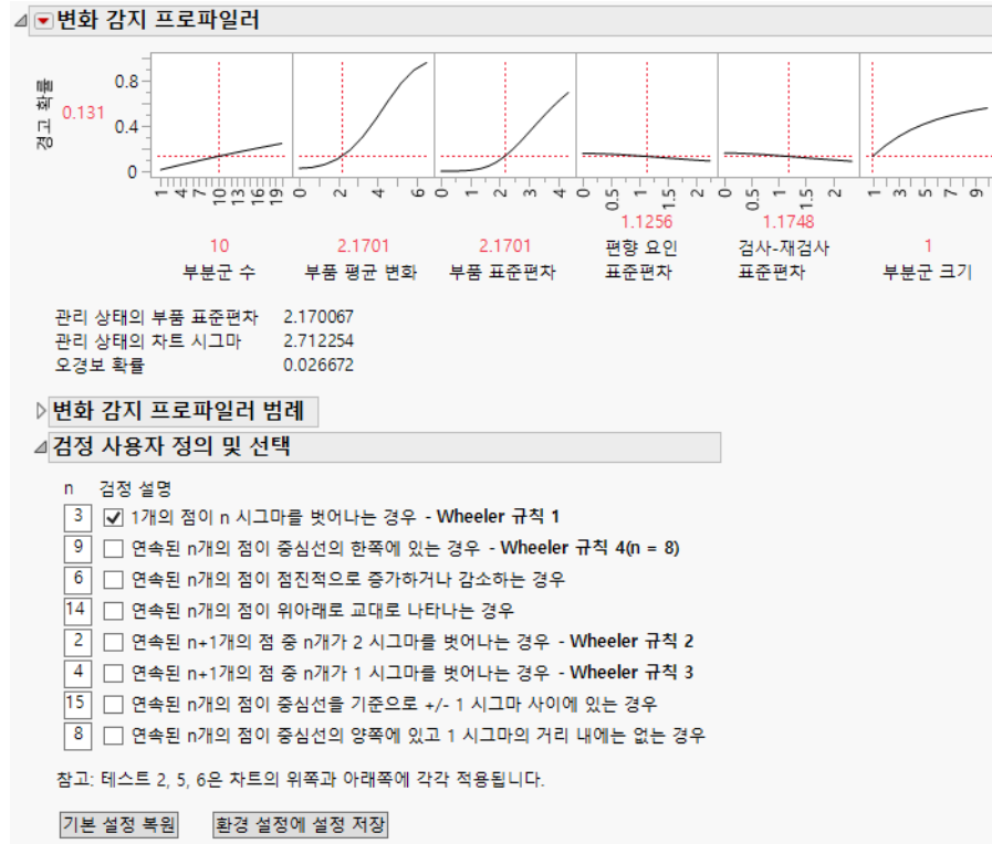
그림 4.13 변화 감지 프로파일러
