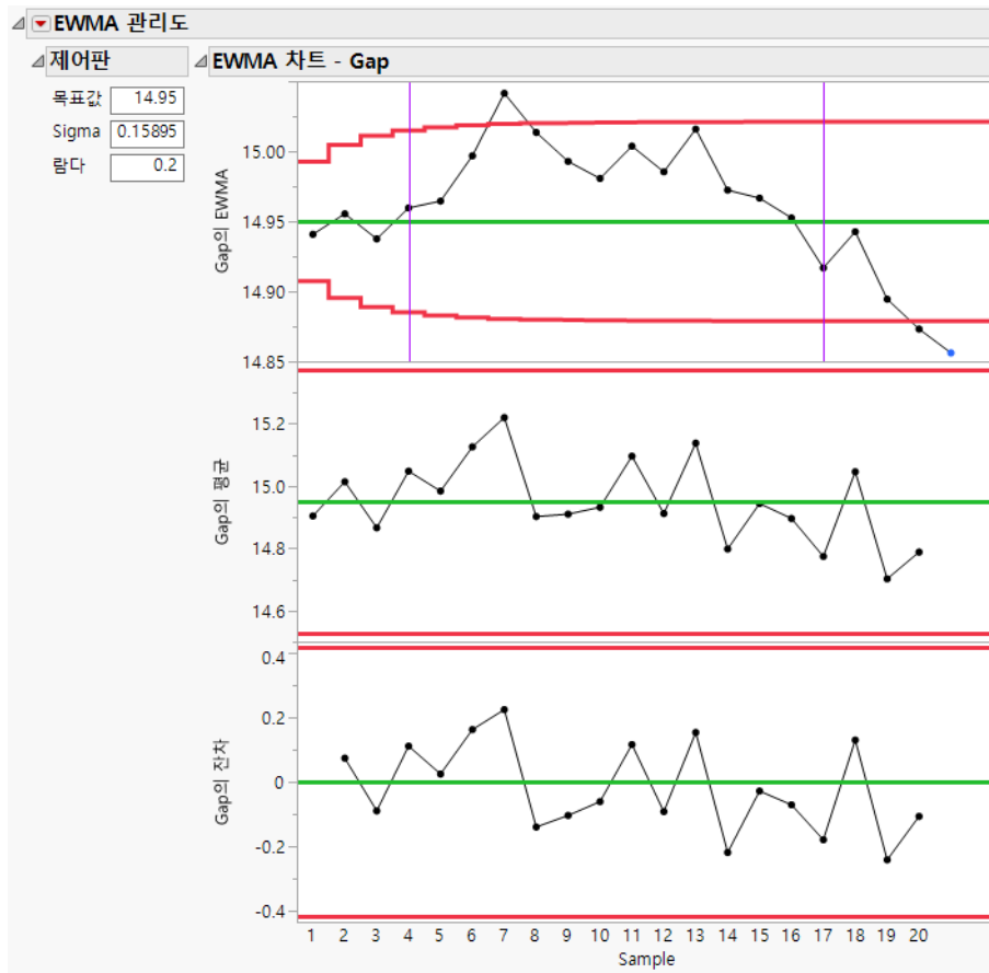
그림 11.1 EWMA 관리도 보고서
