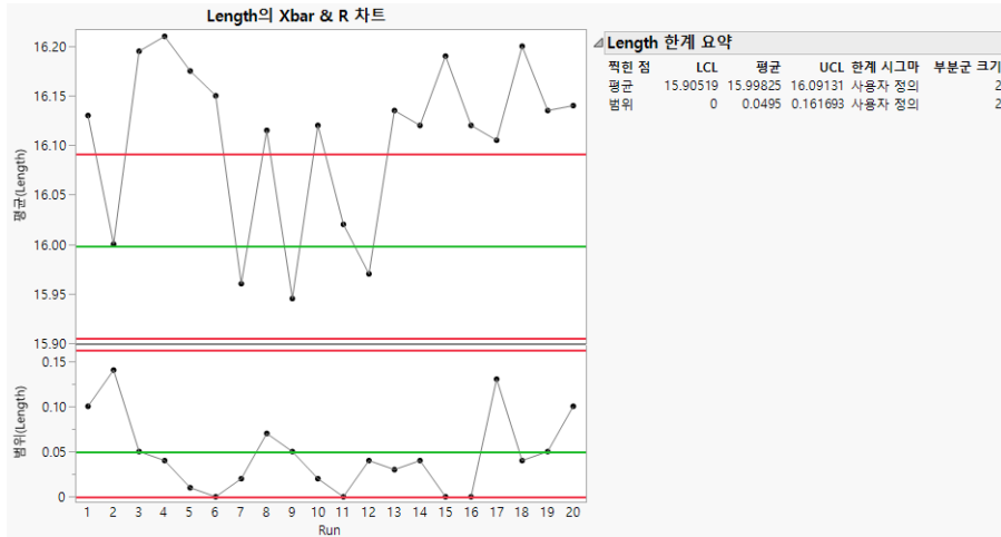
그림 3.11 과거 한계를 사용한 Length( 선 길이 ) 의 Xbar-R 차트
