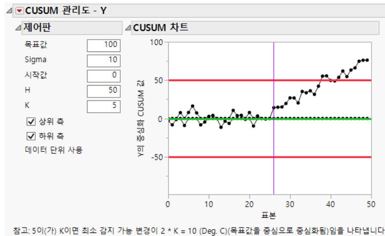
그림 10.6 CUSUM 관리도 보고서
