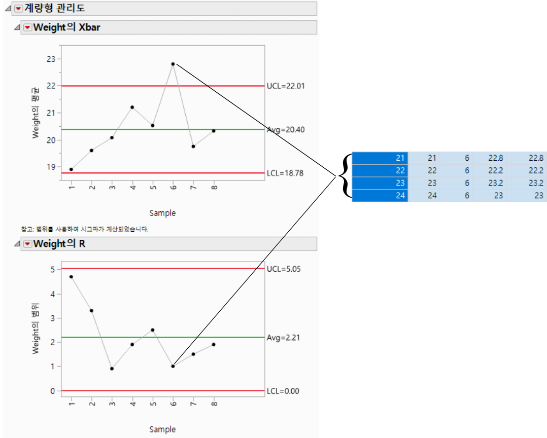
그림 14.2 Coating( 코팅 ) 데이터에 대한 계량형 차트
