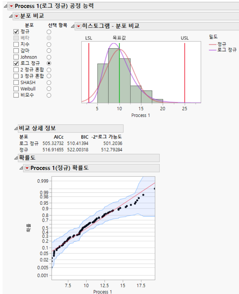
그림 9.16 정규 분포의 확률도를 사용한 분포 비교
