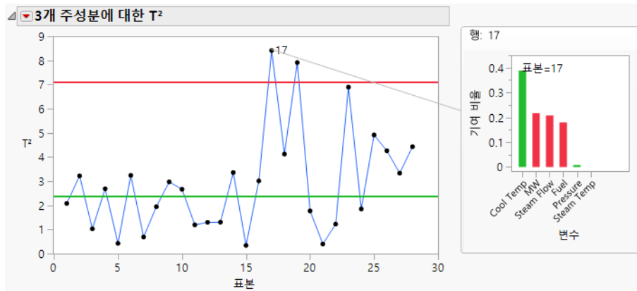
그림 13.1 모형 기반 다변량 관리도
