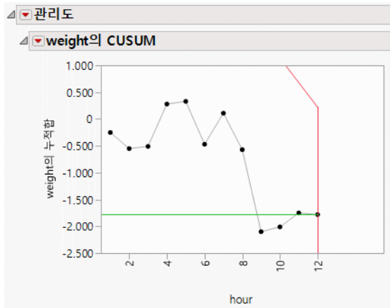
그림 14.19 Oil1 Cusum.jmp 데이터에 대한 양측 CUSUM 차트
