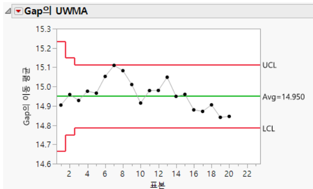
그림 14.21 Clips1 데이터에 대한 UWMA 차트
