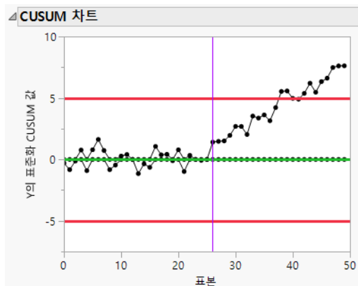
그림 10.1 CUSUM 관리도
