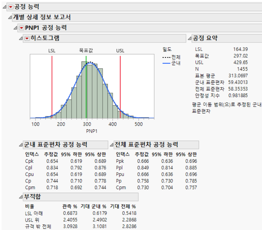
그림 9.14 개별 상세 정보 보고서
