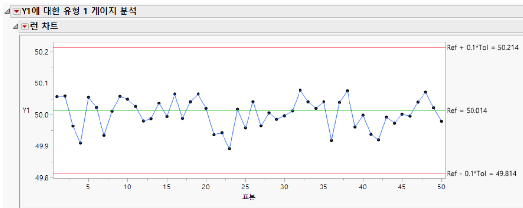
그림 5.1 유형 1 게이지 분석의 예
