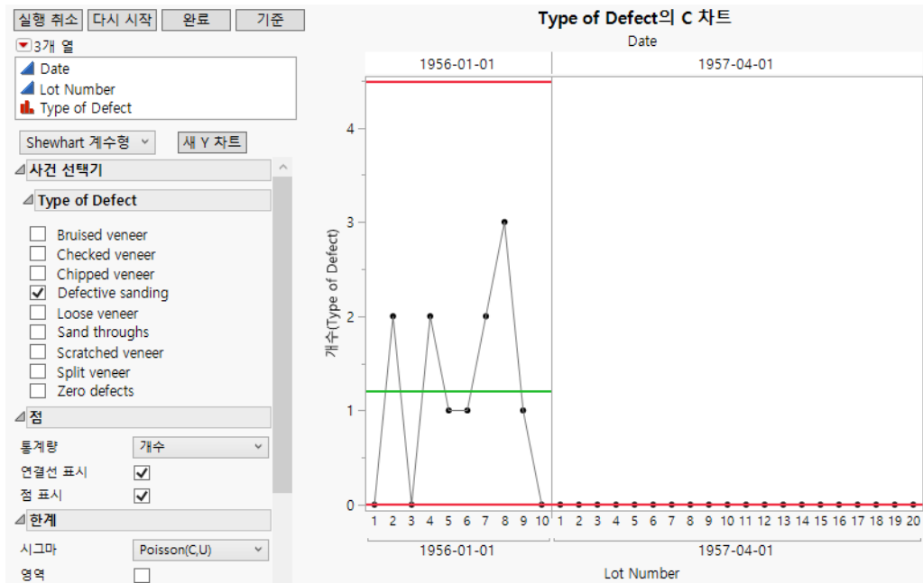
그림 3.29 Defective Sanding 결함 유형의 C 차트
