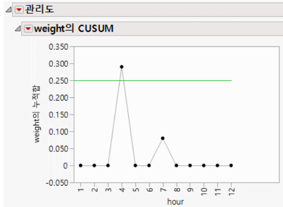
그림 14.10 단측 CUSUM 차트의 예
