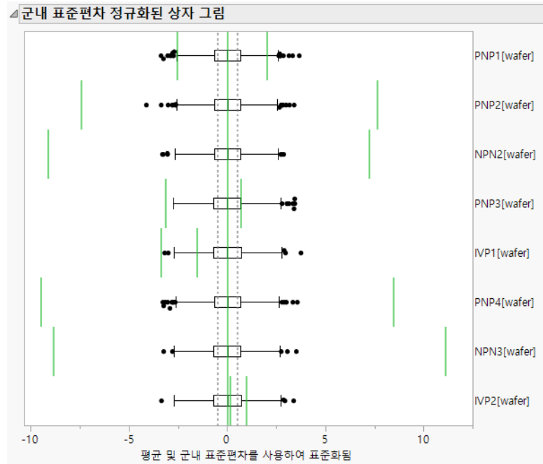
그림 9.17 군내 표준편차 정규화된 상자 그림
