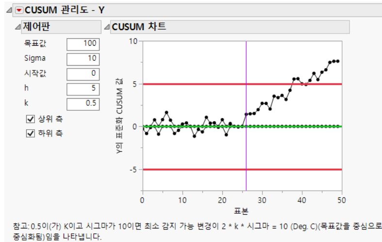
그림 10.2 CUSUM 관리도 보고서
