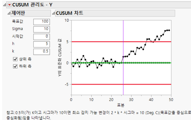
그림 10.5 CUSUM 관리도 보고서
