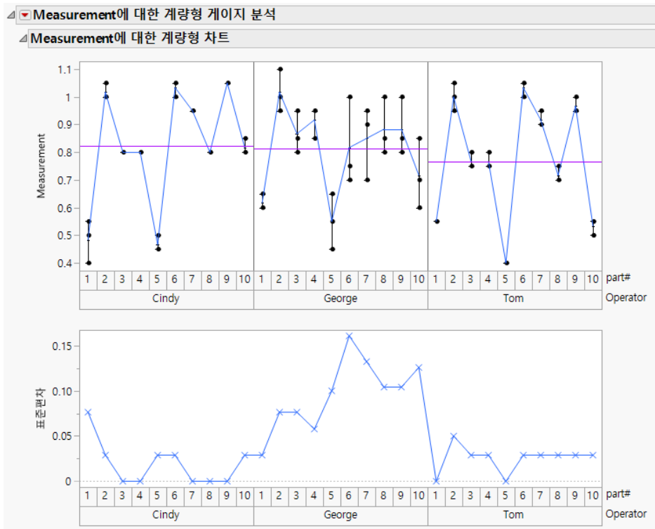
그림 6.2 계량형 차트의 예
