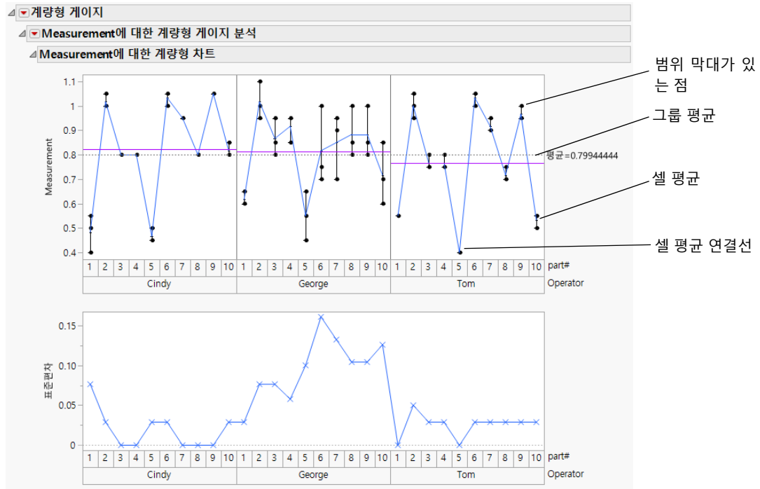
그림 6.4 계량형 게이지 보고서
