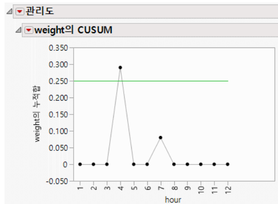
그림 14.20 Oil1 Cusum.jmp 데이터에 대한 단측 CUSUM 차트
